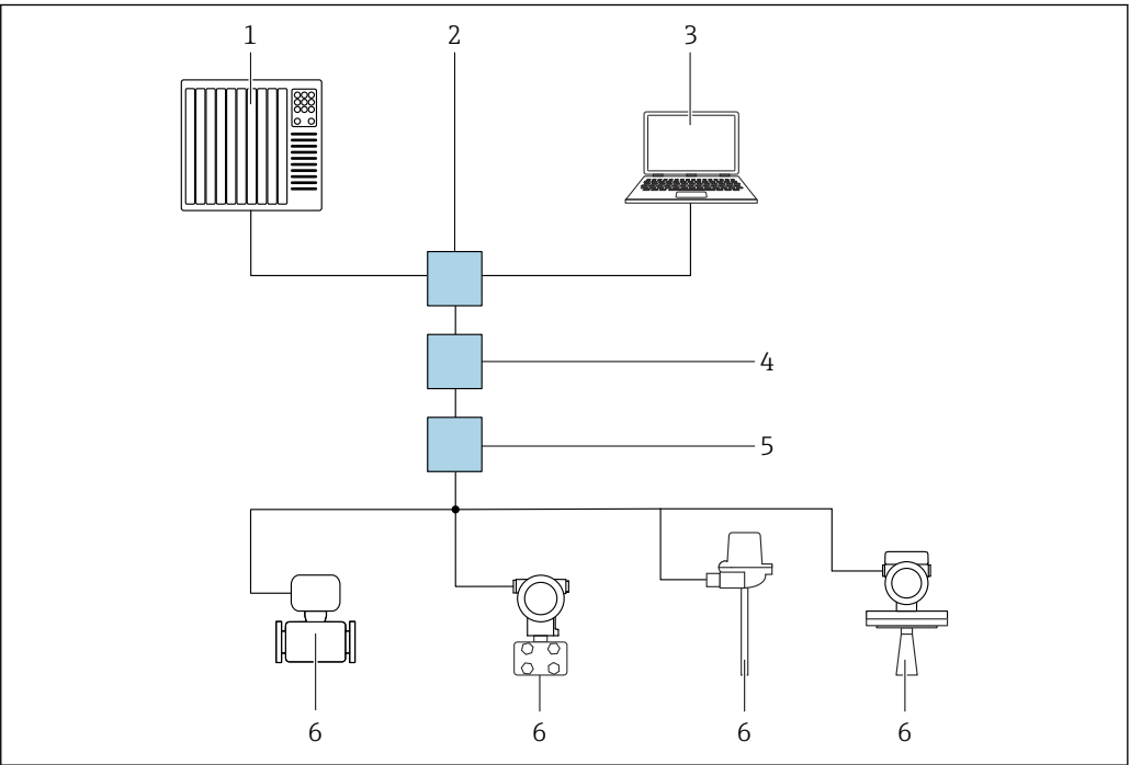
图 49 通过 PROFINET + Ethernet-APL 网络实现远程操作：星形拓扑结构
