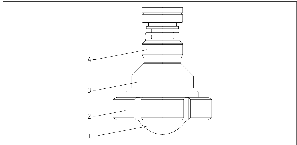
图 44 涂层天线（齐平安装，80 mm (3 in)口径）的材质；带 DIN11851 开槽螺母。测量单位 mm (in)
