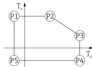
图 30 316L 外壳，卫生型；过程温度范围：-40 ... +200 °C (-40 ... +392 °F)
