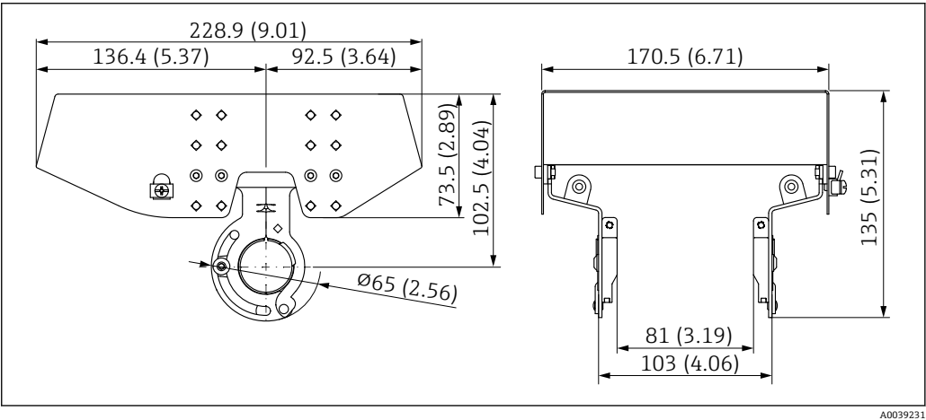
50 外形尺寸示意图。测量单位 mm (in)
