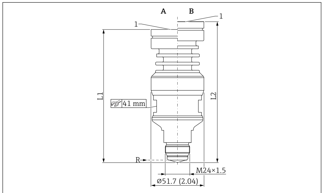
■ 36 PEEK 一体式天线（20 mm 口径）的外形尺寸示意图；M24×1.5 过程连接。测量单位 mm (in)
