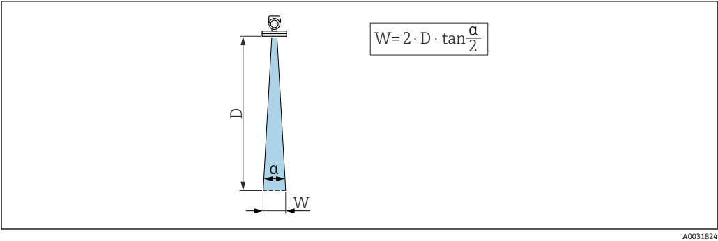
图 10 波束角 \alpha 、距离 D 和波束宽度 W 的相互关系
