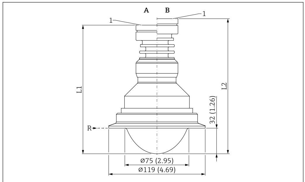
41 PTFE 涂层天线（齐平安装，80 mm (3 in) 口径）的外形尺寸示意图；带 ISO2852 Tri-Clamp DN101.6 (4") 卡箍。测量单位 mm (in)
