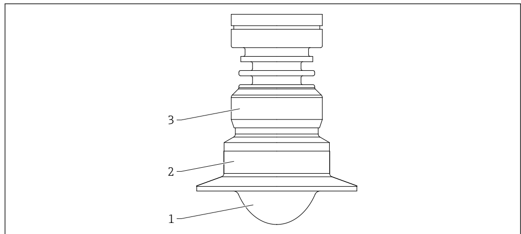
图 45 PTFE 涂层天线（齐平安装，50 mm (2 in)口径）的材质；带 ISO2852 Tri-Clamp 卡箍。测量单位 mm (in)
