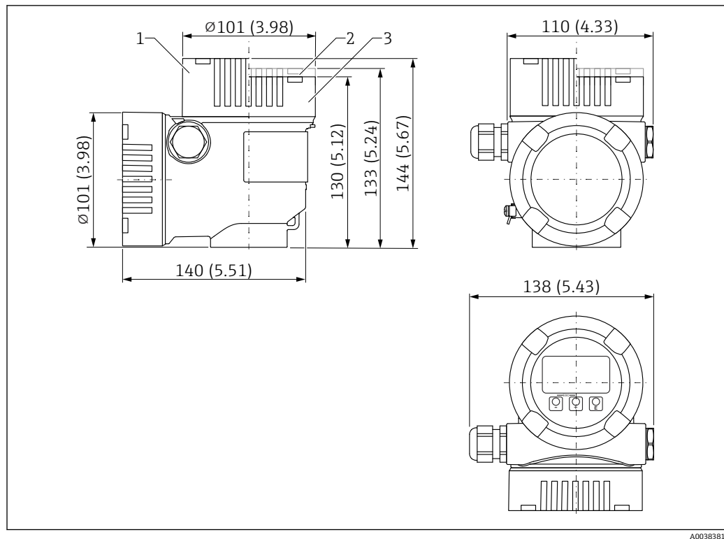
图 35 双腔室外壳 (L 型) 的外形尺寸示意图。测量单位 mm (in)
