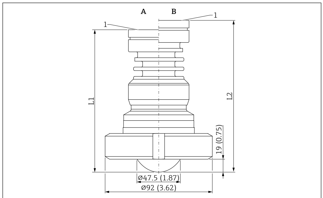
■ 37 PTFE 涂层天线（齐平安装，50 mm (2 in) 口径）的外形尺寸示意图；带 DIN11851 开槽螺母。测量单位 mm (in)
