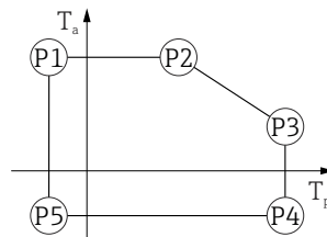
图 15 塑料外壳; 过程温度范围: -40 ... +150 °C (-40 ... +302 °F)
