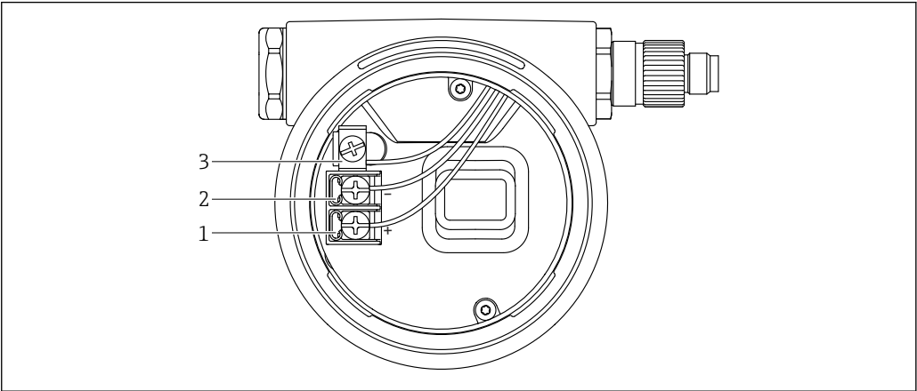
4 接线腔中的接线端子和接地端
