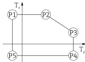
图 27 316L 外壳, 卫生型; 过程温度范围: -20 \dots +150 \text{ }^{\circ}\text{C} ( -4 \dots +302 \text{ }^{\circ}\text{F} )
