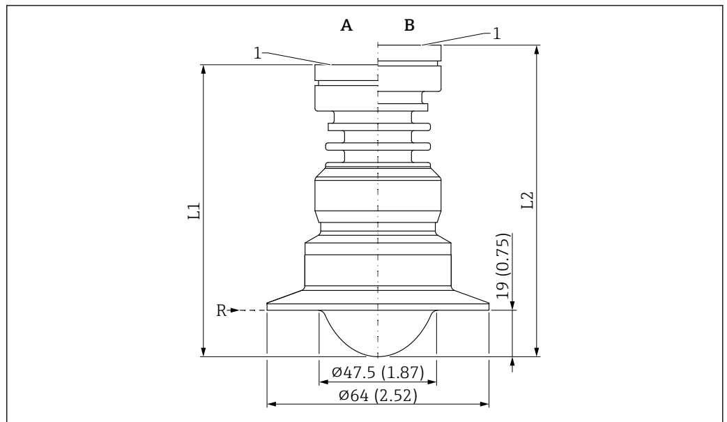
39 PTFE 涂层天线（齐平安装，50 mm (2 in)口径）的外形尺寸示意图；带 ISO2852 Tri-Clamp DN51 (2")卡箍。测量单位 mm (in)
