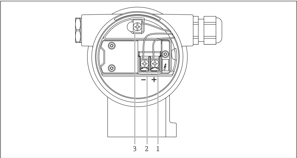
5 接线腔中的接线端子和接地端
