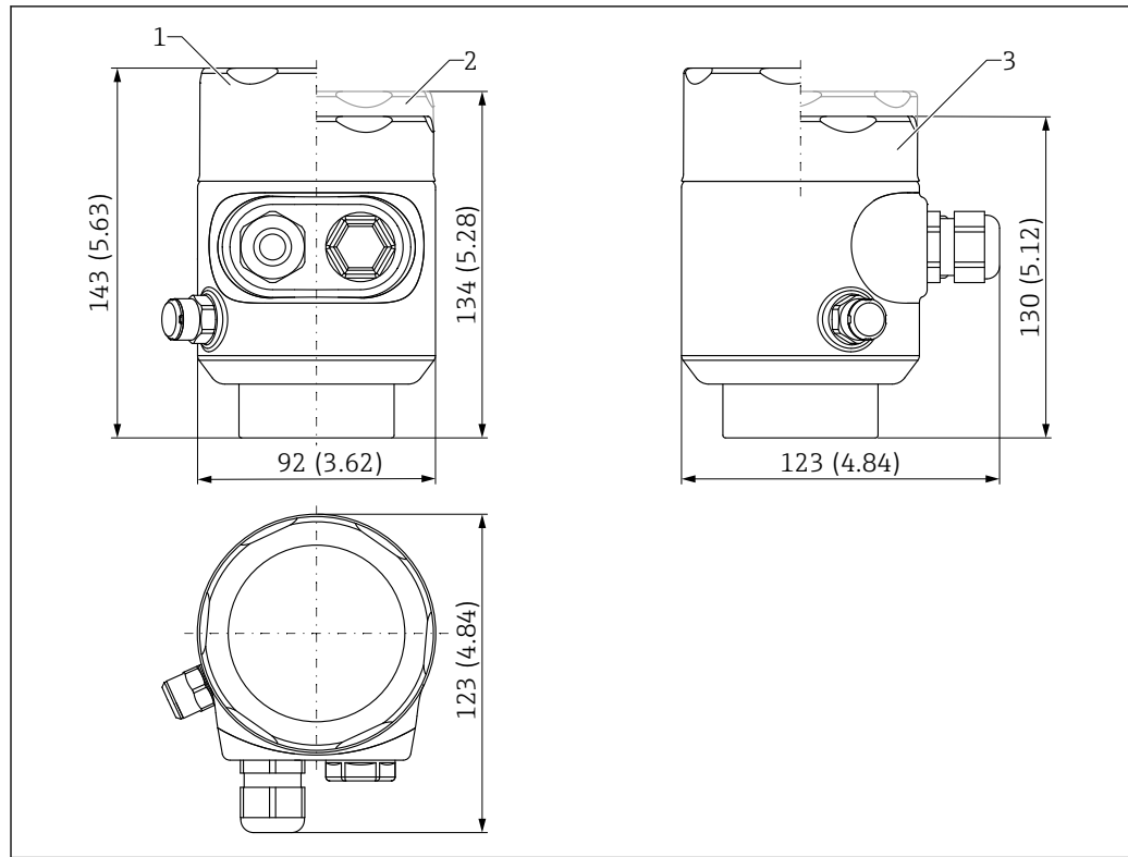
图 33 316L 单腔室外壳（卫生型）的外形尺寸示意图。测量单位 mm (in)
