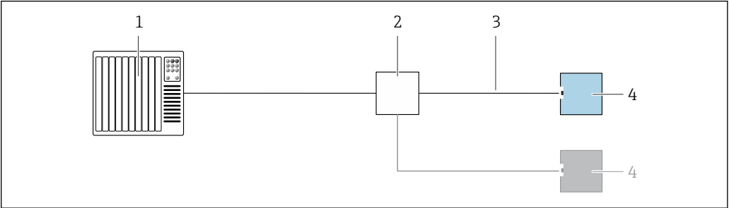
图 8 接线示例：具有 Ethernet-APL 功能的 PROFINET
