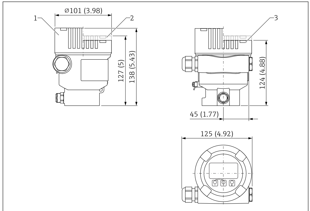
图 32 单腔室铝外壳的外形尺寸示意图。测量单位 mm (in)
