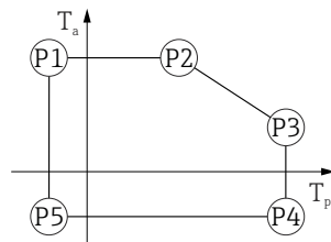
图 21 铝外壳, 带涂层; 过程温度范围: -40 \dots +150 \text{ }^{\circ}\text{C} ( -40 \dots +302 \text{ }^{\circ}\text{F} )
