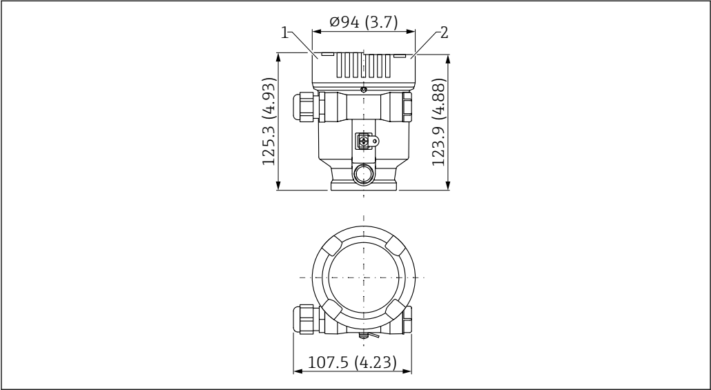
图 31 单腔室塑料 (PBT) 外壳的外形尺寸示意图。测量单位 mm (in)
