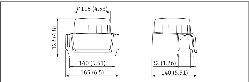
51 外形尺寸示意图。测量单位 mm (in)
