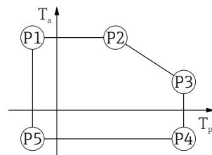
图 29 316L 外壳，卫生型；过程温度范围：-40 ... +150 °C (-40 ... +302 °F)
