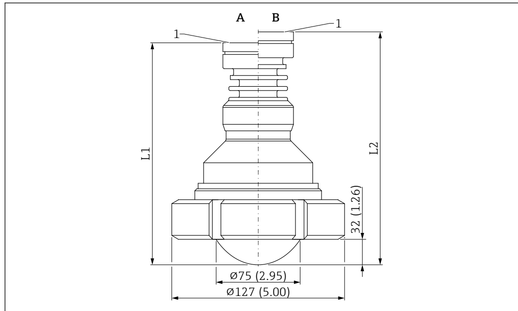
图 38 PTFE 涂层天线（齐平安装，80 mm (3 in)口径）的外形尺寸示意图；带 DIN11851 开槽螺母。测量单位 mm (in)
