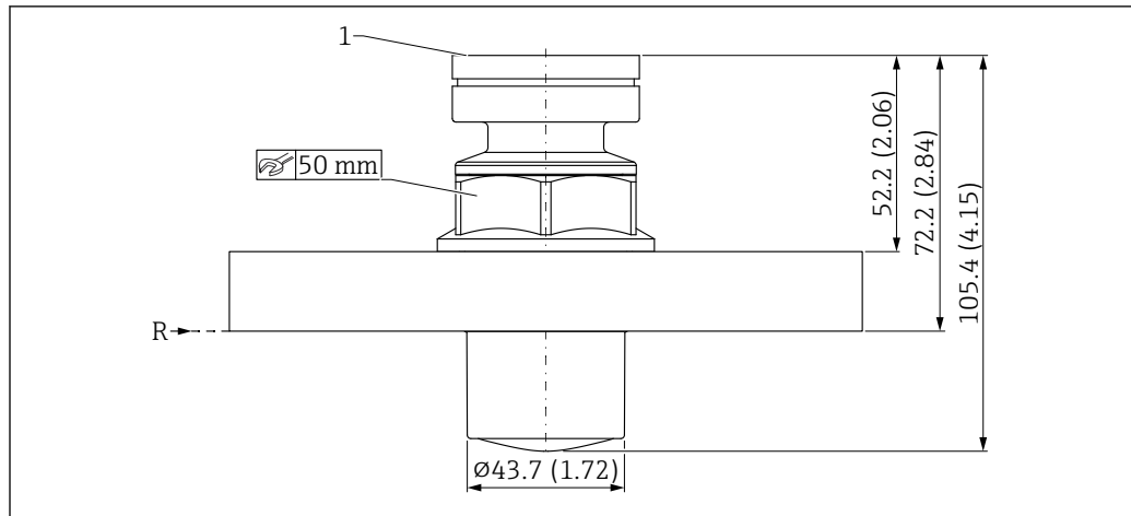
26 Medidas de la antena encapsulada, PVDF, 40 mm (1,5 in), conexión a proceso: brida UNI. Unidad de medida mm (in)
