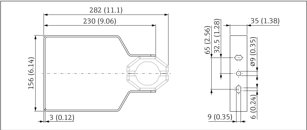
43 Dimensiones del soporte de montaje. Unidad de medida mm (in)
