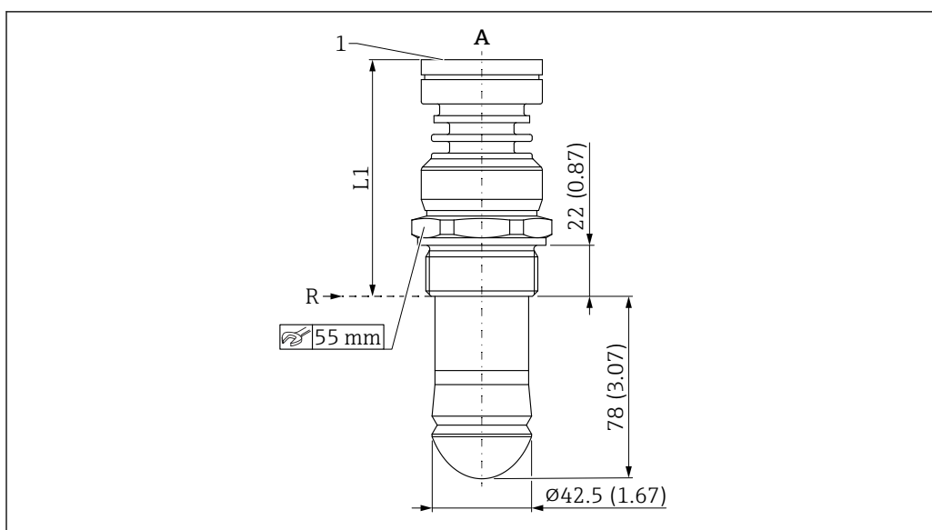
30 Medidas de la antena de goteo de 50 mm (2 in), conexión a proceso rosca. Unidad de medida mm (in)
