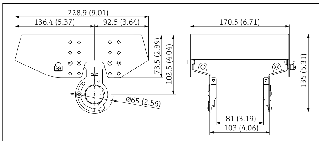
40 Medidas. Unidad de medida mm (in)
