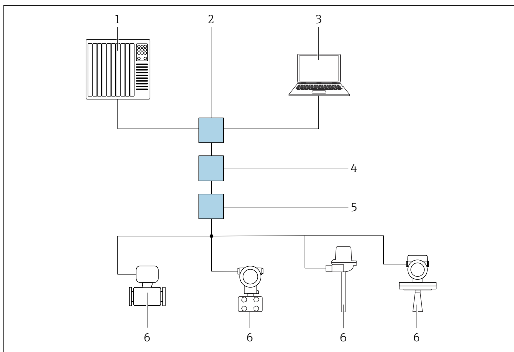
39 Opciones para la configuración a distancia a través de la red PROFINET con Ethernet-APL: topología en estrella
