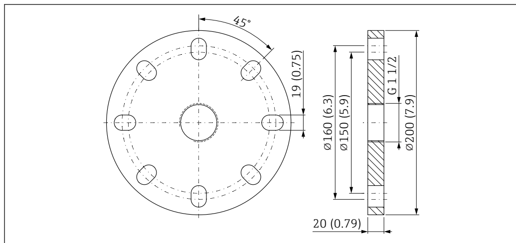
27 Medidas de la brida UNI 3" / DN 80 / 80 A. Unidad de medida mm (in)
