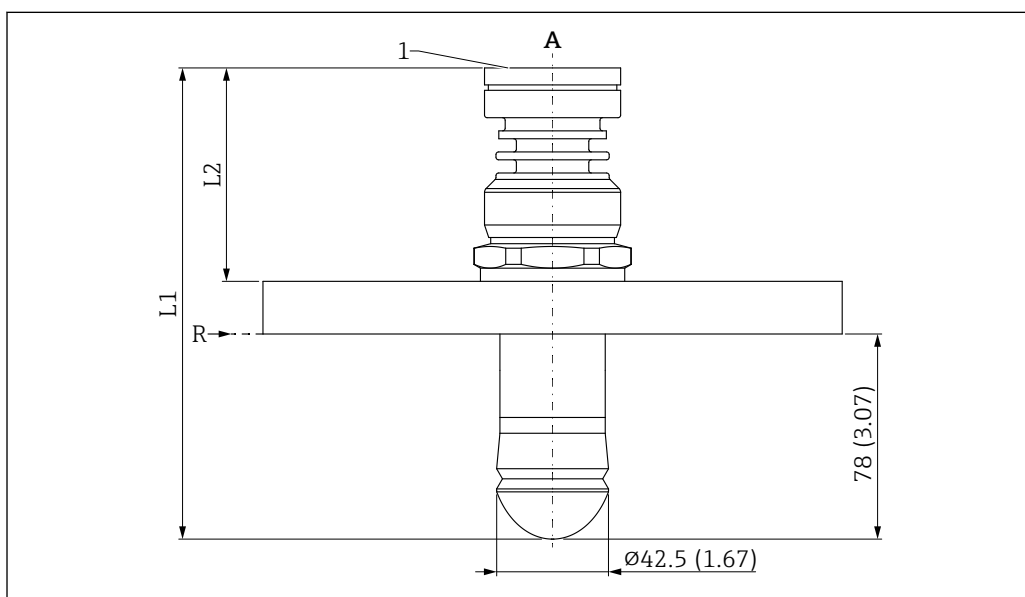
31 Medidas de la antena de goteo de 50 mm (2 in), conexión a proceso con brida UNI. Unidad de medida mm (in)
