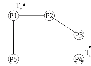
■ 19 Caja de 316L, higiene; temperatura de proceso -40 \dots +130 \text{ }^{\circ}\text{C} ( -40 \dots +266 \text{ }^{\circ}\text{F} )
