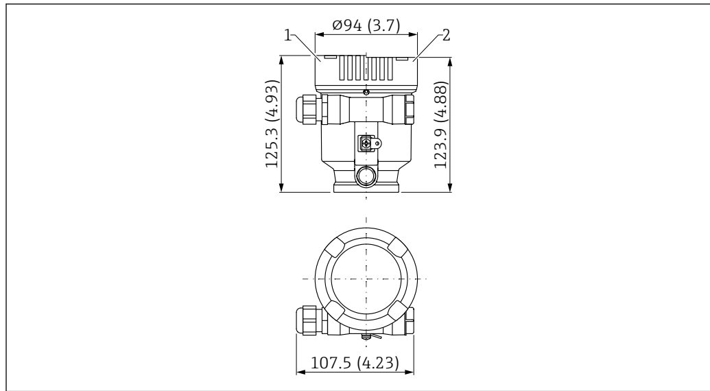
20 Medidas de la caja de compartimento único, plástico (PBT). Unidad de medida mm (in)
