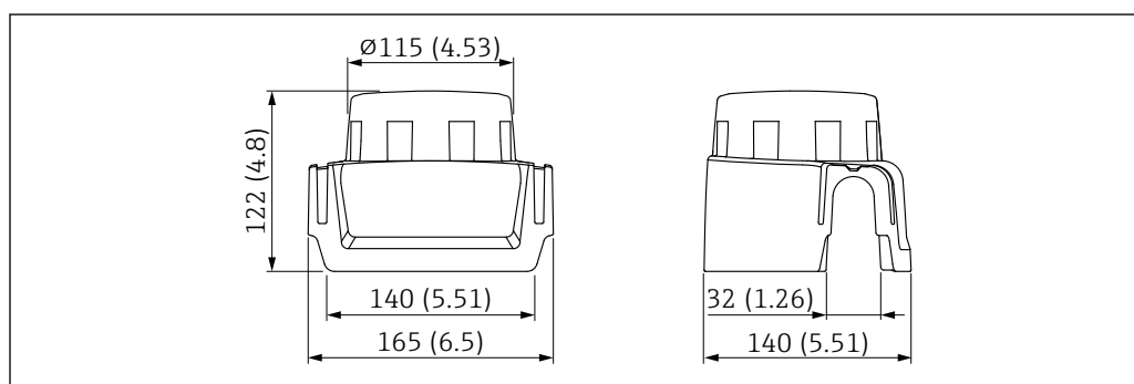
41 Medidas. Unidad de medida mm (in)
