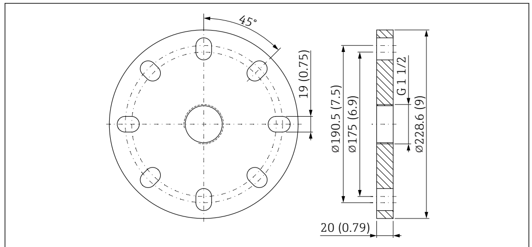
33 Medidas de la brida UNI de 4"/DN100/100A. Unidad de medida mm (in)
