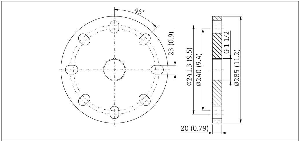
34 Medidas de la brida UNI de 6"/DN150/150A. Unidad de medida mm (in)
