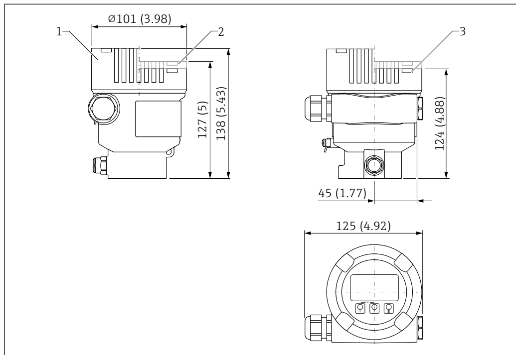
21 Medidas de la caja de aluminio de compartimento único. Unidad de medida mm (in)
