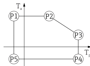
10 Caja de plástico; temperatura de proceso -40 ... +80 °C (-40 ... +176 °F)
