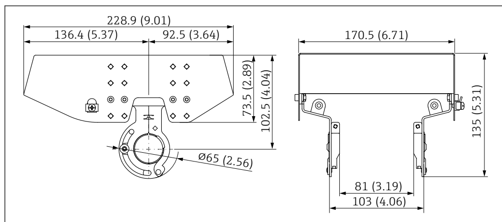
図 40 寸法。測定単位 mm (in)
