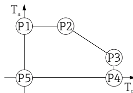
図 11 プラスチックハウジング；プロセス温度 0～+80 °C (+32～+176 °F)、CSA C/US 認定取得
