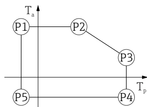
図 14 アルミニウムハウジング ; コーティング ; プロセス温度 -40\sim+80\text{ }^{\circ}\text{C} ( -40\sim+176\text{ }^{\circ}\text{F} )
