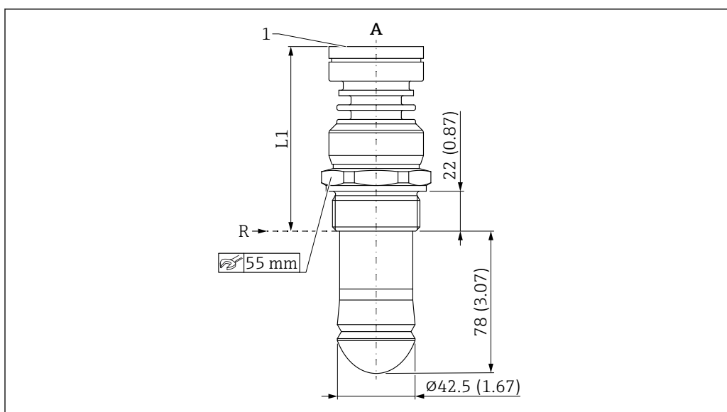
図 30 ドリップオフアンテナ 50 mm (2 in) (ネジ込みプロセス接続) の寸法。測定単位 mm (in)
