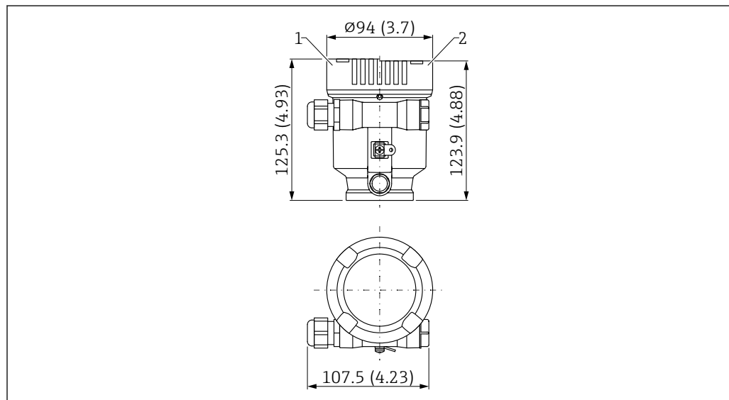
図 20 シングル端子箱部、プラスチック (PBT) の寸法。測定単位 mm (in)
