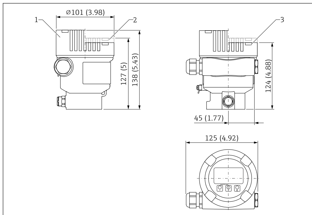
図 21 アルミニウムシングル端子箱部の寸法。測定単位 mm (in)
