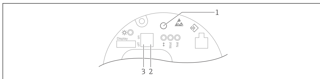
図 37 Ethernet-APL エレクトロニックインサート上の操作キーおよび DIP スイッチ
