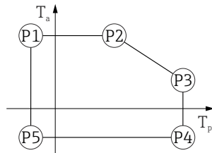
図 10 プラスチックハウジング；プロセス温度 -40～+80 °C (-40～+176 °F)
