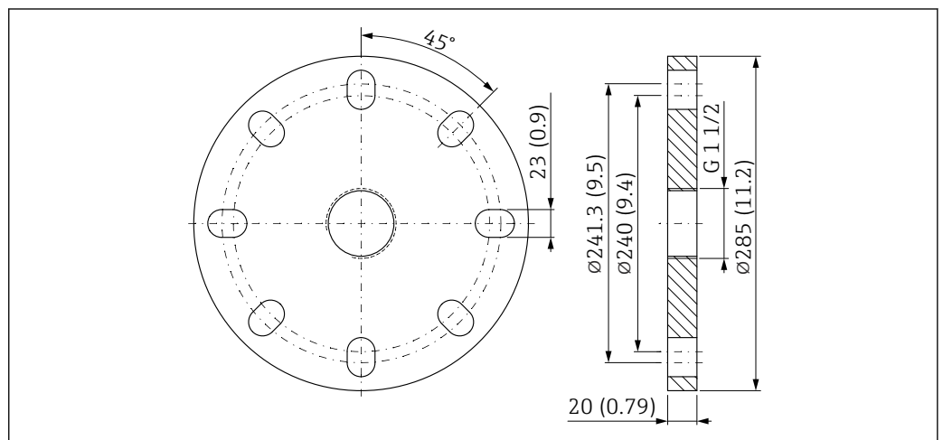
図 29 UNI フランジ 6"/DN150/150A の寸法。測定単位 mm (in)
