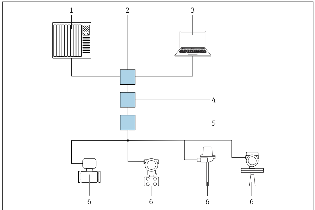
図 39 PROFINET (Ethernet-APL 対応) ネットワーク経路のリモート操作オプション：スター型トポロジ
