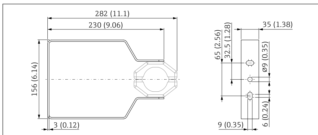
図 43 取付ブラケットの寸法。測定単位 mm (in)
