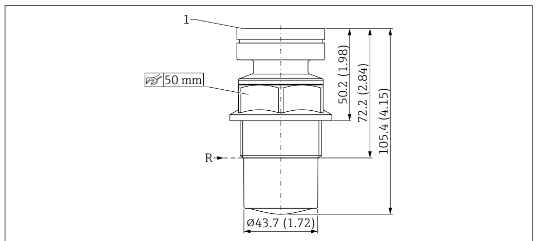
図 25 被覆アンテナ (PVDF、40 mm (1.5 in)) の寸法。測定単位 mm (in)
