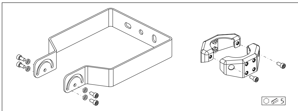
図 44 取付ブラケット（調整可能）の納入範囲
