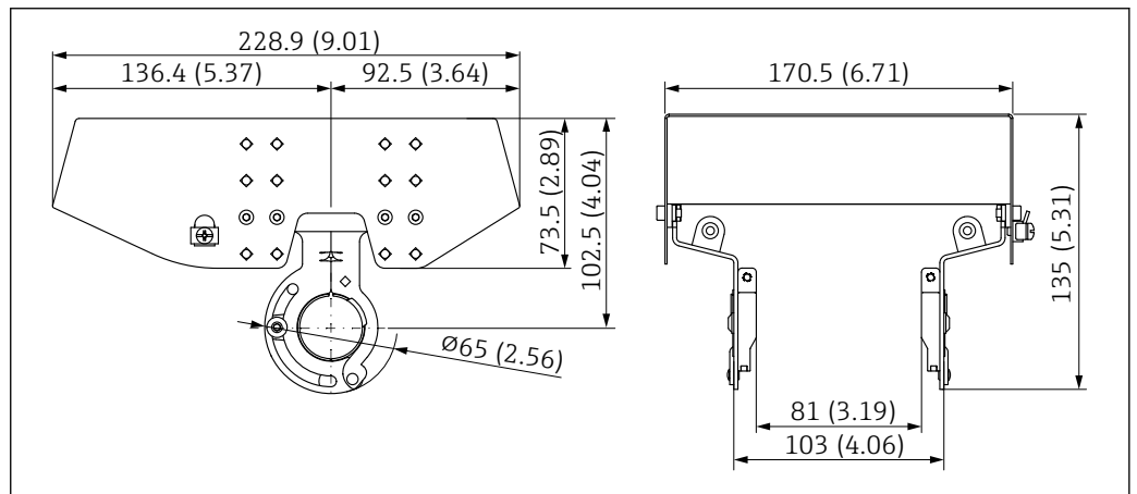
图 69 外形尺寸示意图。测量单位 mm (in)
