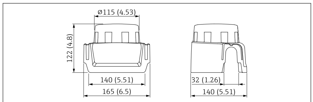
图 70 外形尺寸示意图。测量单位 mm (in)
