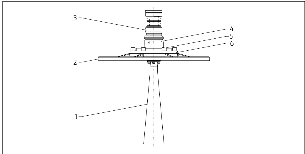
图 61 DN65 喇叭天线的材质; 带 UNI 法兰和天线角度调节装置。测量单位 mm (in)
