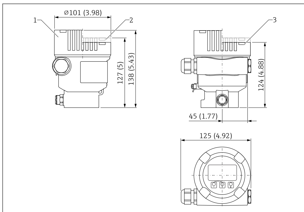
图 37 单腔室铝外壳的外形尺寸示意图。测量单位 mm (in)
