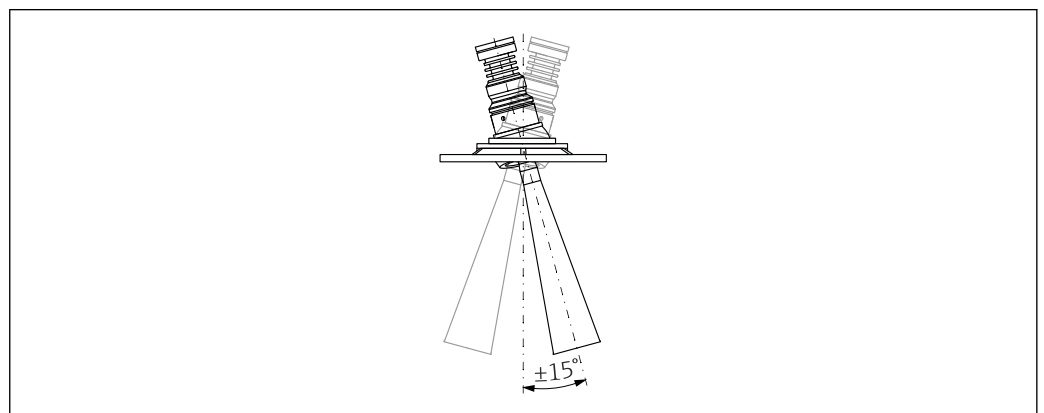
9 喇叭天线，带天线角度调节装置
