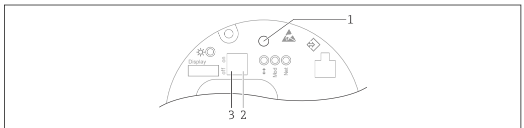
图 66 Ethernet-APL 电子插件上的操作按键和 DIP 开关
