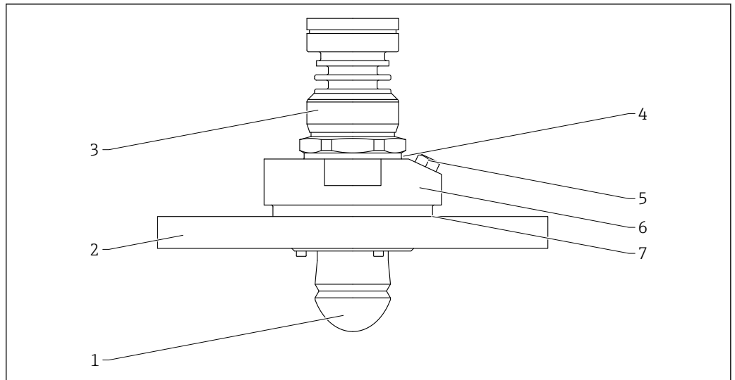
▣ 62 水滴型天线的材质；带空气吹扫接口。测量单位 mm (in)
