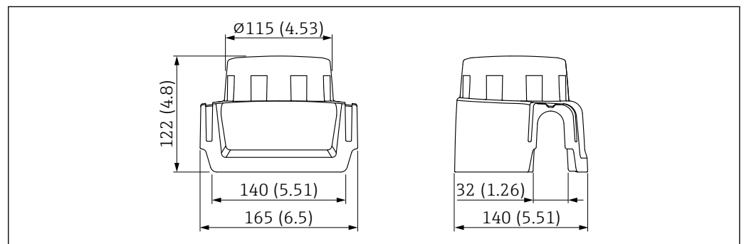
图 24 外形尺寸示意图。测量单位 mm (in)
