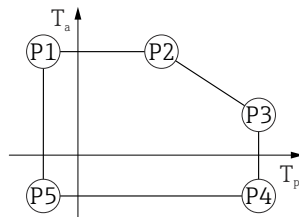
▣ 47 铝外壳, 带涂层; 过程温度范围: -40 ... +150 °C (-40 ... +302 °F)
