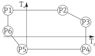
▣ 66 316L 外壳, 卫生型; 过程温度: -196 ... +200 °C (-320 ... +392 °F)
