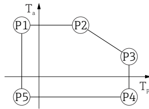
▣ 49 铝外壳, 带涂层; 过程温度: -40 ... +280 °C (-40 ... +536 °F)
