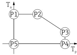
▣ 42 塑料外壳; 过程温度: 0 ... +150 °C (+32 ... +302 °F), 针对 CSA C/US 认证型仪表
