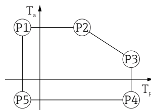
图 53 316L 外壳; 过程温度范围: -20 ... +150 °C (-4 ... +302 °F)
