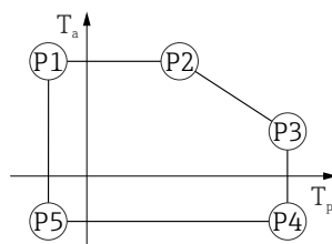
▣ 56 316L 外壳; 过程温度范围: -40 ... +200 °C (-40 ... +392 °F)
