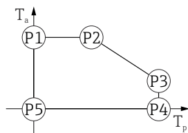
▣ 44 塑料外壳; 过程温度: 0 ... +200 °C (+32 ... +392 °F), 针对 CSA C/US 认证型仪表
