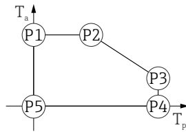
▣ 30 塑料外壳; 过程温度范围: 0 ... +150 °C (+32 ... +302 °F), 适用 CSA C/US 认证型仪表
