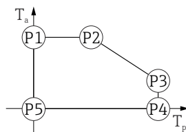
▣ 38 塑料外壳; 过程温度: 0 ... +280 °C (+32 ... +536 °F), 针对 CSA C/US 认证型仪表
