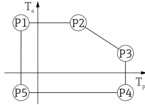
▣ 45 铝外壳, 带涂层; 过程温度范围: -20 ... +150 °C (-4 ... +302 °F)
