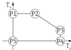
图 40 塑料外壳; 过程温度: 0 ... +450 °C (+32 ... +842 °F), 针对 CSA C/US 认证型仪表
