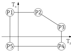
▣ 62 316L 外壳, 卫生型; 过程温度范围: -20 ... +200 °C (-4 ... +392 °F)
