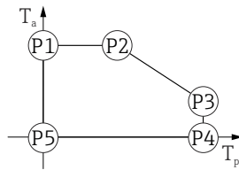
▣ 32 塑料外壳; 过程温度范围: 0 ... +200 °C (+32 ... +392 °F), 适用 CSA C/US 认证型仪表
