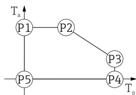
图 30 塑料外壳；过程温度范围：0 ... +150 °C (+32 ... +302 °F)，适用 CSA C/US 认证型仪表
