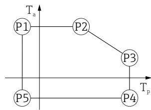
图 46 316L 外壳，卫生型；过程温度范围：-20 ... +200 °C (-4 ... +392 °F)
