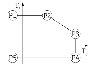
33 塑料外壳; 过程温度范围: -40 ... +150 °C (-40 ... +302 °F)
