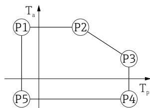
图 31 塑料外壳；过程温度范围：-20 ... +200 °C (-4 ... +392 °F)
