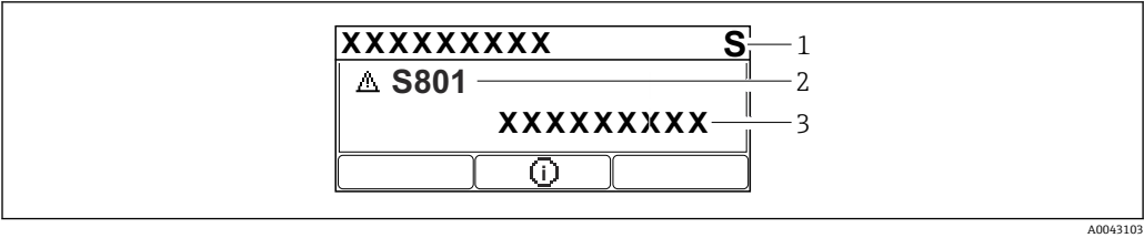
图 20 图形显示屏，带按键
