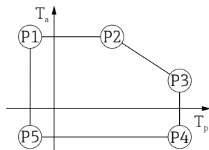
图 42 316L 外壳; 过程温度范围: -20 \dots +200 \text{ }^{\circ}\text{C} ( -4 \dots +392 \text{ }^{\circ}\text{F} )
