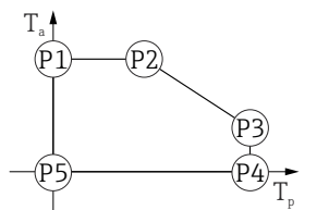
34 塑料外壳; 过程温度范围: 0 ... +150 °C (+32 ... +302 °F), 适用 CSA C/US 认证型仪表
