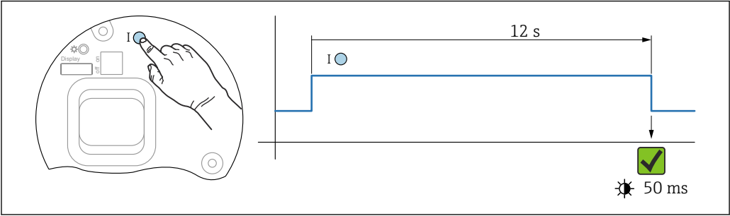
图 22 时序图 - 恢复出厂设置
