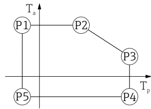
图 45 316L 外壳，卫生型；过程温度范围：-20 ... +150 °C (-4 ... +302 °F)
