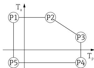
图 43 316L 外壳; 过程温度范围: -40 \dots +150 \text{ }^{\circ}\text{C} ( -40 \dots +302 \text{ }^{\circ}\text{F} )
