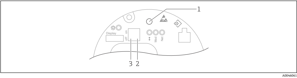
图 8 Ethernet-APL 电子插件上的操作按键和 DIP 开关
