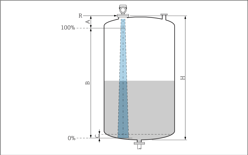
图 28 有效测量范围
