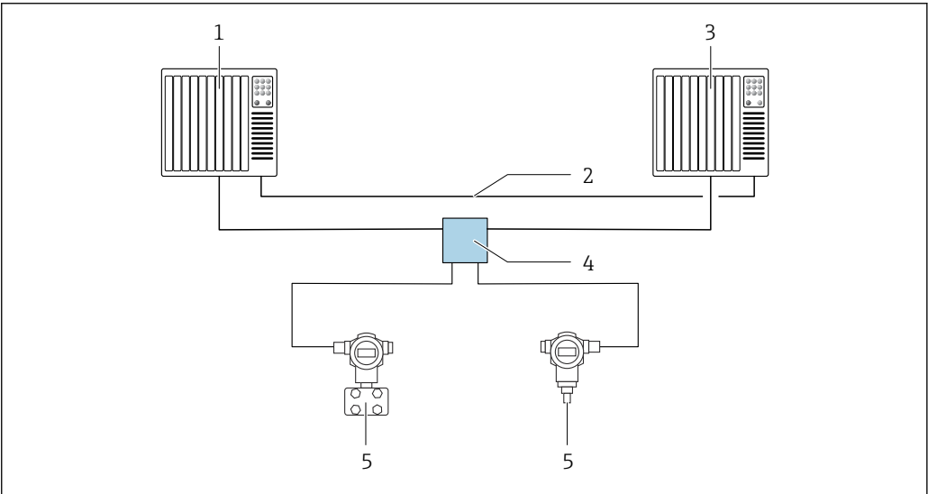
15 S2 系统冗余布局实例：星形拓扑结构
