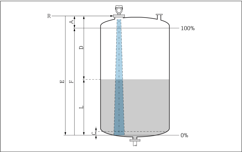
图 17 液位测量的设置参数
