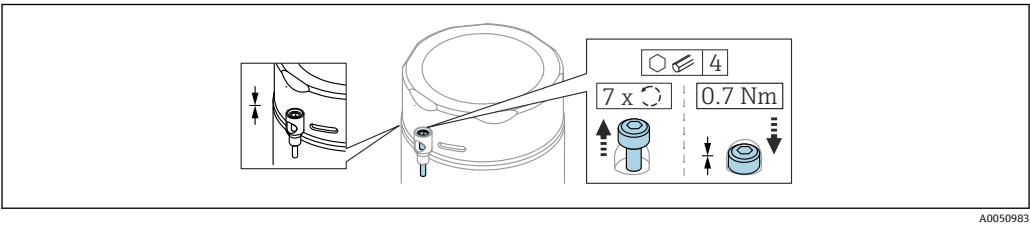
图 3 带锁定螺丝的外壳盖；卫生型外壳（仅适用于粉尘防爆场合）
