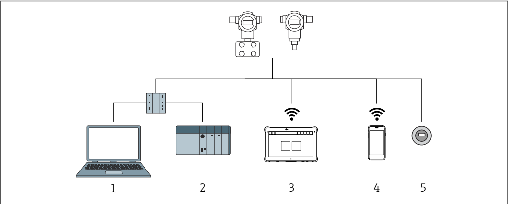
图 16 通过 PROFINET 通信实现远程操作
