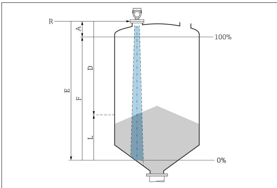
図 7 粉体のレベル測定用パラメータの設定
