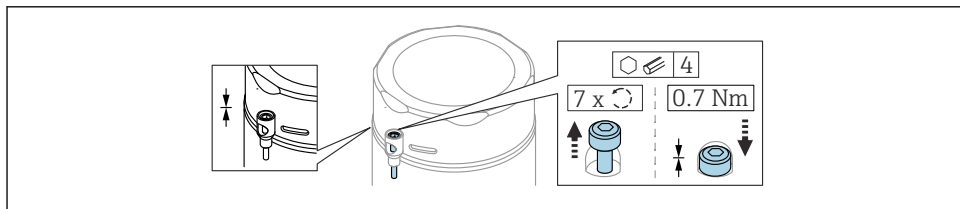
2 Cubierta con tornillo de fijación; caja de higiene (solo para protección contra explosiones por polvo)
