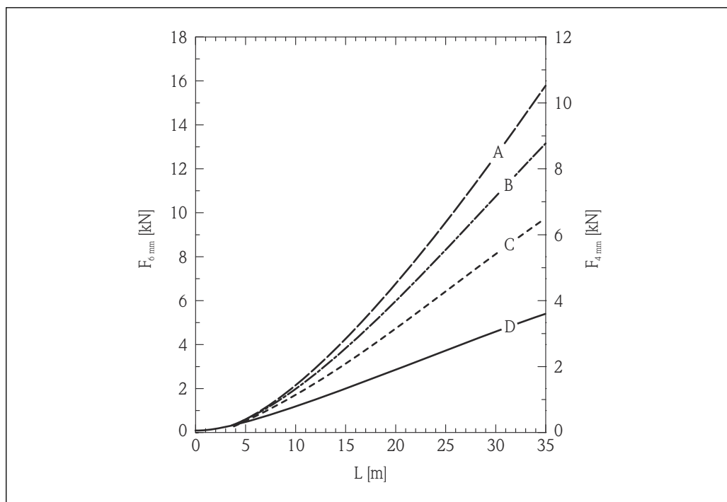
6 Полиэтиленовые гранулы в металлическом силосе с гладкими стенками; прочность на растяжение как функция уровня L для диаметров троса 6 мм (0,24 дюйм) и 4 мм (0,16 дюйм)
