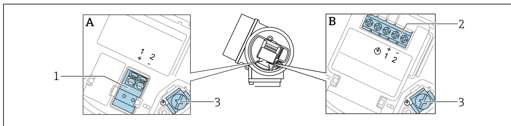
14 Назначение клемм, 2-проводное подключение: 4 до 20 мА HART
