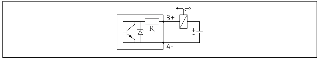
24 Подключение реле
