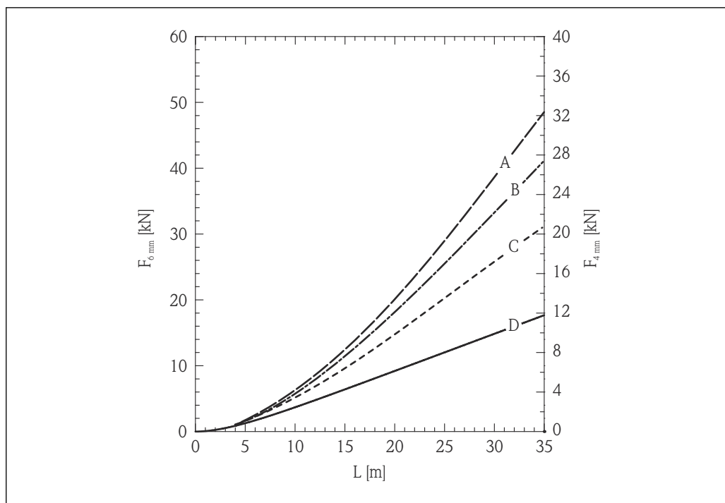
5 кварцевый песок в металлическом силосе с гладкими стенками; прочность на растяжение как функция уровня L для диаметров троса 6 мм (0,24 дюйм) и 4 мм (0,16 дюйм)
