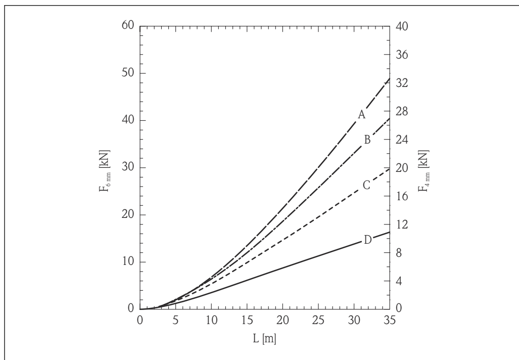
8 Цемент в металлическом силосе с гладкими стенками; прочность на растяжение как функция уровня L для диаметров троса 6 мм (0,24 дюйм) и 4 мм (0,16 дюйм)
