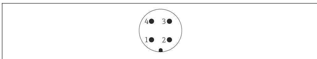
26 Назначение контактов разъема M12
