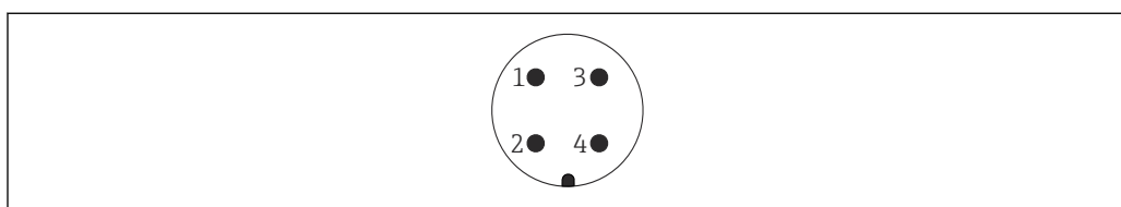
27 Назначение контактов разъема 7/8
