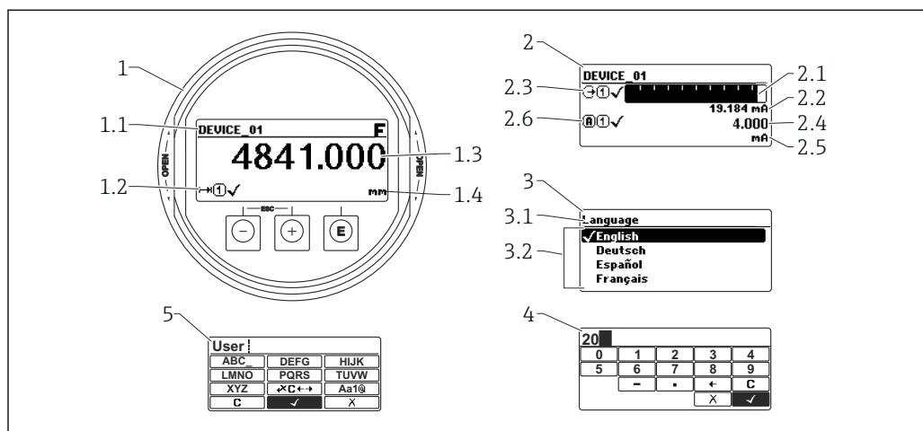
34 Формат индикации на блоке управления и дисплея
