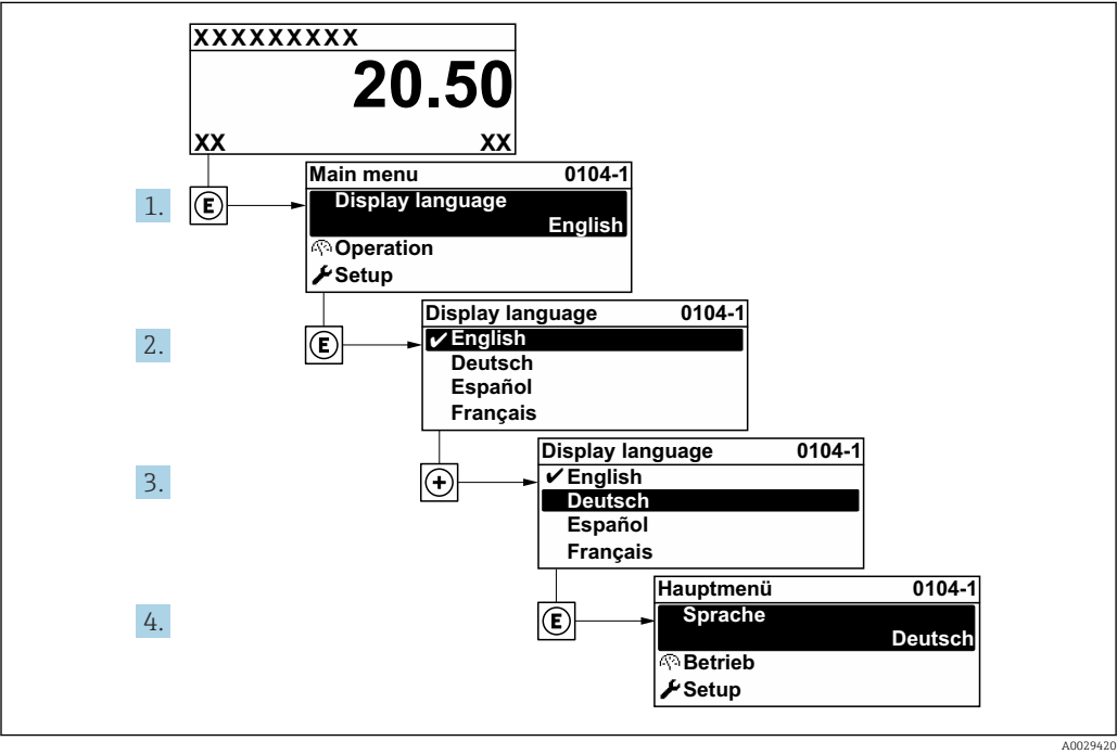
38 Пример конфигурации локального дисплея
