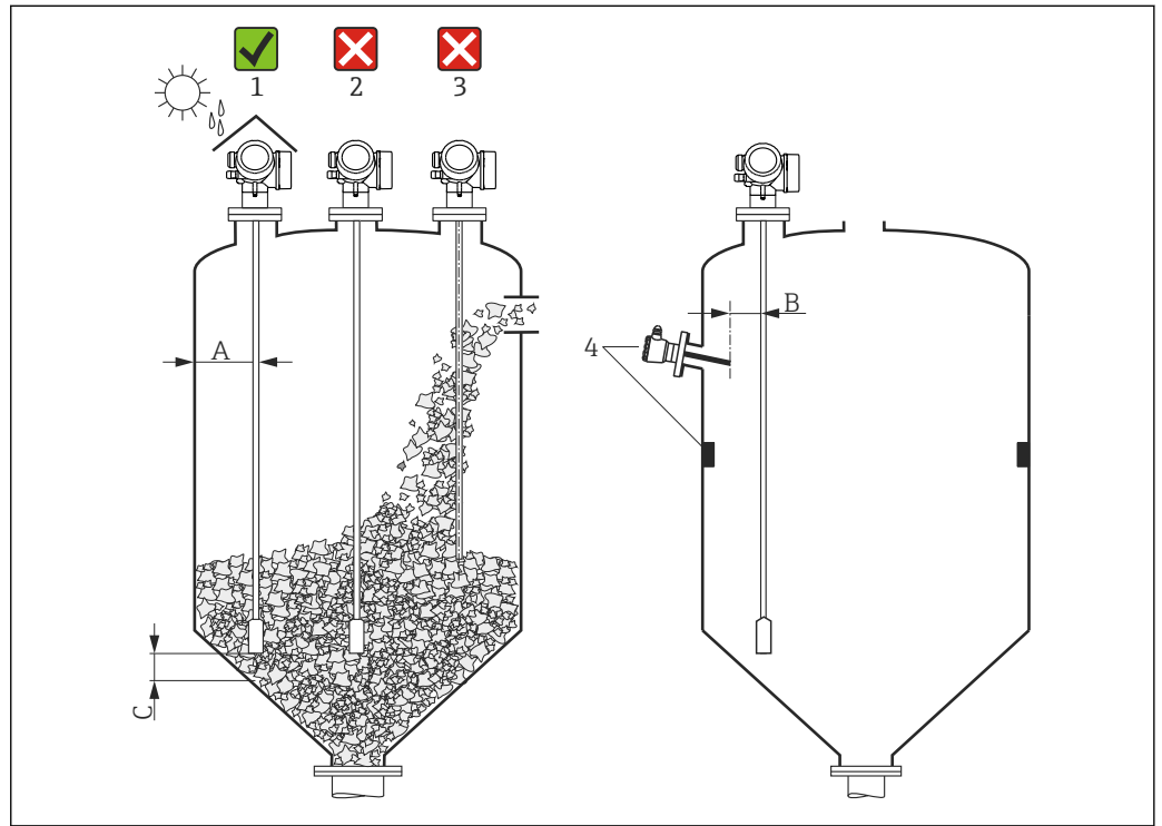
4 Условия монтажа Levelflex
