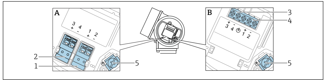
16 Назначение клемм, 2-проводное подключение: 4 до 20 мА HART, релейный выход
