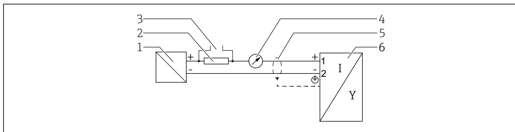
15 Блок-схема, 2-проводное подключение: 4 до 20 мА HART
