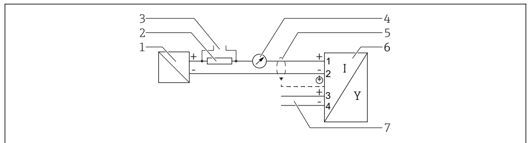
17 Блок-схема, 2-проводное подключение: 4 до 20 мА HART, релейный выход
