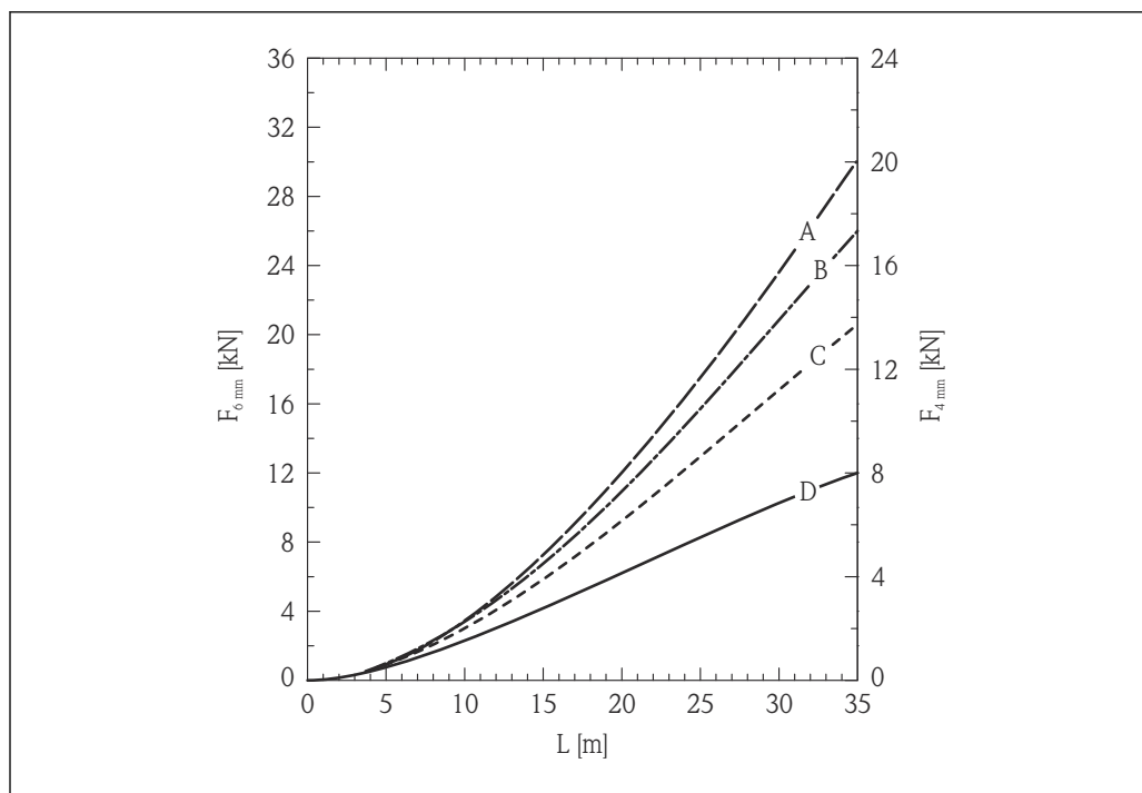
7 Пшеница в металлическом силосе с гладкими стенками; прочность на растяжение как функция уровня L для диаметров троса 6 мм (0,24 дюйм) и 4 мм (0,16 дюйм)
