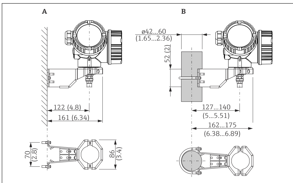
12 Монтаж корпуса электроники на монтажном кронштейне. Единица измерения мм (дюйм)
