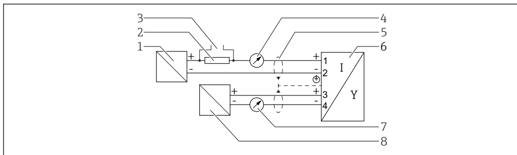
19 Блок-схема, 2-проводное подключение: 4 до 20 мА HART, 4 до 20 мА
