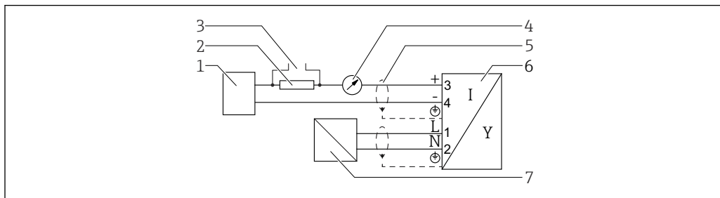
23 Блок-схема, 4-проводное подключение: 4 до 20 мА HART (90 до 253 V AC )
