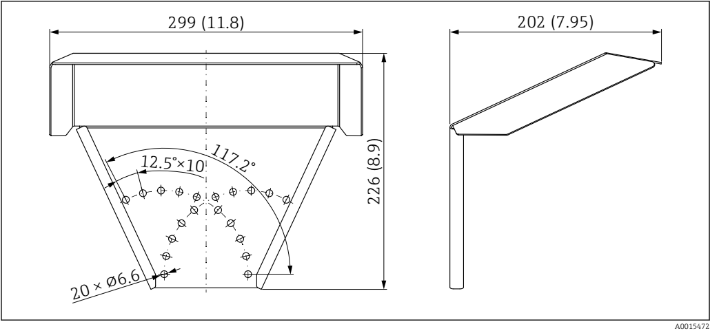
52 Dimensions. Unité de mesure mm (in)
