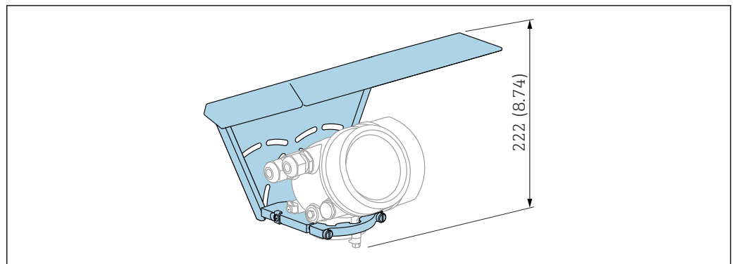
51 Hauteur. Unité de mesure mm (in)
