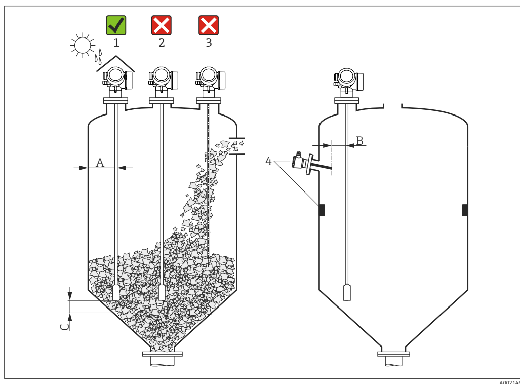
25 Conditions de montage pour le Levelflex
