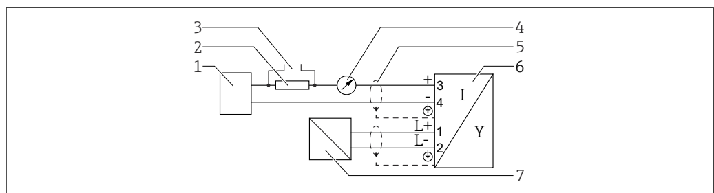
13 Schéma de principe, 4 fils : 4 ... 20 mA HART (10,4 ... 48 V DC )
