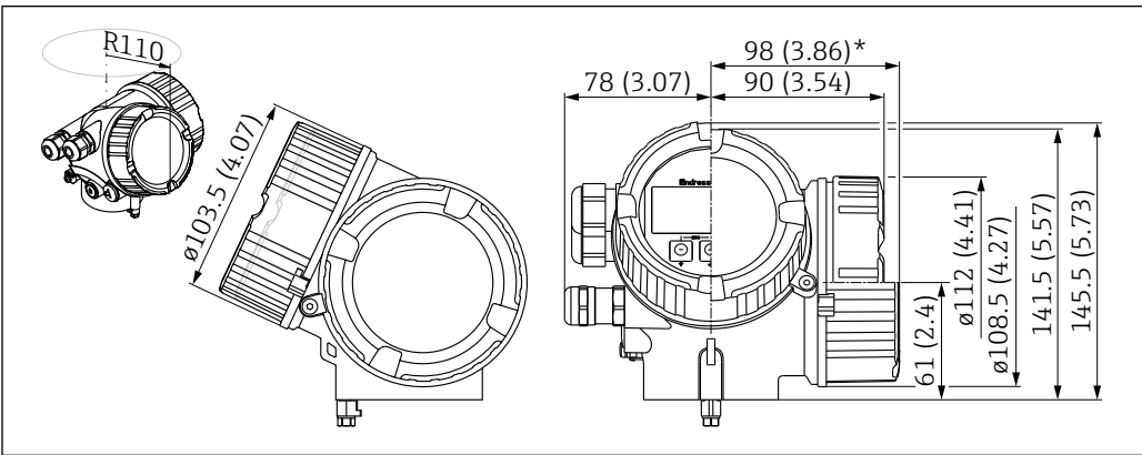
35 Boîtier GT20 (revêtu d'aluminium). Unité de mesure mm (in)
