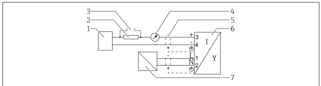
15 Schéma de principe, 4 fils : 4 ... 20 mA HART (90 ... 253 V AC )
