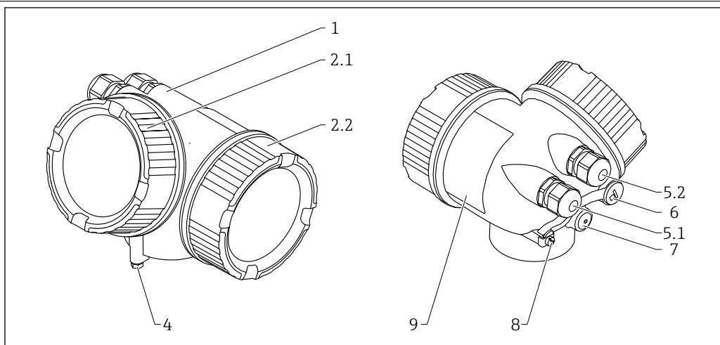
41 Matériau ; boîtier GT19
