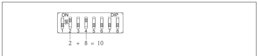
図 20 ハードウェアアドレス指定の例：スイッチ 8 を「オフ」位置にし、スイッチ 1~7 にアドレスを定義します。
