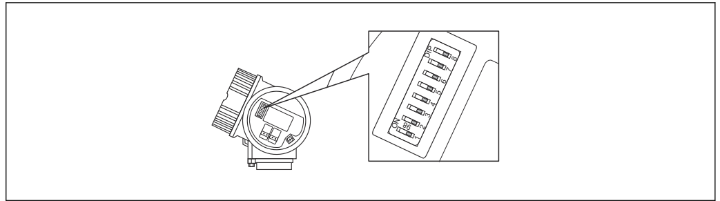
図 19 端子部のアドレススイッチ
