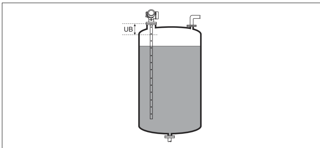
38 液体計測の不感知距離 (UB)
