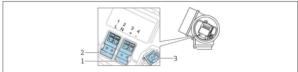
図 9 端子の割当て、4線式：4～20 mA HART (90～253 V AC )
