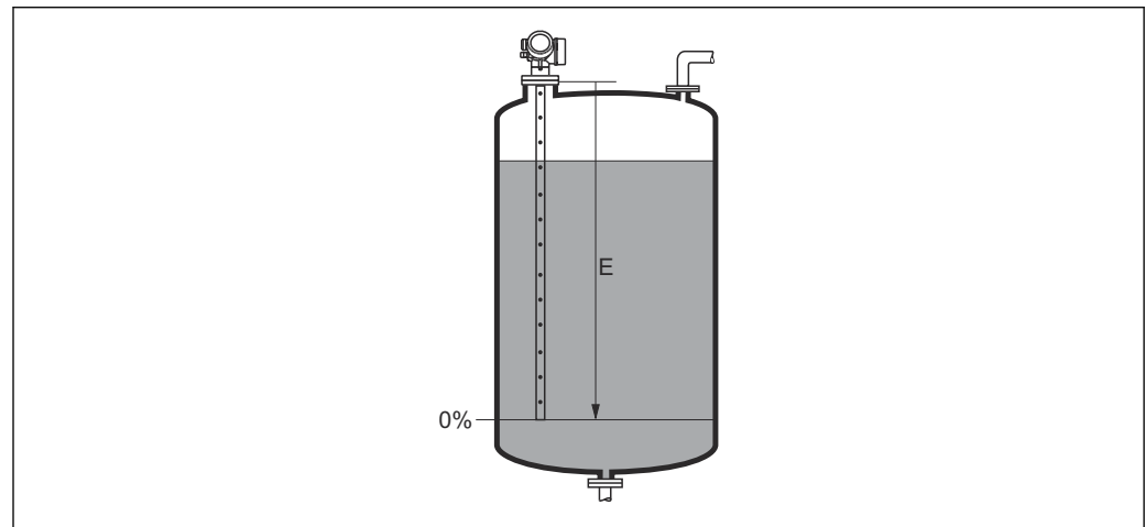
🔍 31 液体レベル測定用の空校正 (E)
