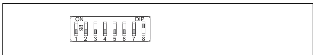
図 21 ソフトウェアアドレス指定の例：スイッチ 8 を「オン」位置にし、アドレスは操作メニューで定義します（設定 → 機器アドレス）。
