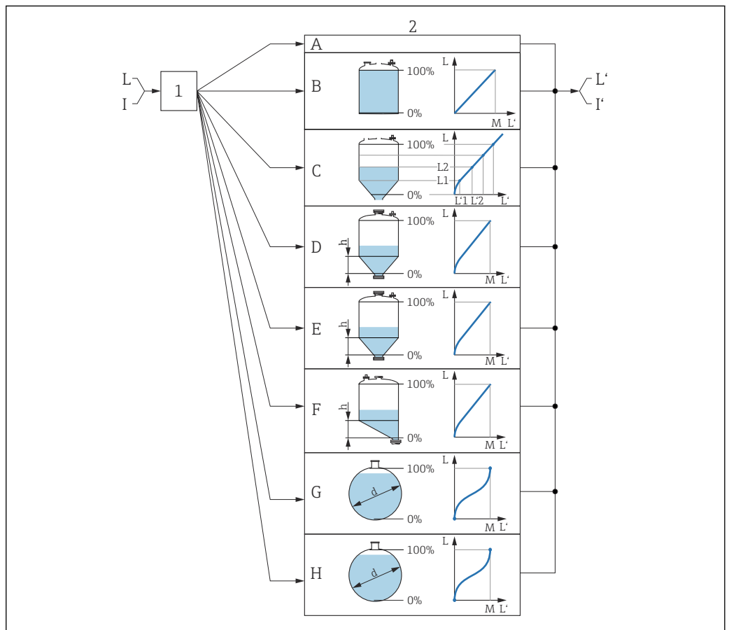
36 リニアライゼーション：レベルから、および（該当する場合は）界面から体積または質量に変換。変換は容器の形状に依存
