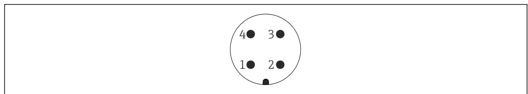
図 14 M12 プラグのピン割当て
