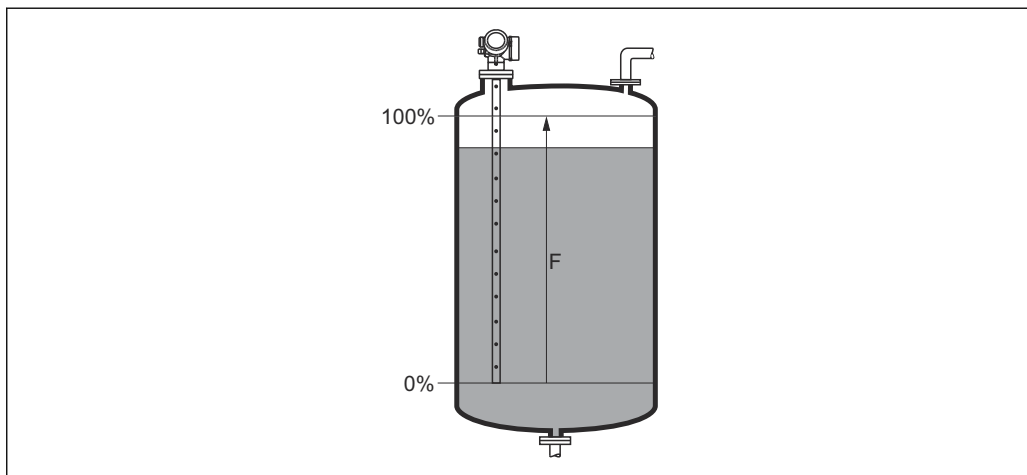
☐ 32 液体レベル測定用の満量校正 (F)
