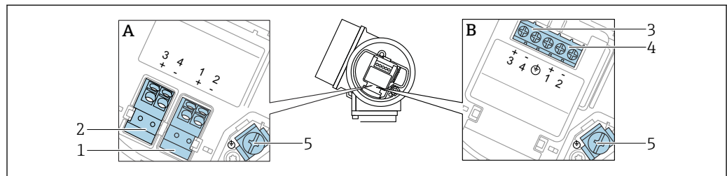
図 10 端子の割当て PROFIBUS PA / FOUNDATION フィールドバス
