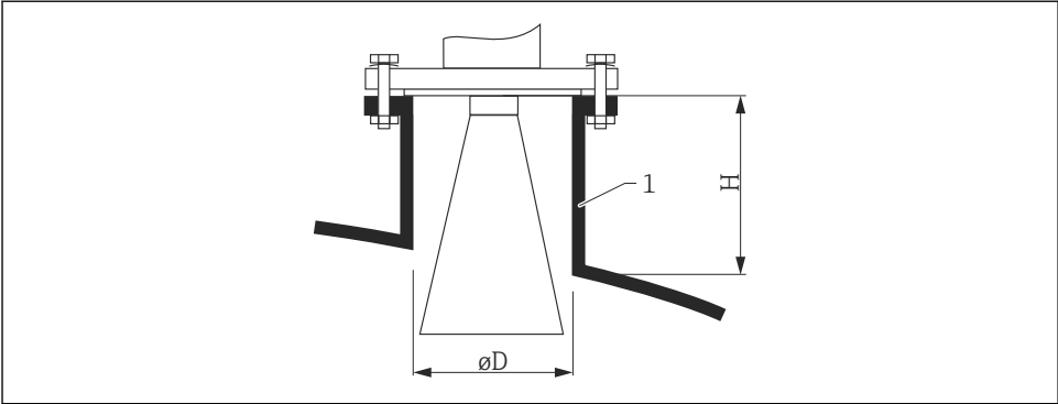
3 喇叭天线的安装短管高度和管径示意图
