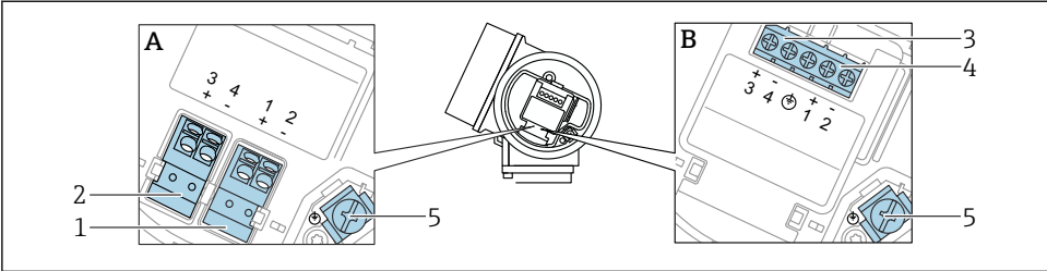
4 接线端子分配 PROFIBUS PA / FOUNDATION Fieldbus
