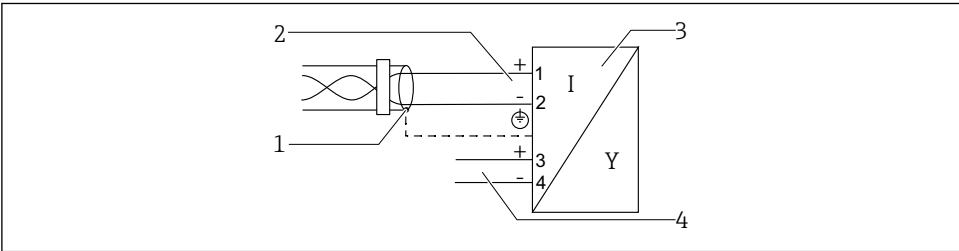
5 接线图: PROFIBUS PA / FOUNDATION Fieldbus
