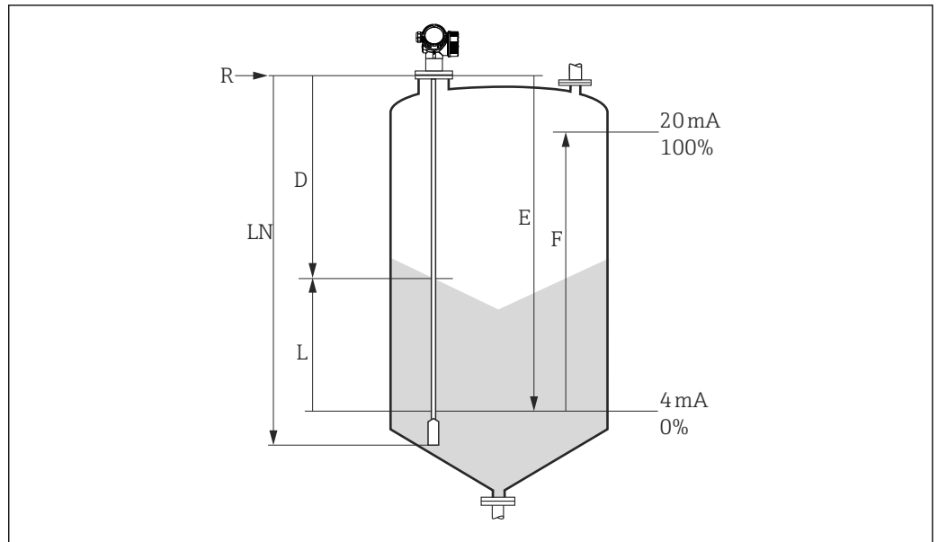
28 Paramètres de configuration pour la mesure de niveau dans les solides en vrac
