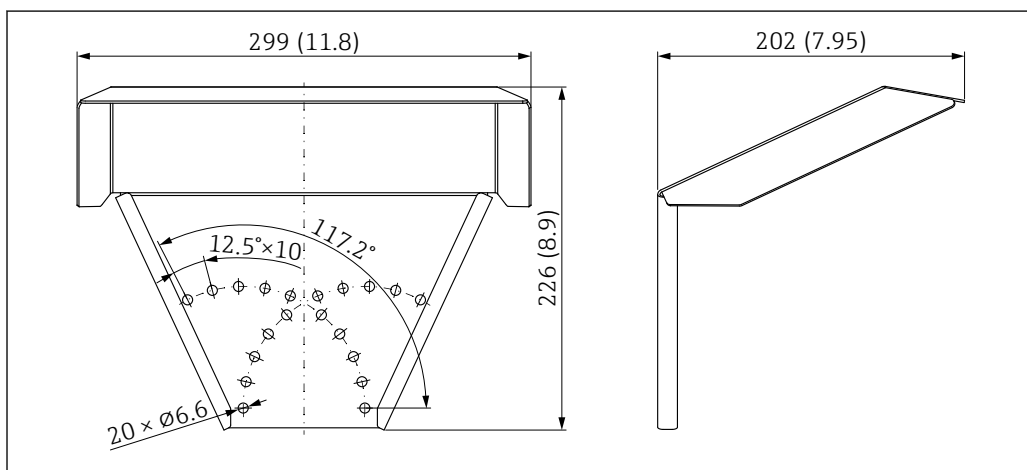
33 Dimensions. Unité de mesure mm (in)
