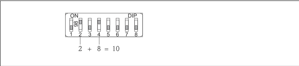
25 Exemple pour l'adressage hardware ; le commutateur 8 est en position "OFF" ; les commutateurs 1 à 7 définissent l'adresse.
