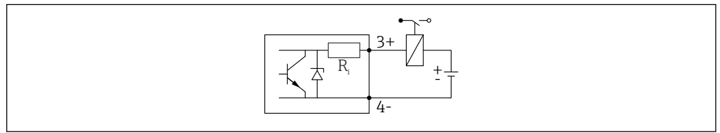
17 Raccordement d'un relais
