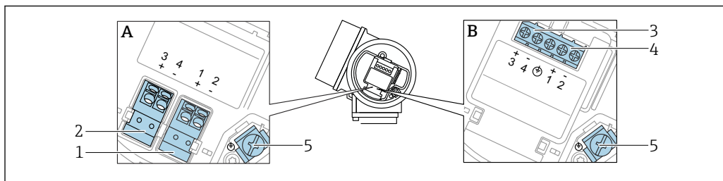
15 Affectation des bornes PROFIBUS PA / FOUNDATION Fieldbus
