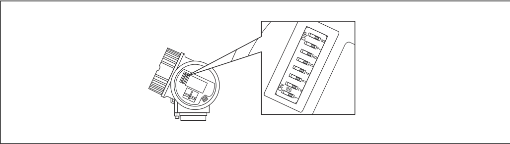
24 Commutateur d'adresses dans le compartiment de raccordement
