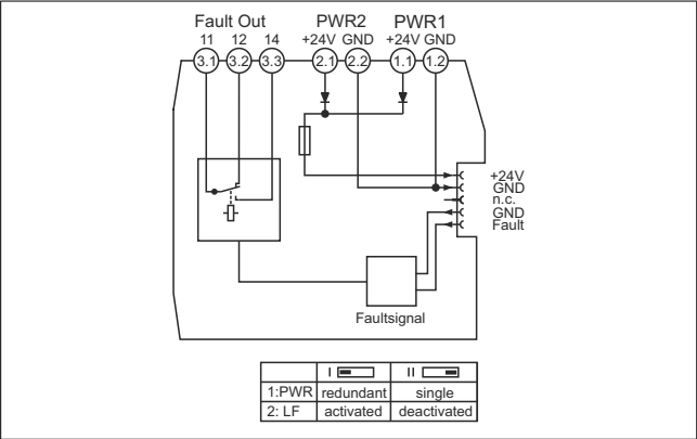
図 2 RNF22 端子の割当て：電源モジュールおよびエラー伝送モジュール
