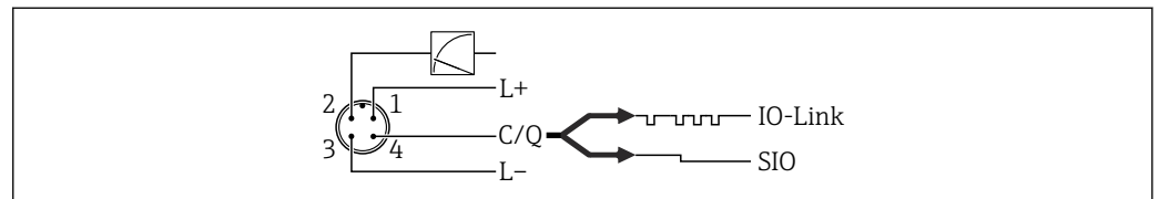
図 1 M12 プラグ
