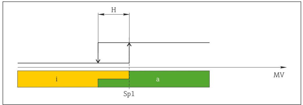
図 2 SSC、1点
