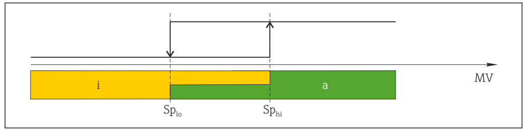
図 4 SSC、2点
