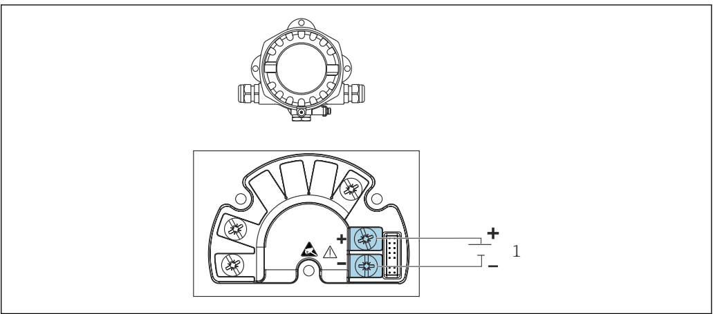
3 Asignación de terminales del indicador de campo
