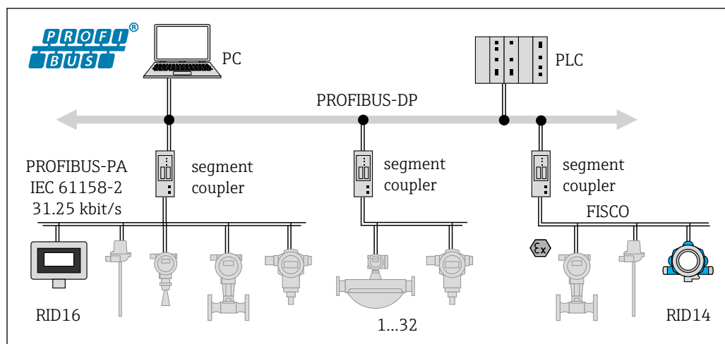
2 Integración en un sistema con el PROFIBUS® PA
