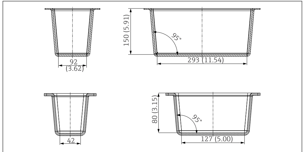
37 Большой калибровочный резервуар (вверху) и малый калибровочный резервуар (внизу). Единица измерения: мм (дюйм)
