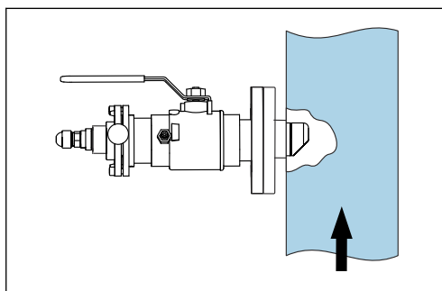
13 Монтаж с выдвижной арматурой CUA451
