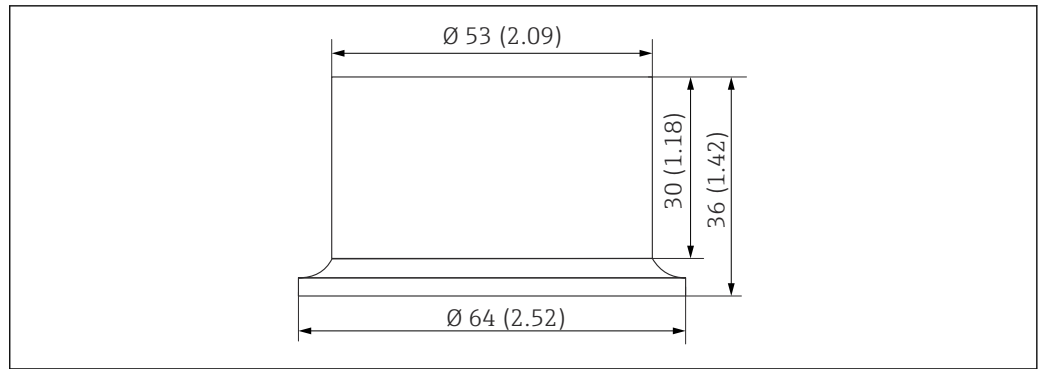
38 Приварной переходник. Размеры в мм (дюймах)
