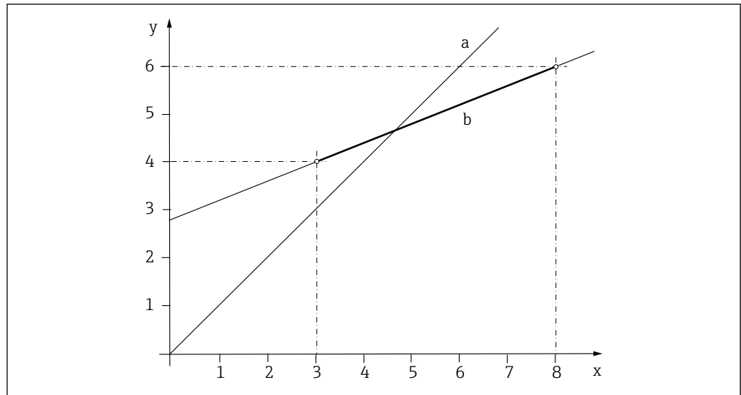
30 Принцип 2-точечной калибровки
