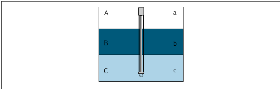
13 Wasserstandsmessung in drei Schichten
