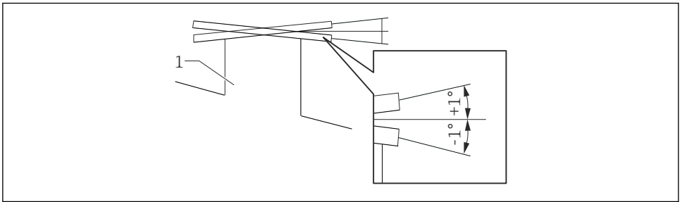
18 Zulässige Neigung des Montageflansches
