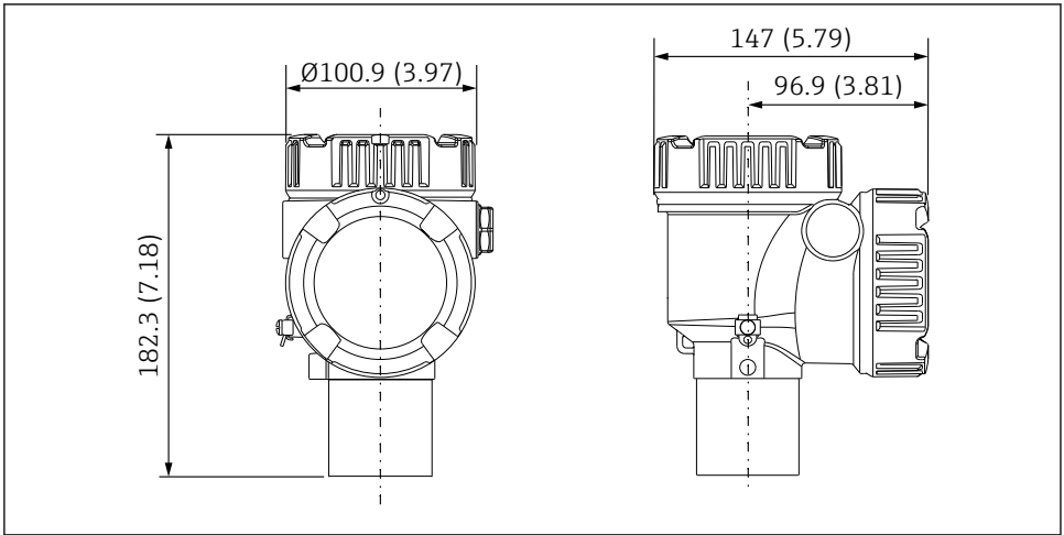
3 Standardmessumformer. Maßeinheit mm (in)
