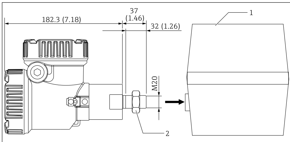
5 Option 2: Messumformer (Varec 1700, M20-Schraubverbindung). Maßeinheit mm (in)
