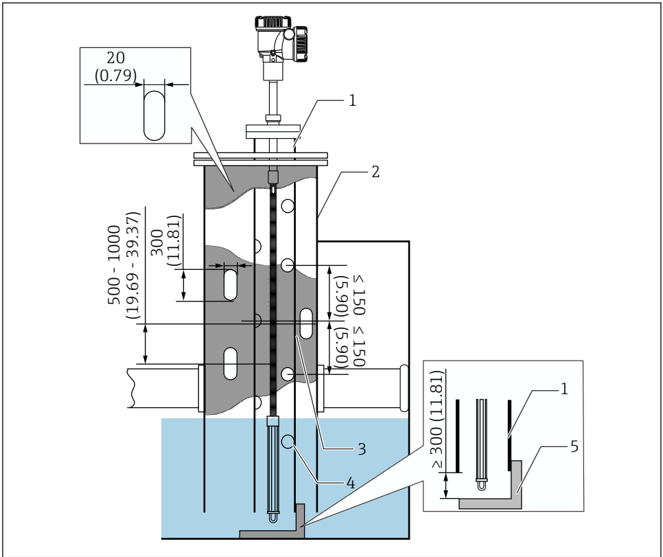
29 Montage im Schwallrohr. Maßeinheit mm (in)
