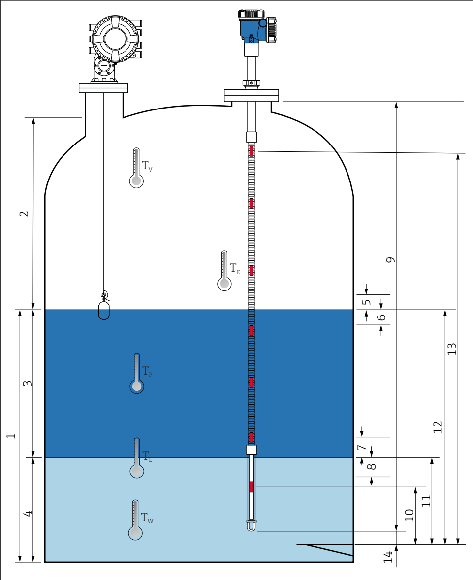
38 Auf den Einbau des NM81 bezogene Fachbegriffe
