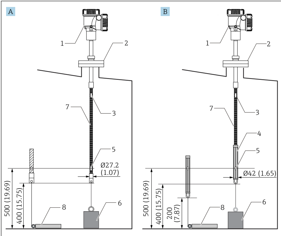
26 Montage mit Ankergewicht. Maßeinheit mm (in)
