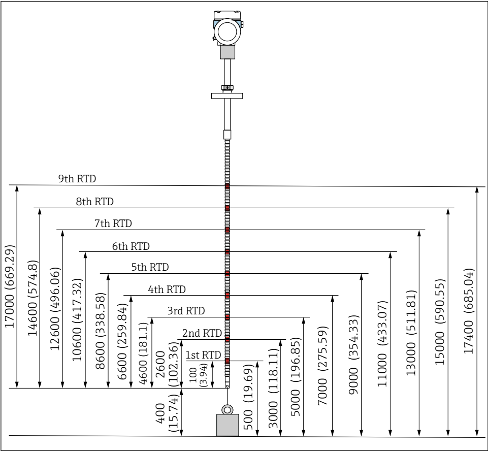
11 Elementposition. Maßeinheit mm (in)
