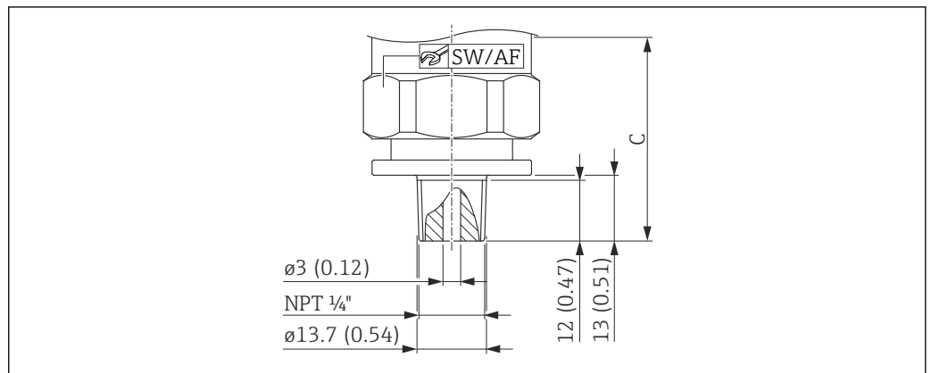
7 ASME 1/4" MNPT, furo 3 mm (0.12 in). Unidade de medida mm (in)
