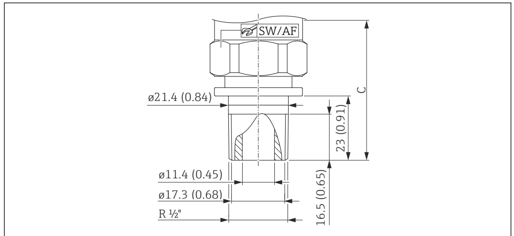
11 Diâmetro da membrana do processo: 17.2 mm (0.68 in). Unidade de medida mm (in)
