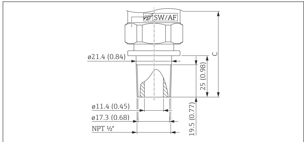
9 ASME 1/2" MNPT, furo 11.4 mm (0.45 in). Unidade de medida mm (in)
