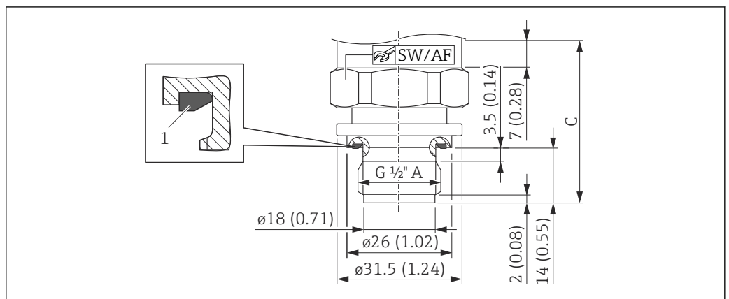
12 DIN 3852, Forma E. Diâmetro da membrana de processo: 17.2 mm (0.68 in). Unidade de medida mm (in)
