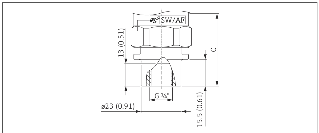
4 Rosca ISO 228 G 1/4" (fêmea). Unidade de medida mm (in)
