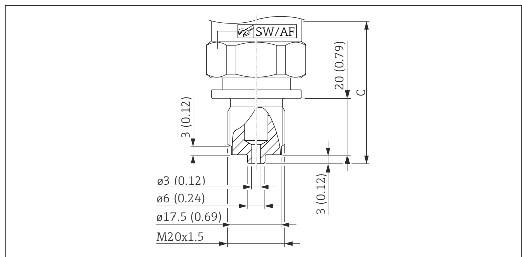
10 DIN 13 M20 x 1,5, EN 837, furo 3 mm (0.12 in). Unidade de medida mm (in)
