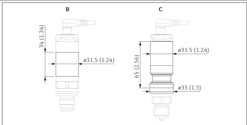
Unidade de medida mm (in)
