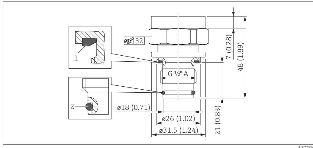
13 Diâmetro da membrana do processo: 17.2 mm (0.68 in). Unidade de medida mm (in)
