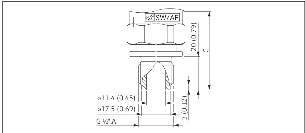
6 Rosca ISO 228 G 1/2" A, furo 11.4 mm (0.45 in). Unidade de medida mm (in)
