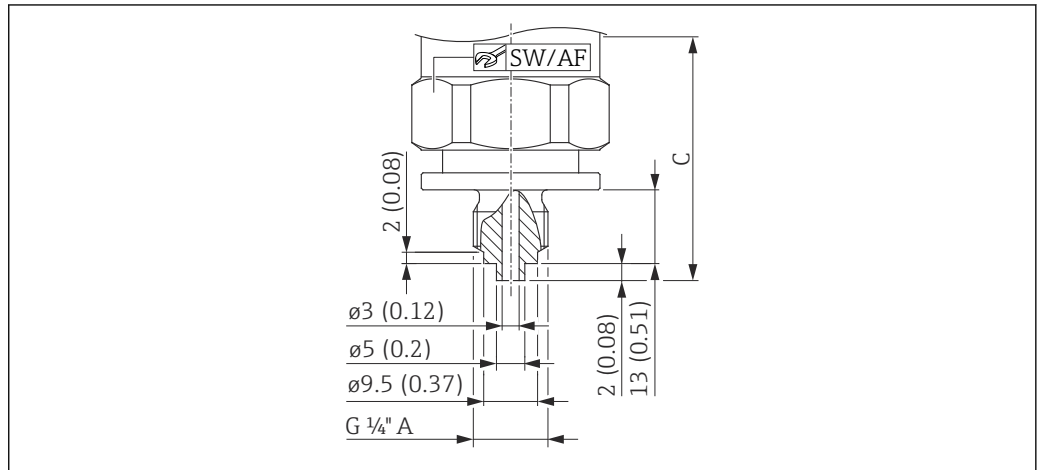
3 Rosca ISO 228 G 1/4" A, EN 837. Unidade de medida mm (in)
