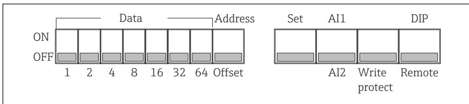
图 11 DIP 开关分配
