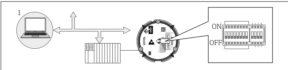
10 总线型数显仪的硬件设置
