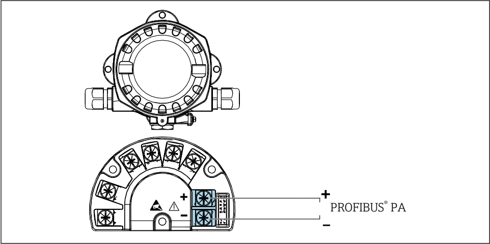
图 5 接线端子分配
