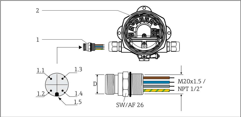
图 7 连接 PROFIBUS® PA 现场总线的连接头
