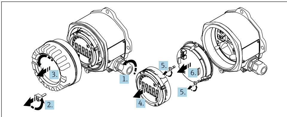
图 4 打开总线型数显仪外壳
