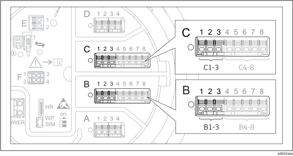
图 25 用作模拟量输出的模拟量输入/输出模块的安装位置示意图。设备的订货号确定当前使用的模块。
