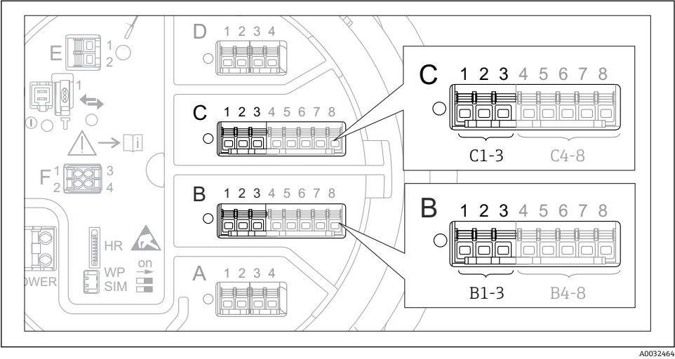
图 20 用作 4...20 mA 输入的模拟量输入/输出模块的安装位置示意图。设备的订货号确定当前使用的模块。
