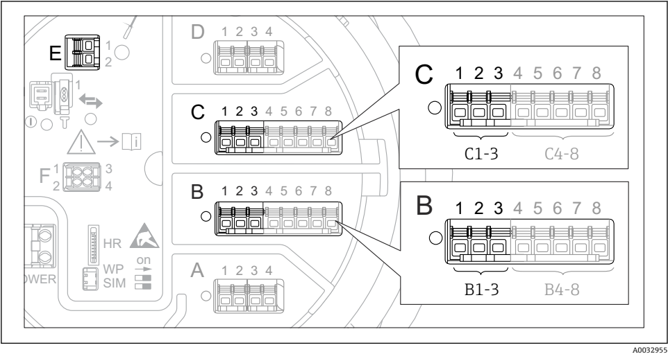
图 19 HART 回路的可能接线端子
