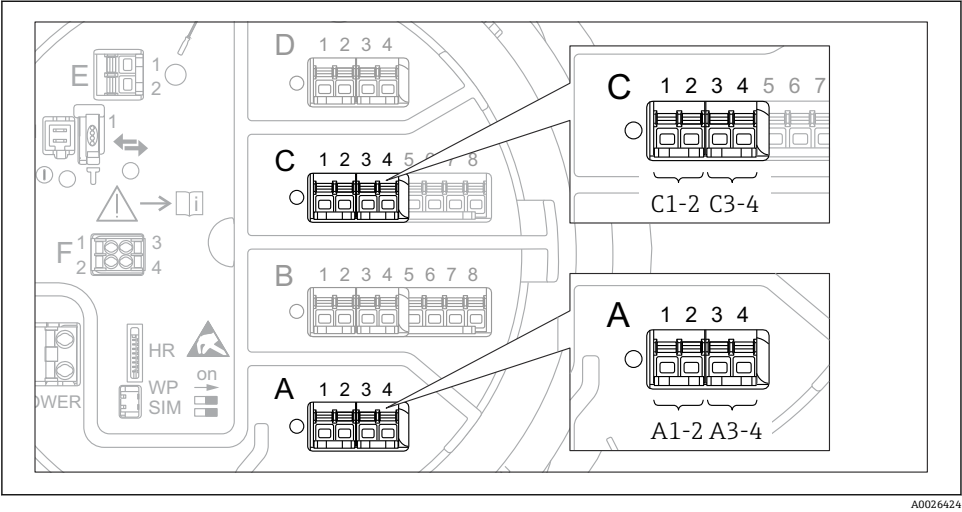
图 23 数字量输入/输出模块的可能安装位置（示例）；订货号确定数字量输入模块的数量和位置。
