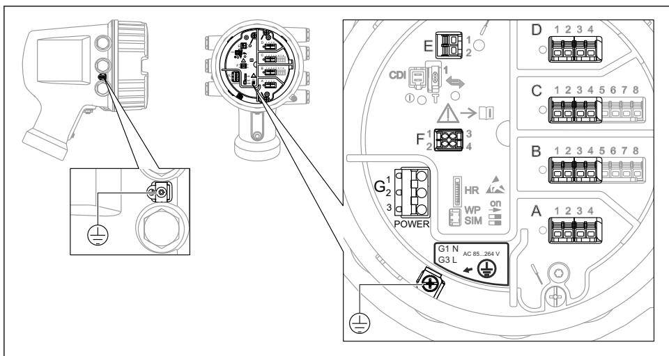
图 3 端子接线腔（典型实例）和接地端子示意图
