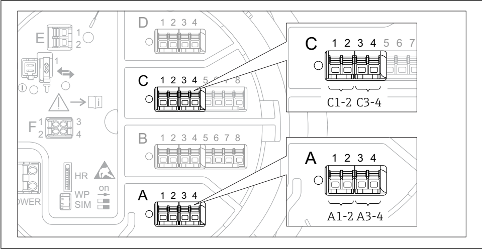
13 数字量输入或输出示例
