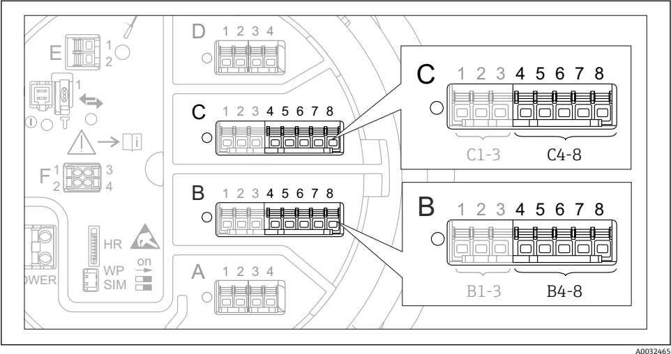
图 22 已连接 RTD 的模拟量输入/输出模块的安装位置示意图。设备的订货号确定当前使用的模块。
