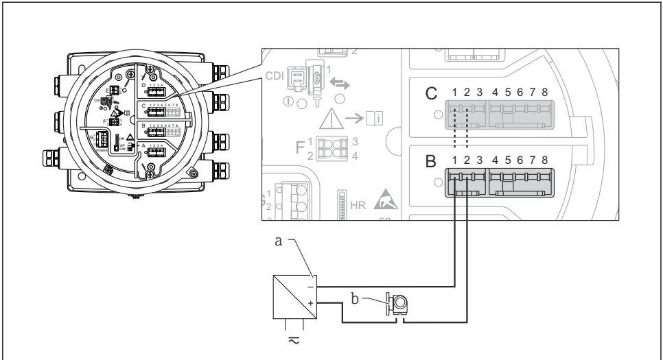
图 8 输入模式下的无源模拟量输入/输出模块
