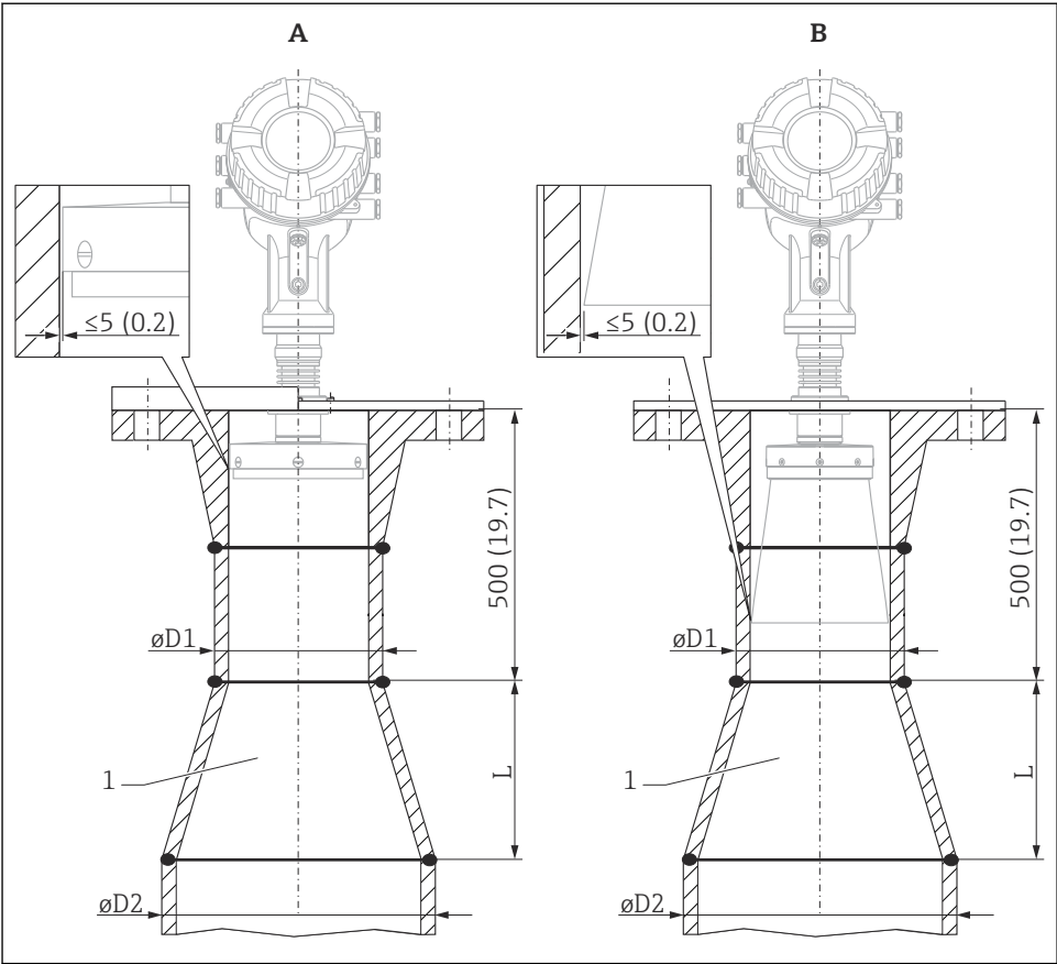
图 2 在较大管径的导尿管中安装 NMR84
