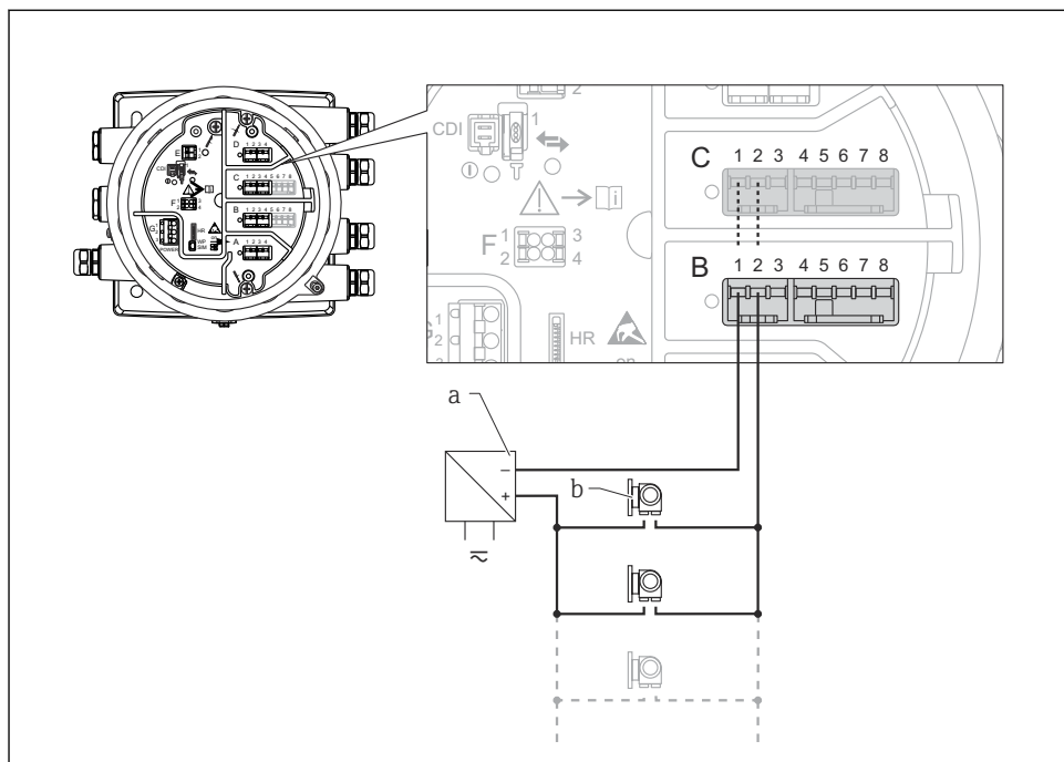
9 HART 主站模式下的无源模拟量输入/输出模块
