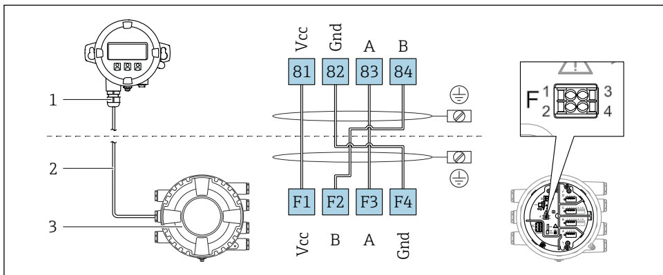
图 5 分离型显示单元与操作单元 DKX001 连接至罐旁指示仪 (NMR8x、NMS8x 或 NRF8x)
