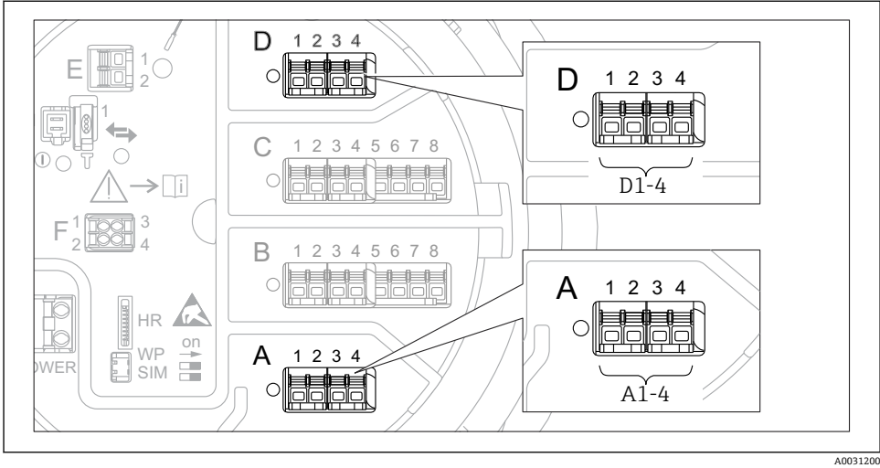
图 26 Modbus 模块或 V1 模块的安装位置示意图；取决于设备版本号，上述模块也可以安装在插槽 B 或 C 中。
