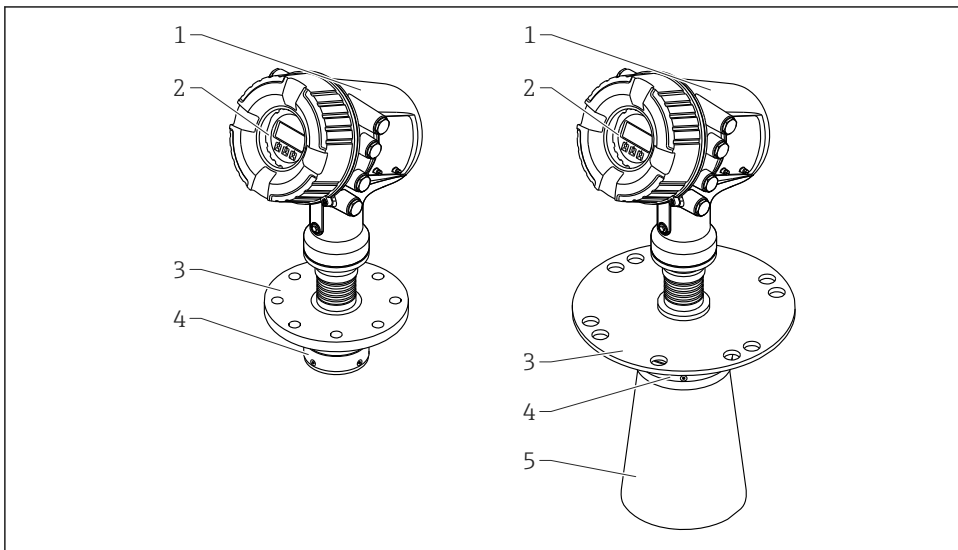
图 1 Micropilot NMR84 的结构示意图
