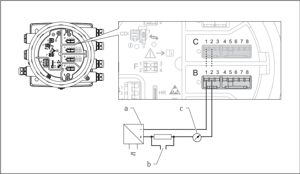
图 7 输出模式下的无源模拟量输入/输出模块
