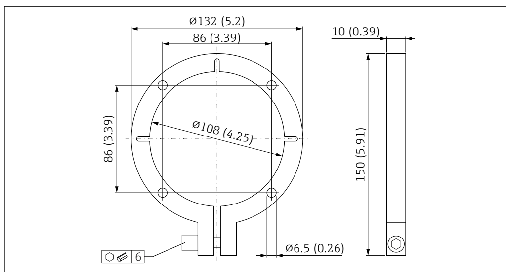
20 Flangia di montaggio, 1,4301, per sensore rotondo in versione corta o in versione media
