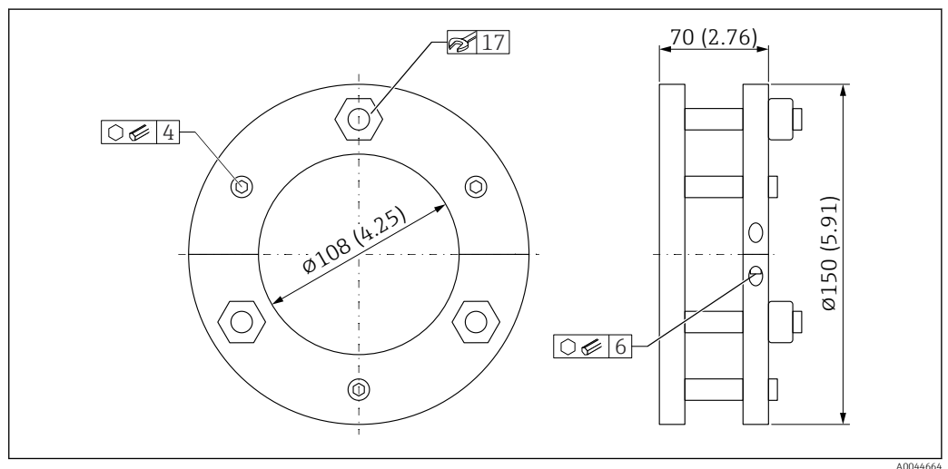
22 Telaio di montaggio, in acciaio zincato, per sensore rotondo, versione lunga
