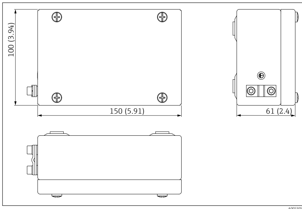
10 Dimensione della custodia elettronica ATEX. Unità di misura mm (in)
