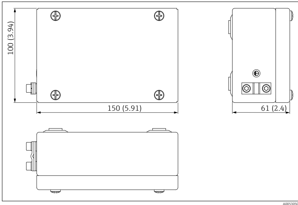
10 Afmetingen van de ATEX-elektronicabehuizing. Maateenheid mm (in)
