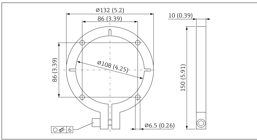
19 Bride de montage, 1.4301, pour capteur rond, version courte, ou capteur rond, version intermédiaire
