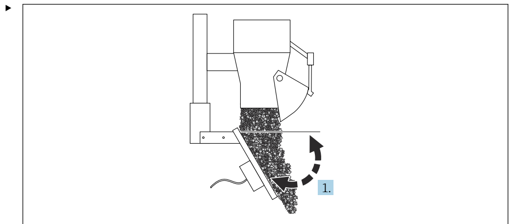
9 Solides en vrac abrasifs, positionnement de la plaque d'impact – trappe d'ouverture
