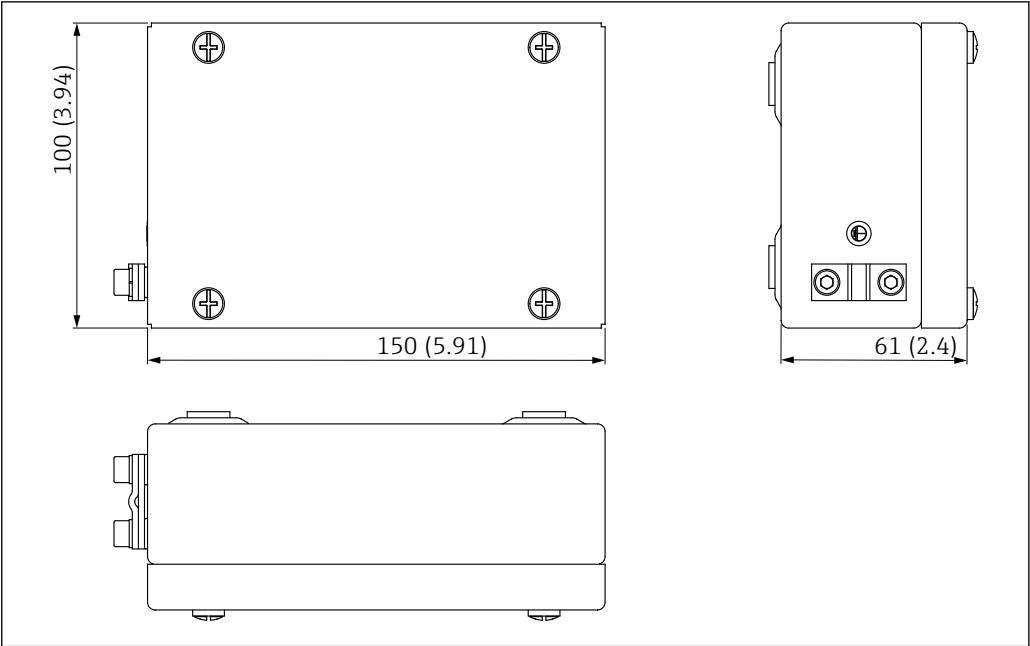
21 Dimensions du boîtier électronique ATEX. Unité de mesure mm (in)
