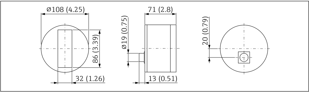
18 Dimensions du capteur rond, intermédiaire. Unité de mesure mm (in)
