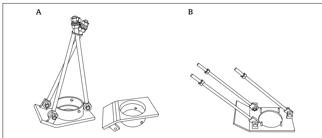
11 Chariot coulissant
