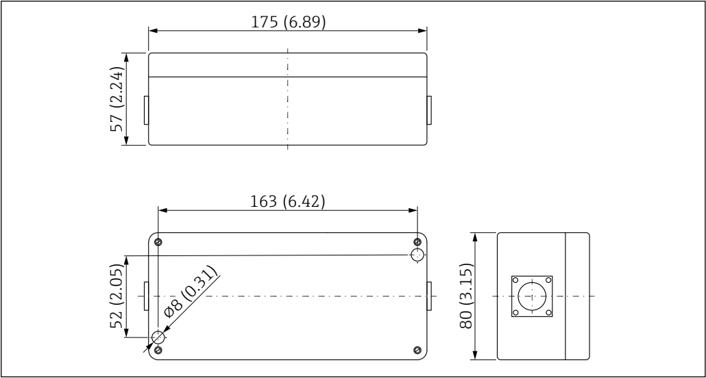
22 Dimensions du boîtier pour le module électronique déporté. Unité de mesure mm (in)
