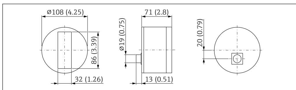
18 Размеры среднего круглого датчика. Единица измерения мм (дюйм)
