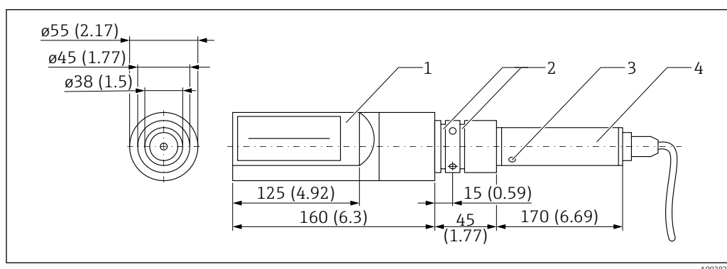
23 Размеры стержневого датчика. Единица измерения мм (дюйм)
