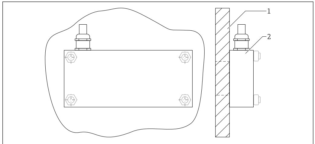
5 Смонтированный прямоугольный датчик, вид сзади
