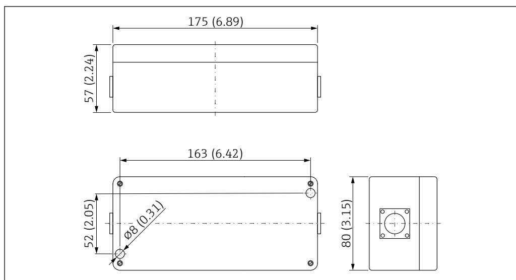
22 Размеры корпуса для выносного модуля электроники. Единица измерения мм (дюйм)
