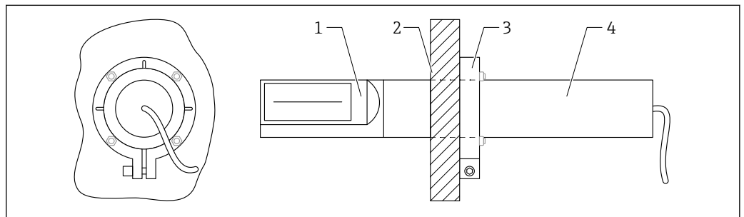
6 Смонтированный стержневой датчик, вид сзади
