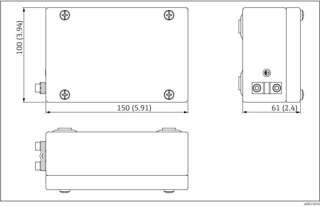
21 Размеры взрывозащищенного корпуса электроники. Единица измерения мм (дюйм)
