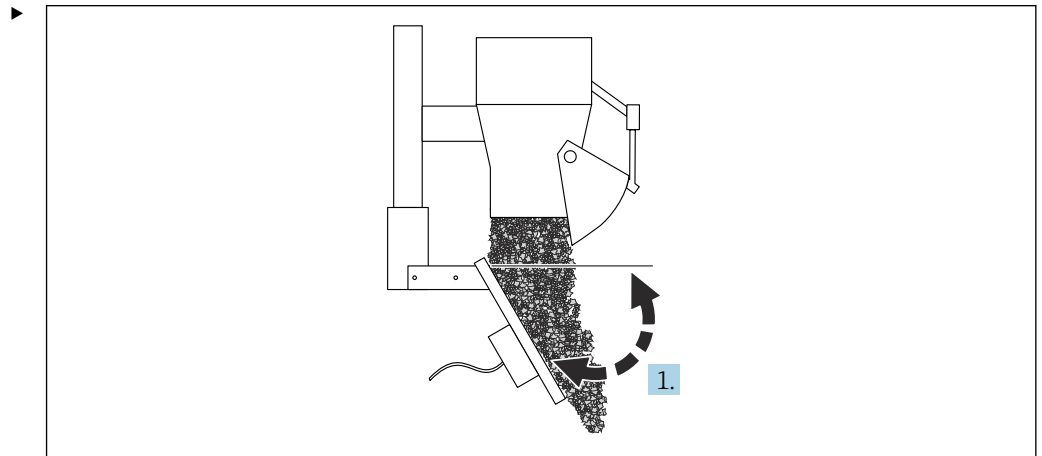
9 Абразивные сыпучие материалы, положение перегородки – открывающийся люк
