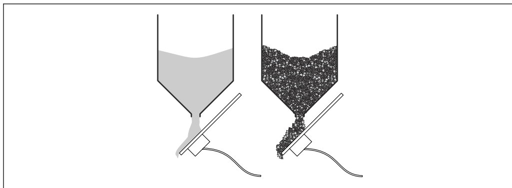
7 Монтаж круглого датчика для измерения влажности песка и гравия под выгрузным люком силоса
