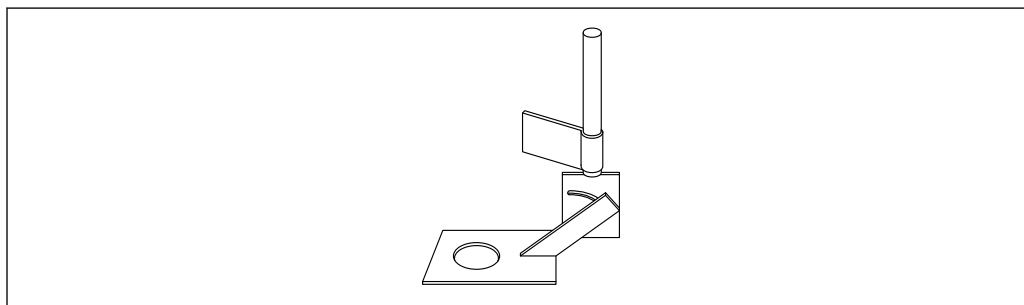
31 Универсальный держатель (1.4301) с механизмом наклона и удерживающей головкой, вырез для датчика \varnothing 108 мм (4,25 дюйм)
