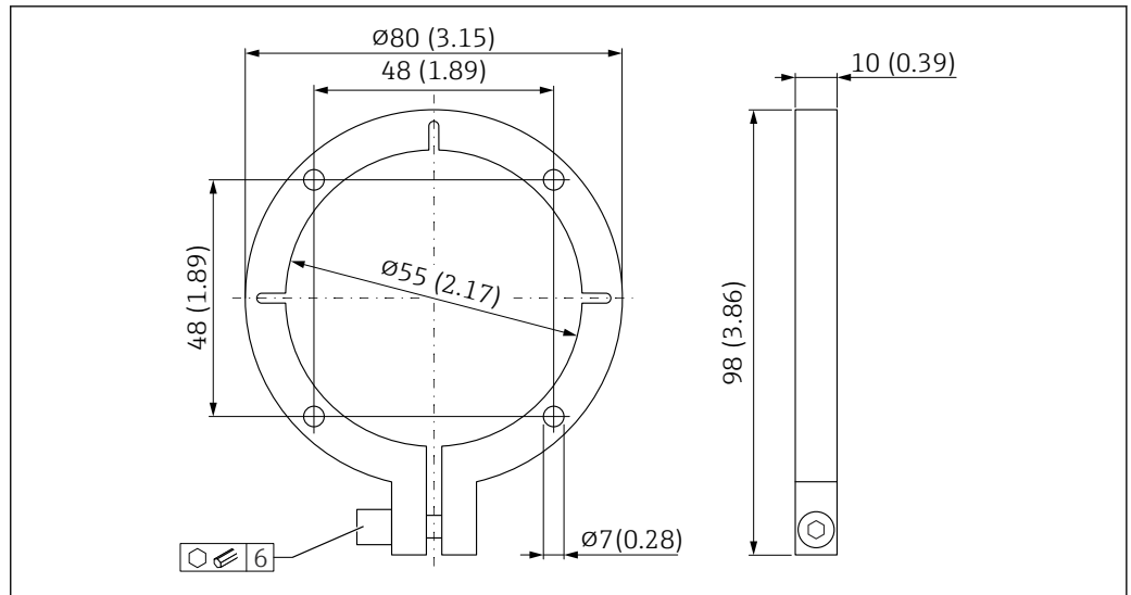
24 Монтажный фланец (1.4301) для стержневого датчика
