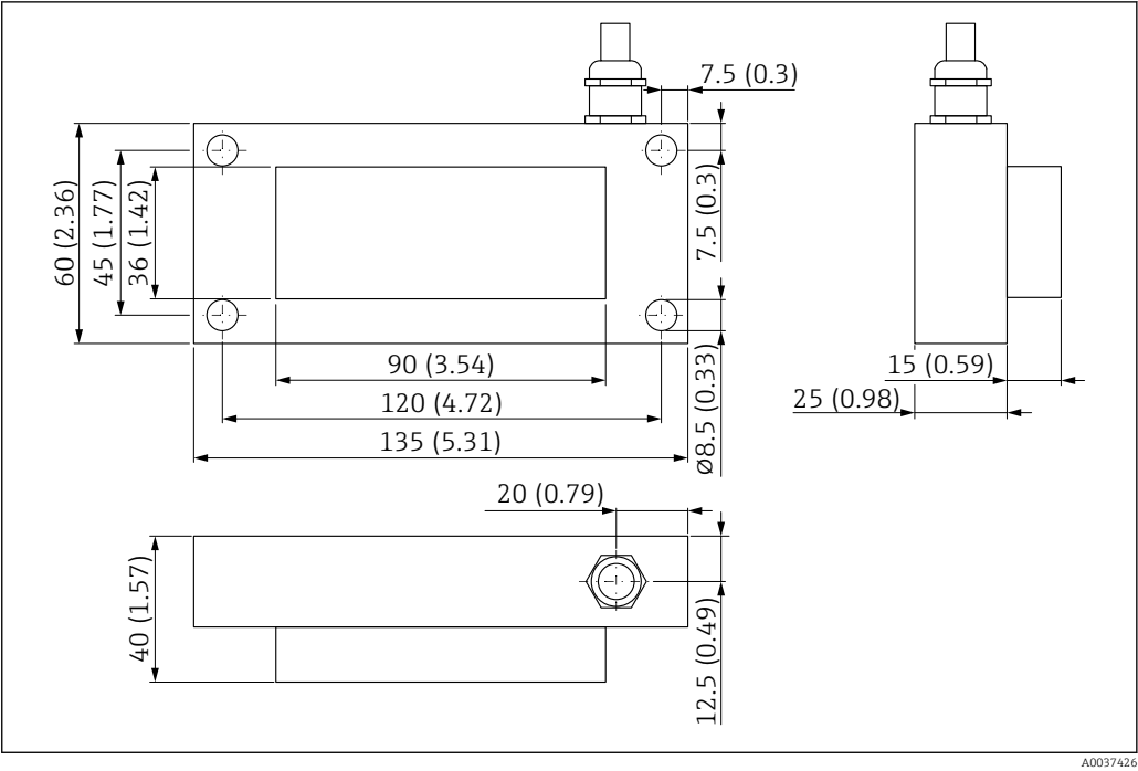
20 Размеры прямоугольного датчика. Единица измерения мм (дюйм)
