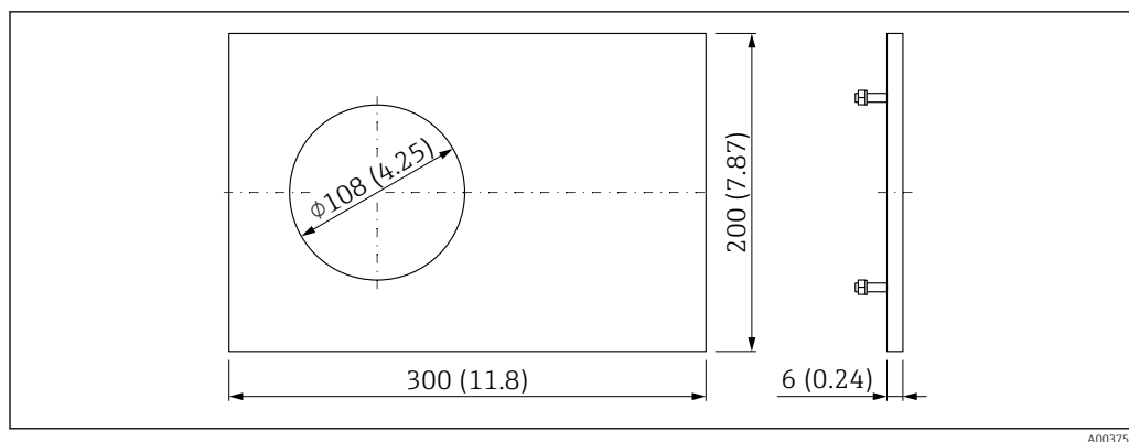
30 Перегородка (1.4301), вырез для датчика \varnothing 108 мм (4,25 дюйм). Единица измерения мм (дюйм)
