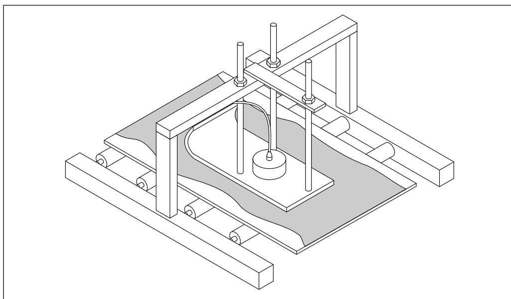
12 Пример монтажа скользящей каретки
