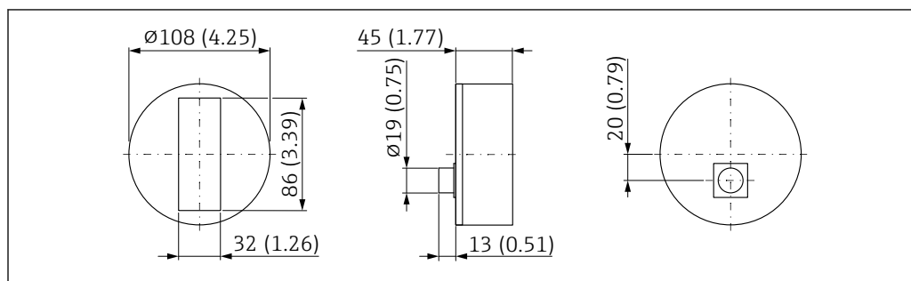
17 Размеры укороченного круглого датчика. Единица измерения мм (дюйм)
