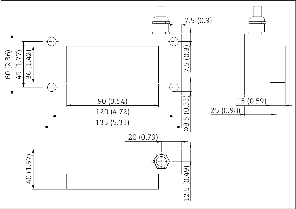
8 Dimensions. Unité de mesure mm (in)
