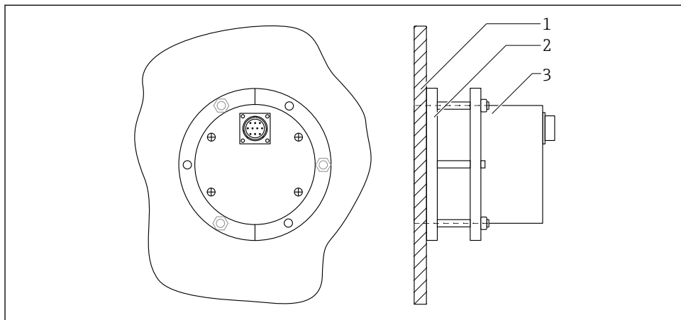
6 Capteur rond monté, version longue, vue arrière
