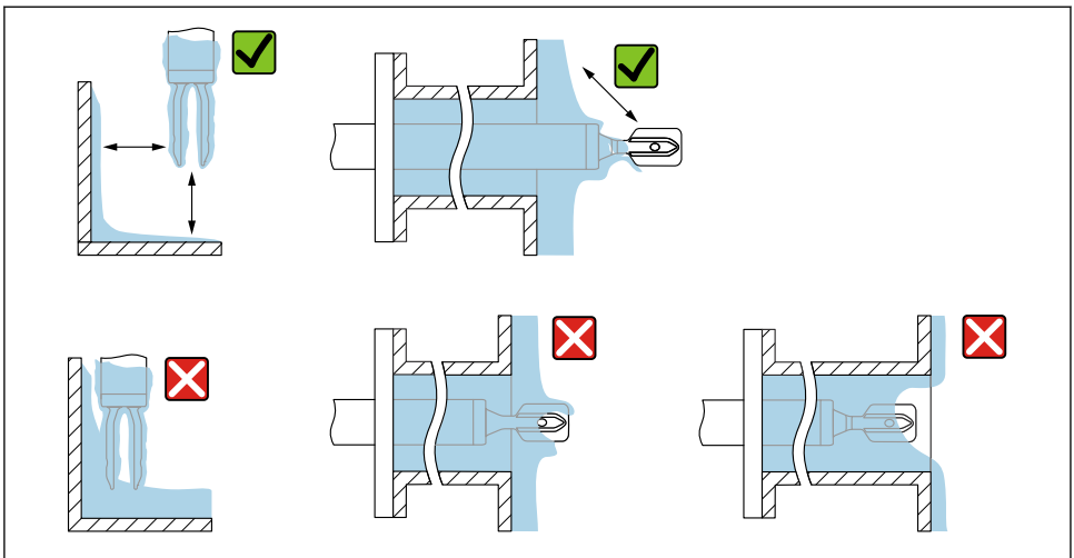
5 Einbaubeispiele für hochviskoses Prozessmedium
