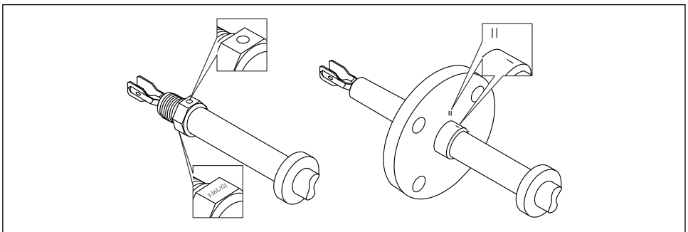
8 Stellung der Schwinggabel bei horizontalem Einbau im Behälter mithilfe der Markierung
