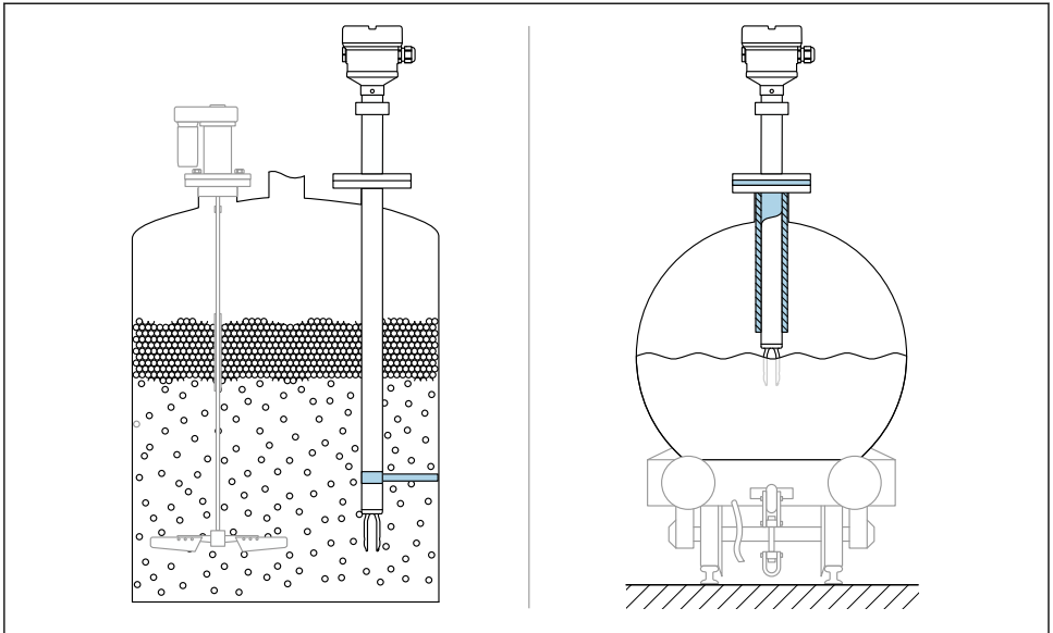
7 Beispiele für Abstützung bei dynamischer Belastung
