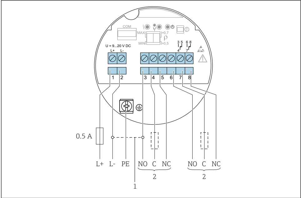
20 Gleichstromanschluss mit Relaisausgang, Elektronikeinsatz FEL64 DC
