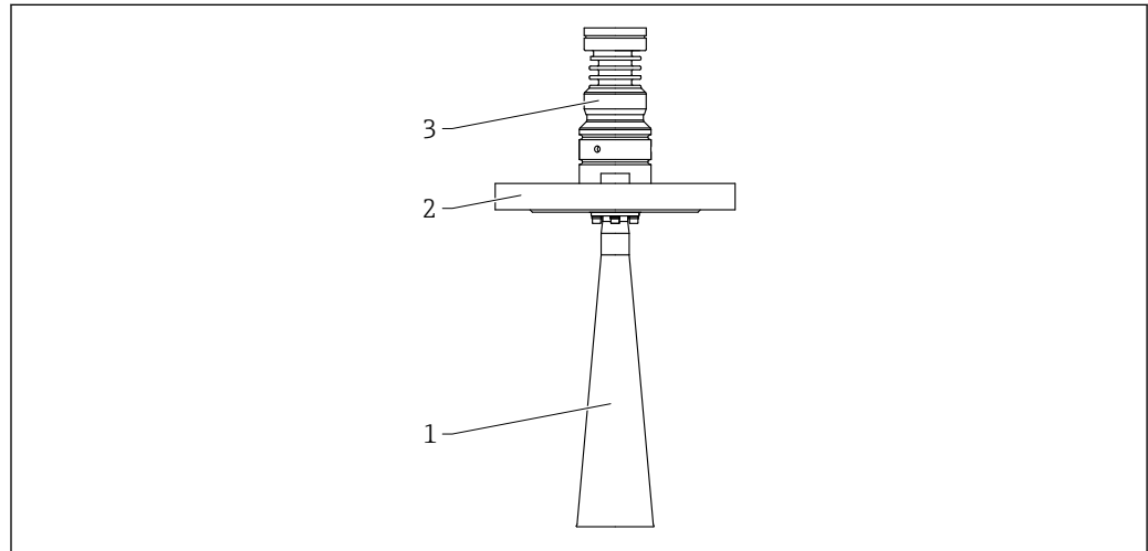
59 Material; DN65 Hornantenne. Maßeinheit mm (in)
