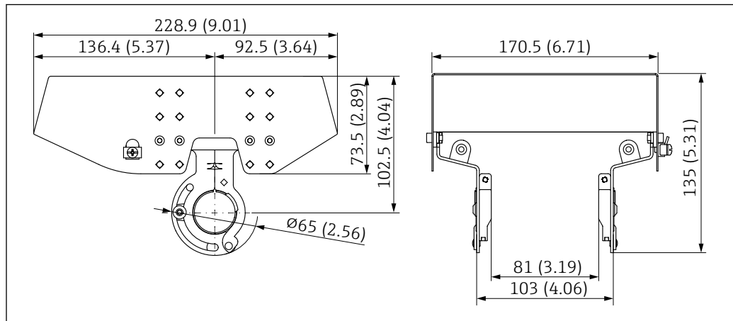
67 Abmessungen. Maßeinheit mm (in)
