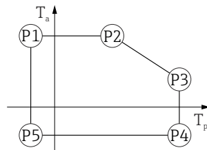
■ 22 Gehäuse Aluminium, beschichtet; Prozesstemperatur -40 \dots +80 \text{ °C} ( -40 \dots +176 \text{ °F} )
