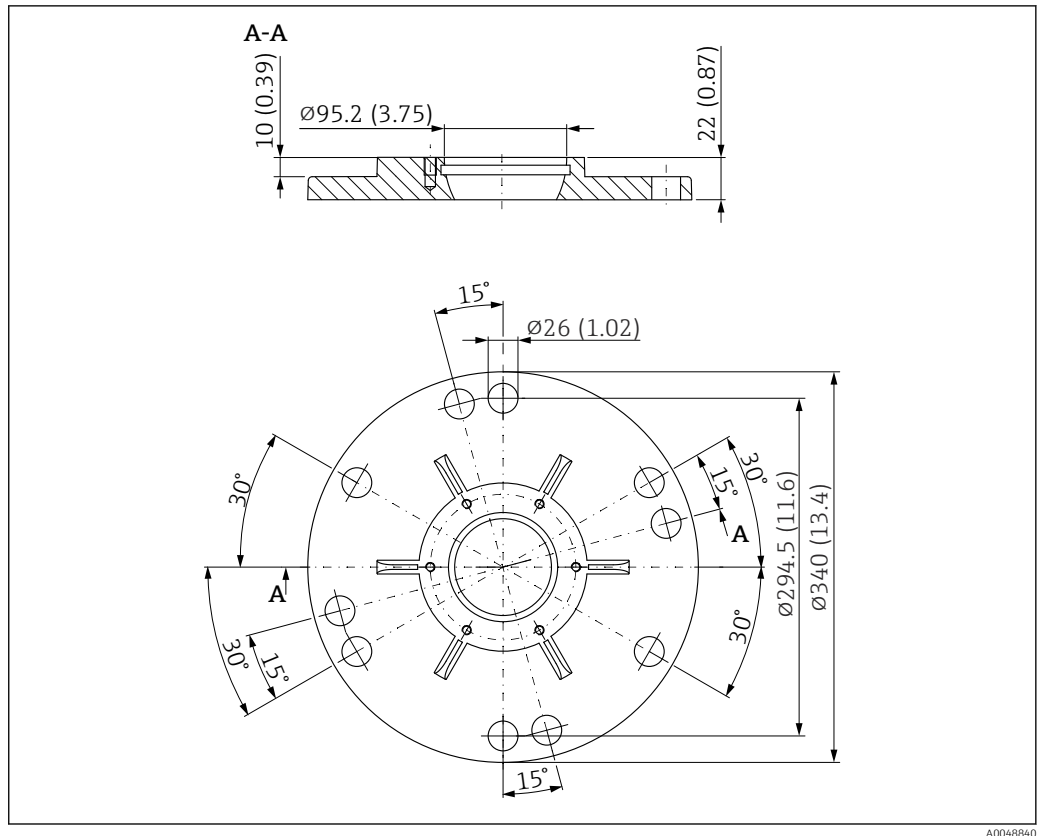
57 Abmessungen UNI Flansch 8"/DN200/200A für Antennen mit Ausrichtvorrichtung. Maßeinheit mm (in)
