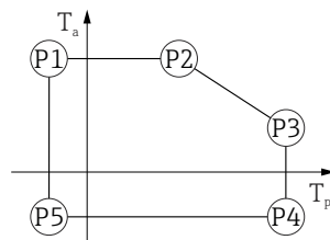
■ 23 Gehäuse Aluminium, beschichtet; Prozesstemperatur -40 \dots +150 \text{ °C} ( -40 \dots +302 \text{ °F} )
