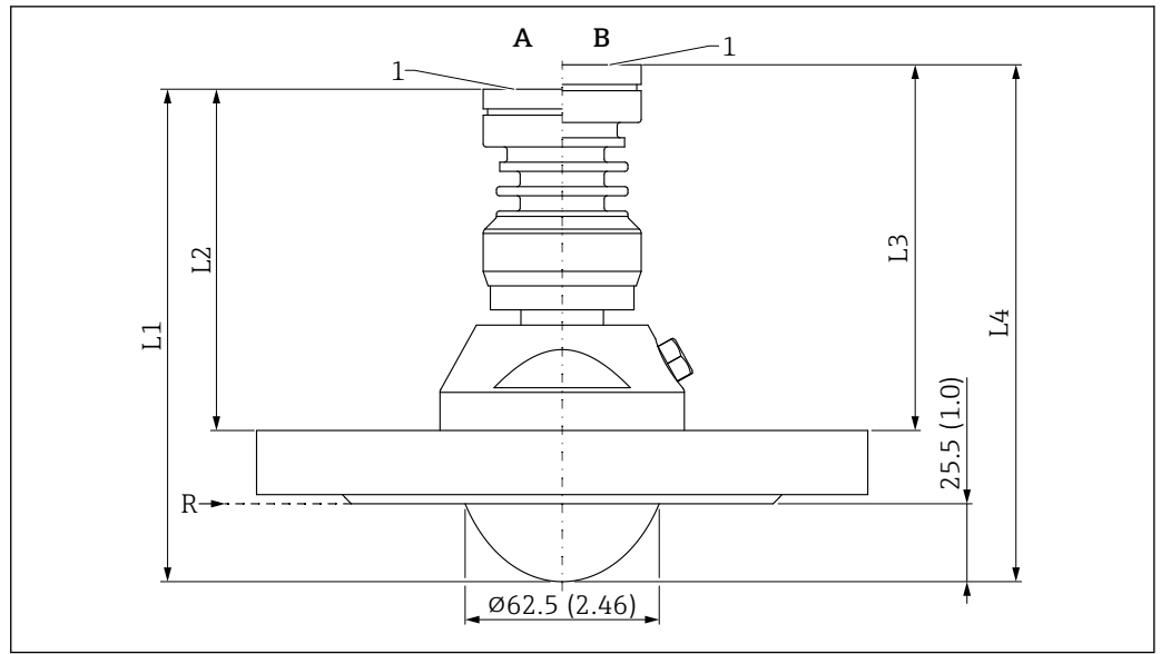
50 Abmessungen Antenne frontbündig, PTFE, 80 mm (3 in), mit Norm-Flansch und Spülluftanschluss . Maßeinheit mm (in)
