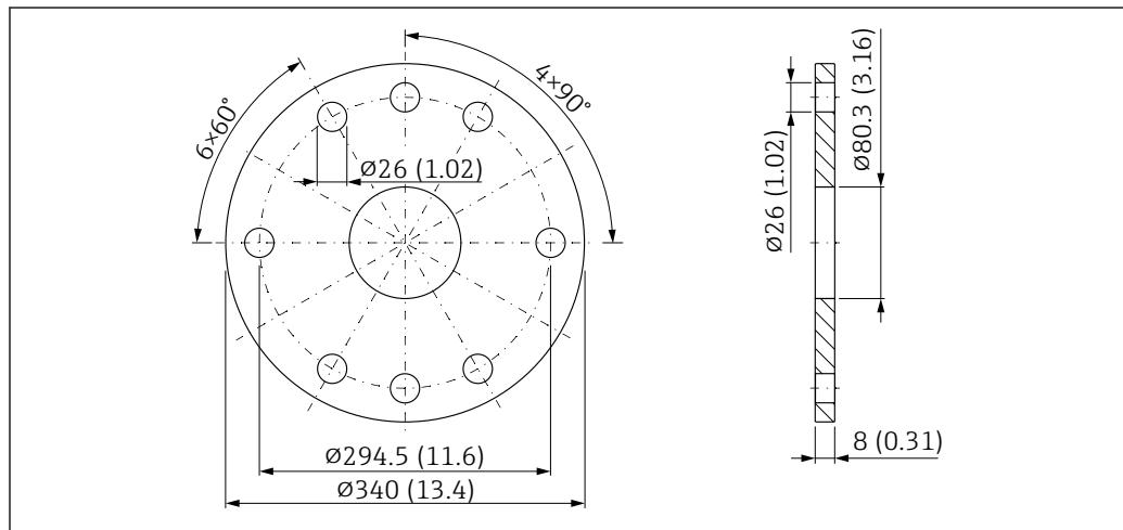
52 Abmessungen UNI-Flansch 8"/DN200/200A für DN80 Antenne mit Spülluftanschluss. Maßeinheit mm (in)
