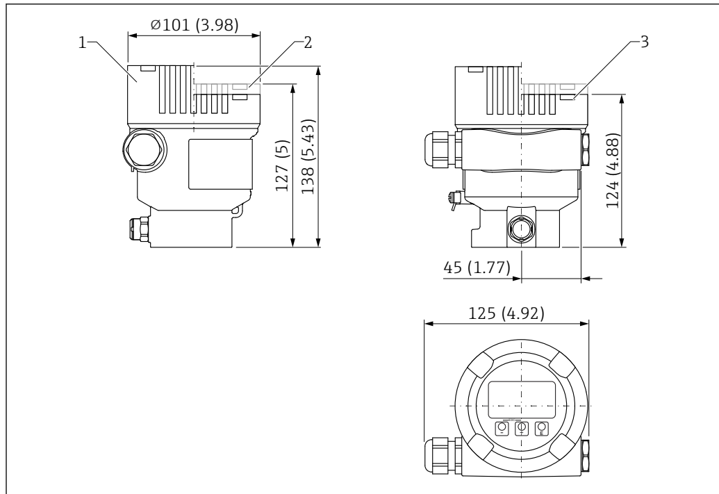
36 Abmessungen Einkammer Gehäuse Aluminium. Maßeinheit mm (in)
