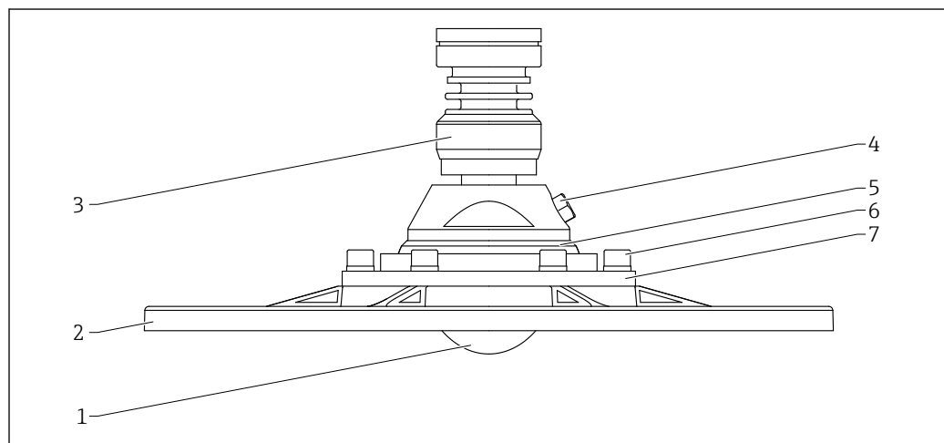
64 Material, Antenne frontbündig, 80 mm (3 in), mit UNI-Flansch, Ausrichtvorrichtung und Spülluftanschluss
