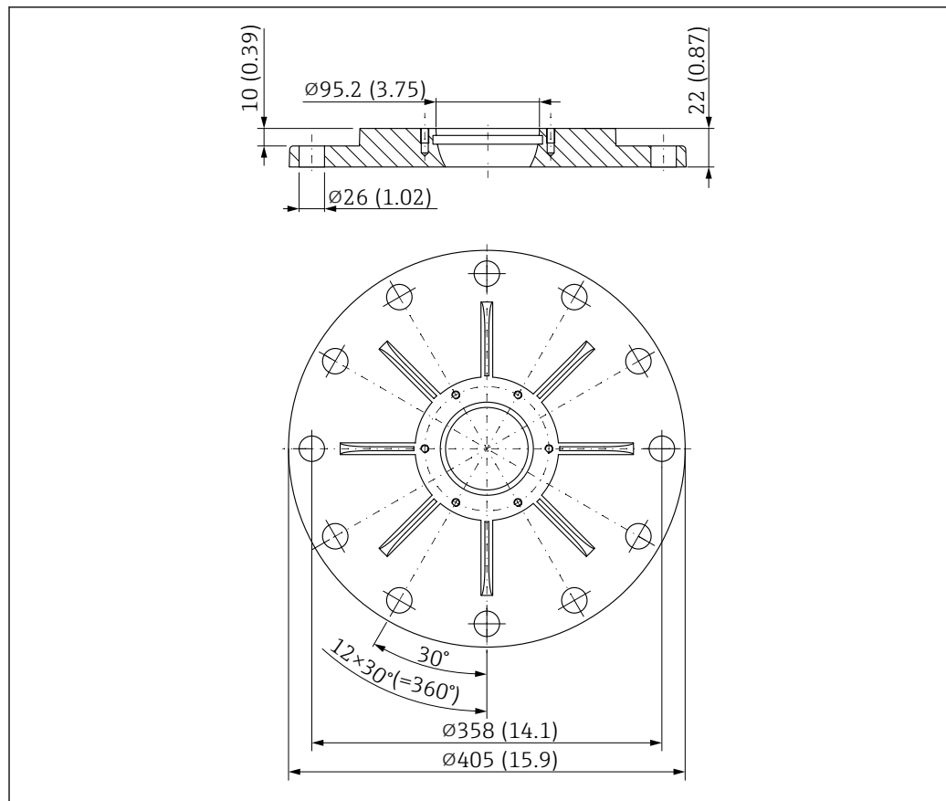
58 Abmessungen UNI Flansch 10"/DN250/250A für Antennen mit Ausrichtvorrichtung. Maßeinheit mm (in)
