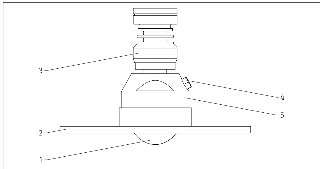
63 Material; Antenne frontbündig, 80 mm (3 in), mit UNI-Flansch und Spülluftanschluss. Maßeinheit mm (in)
