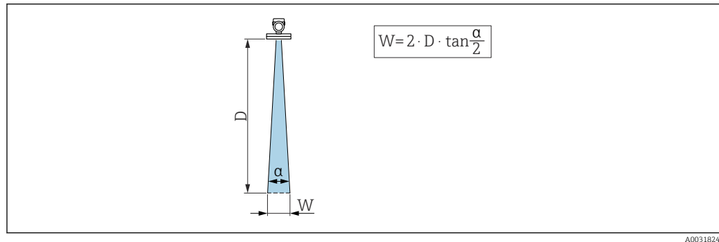
11 Zusammenhang zwischen Abstrahlwinkel \alpha , Distanz D und Kegelweite W
