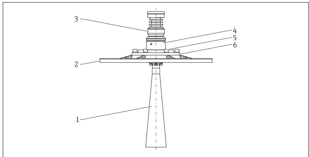
60 Material; DN65 Hornantenne, mit UNI-Flansch und Ausrichtvorrichtung. Maßeinheit mm (in)
