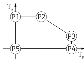
17 Kunststoffgehäuse; Prozesstemperatur 0 \dots +200 \text{ °C} ( +32 \dots +392 \text{ °F} ) bei CSA C/US Zulassung
