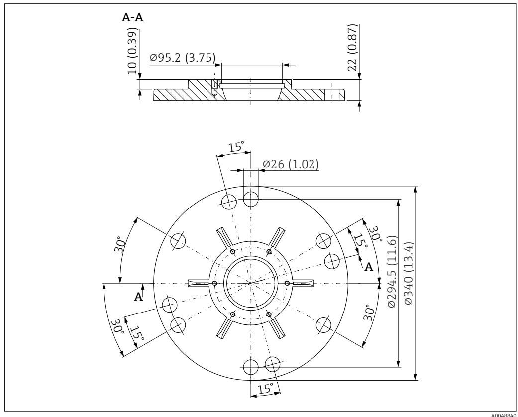
44 Abmessungen UNI Flansch 8"/DN200/200A für Antennen mit Ausrichtvorrichtung. Maßeinheit mm (in)
