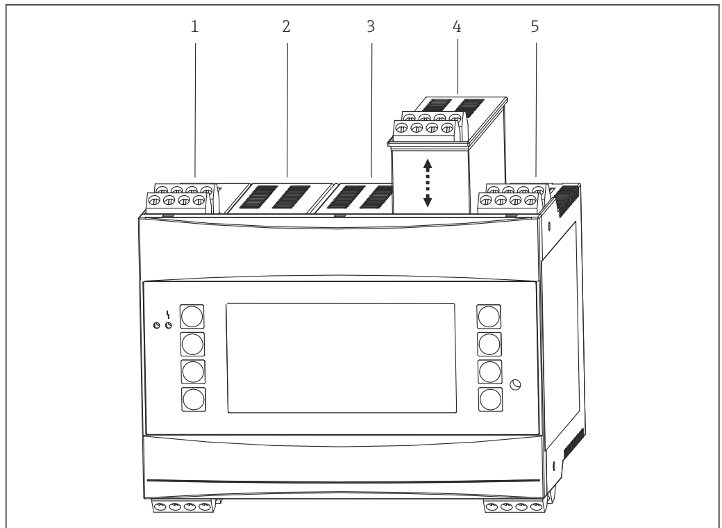
49 Gerät mit zusätzlichen Erweiterungskarten
