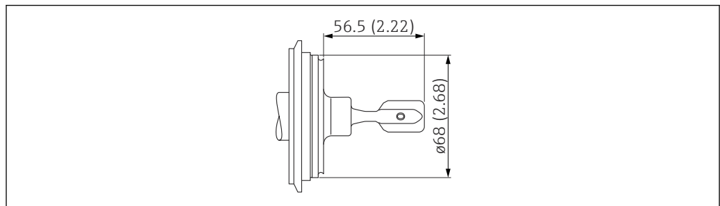
45 Varivent N Rohr DN65-162 PN25. Maßeinheit mm (in)
