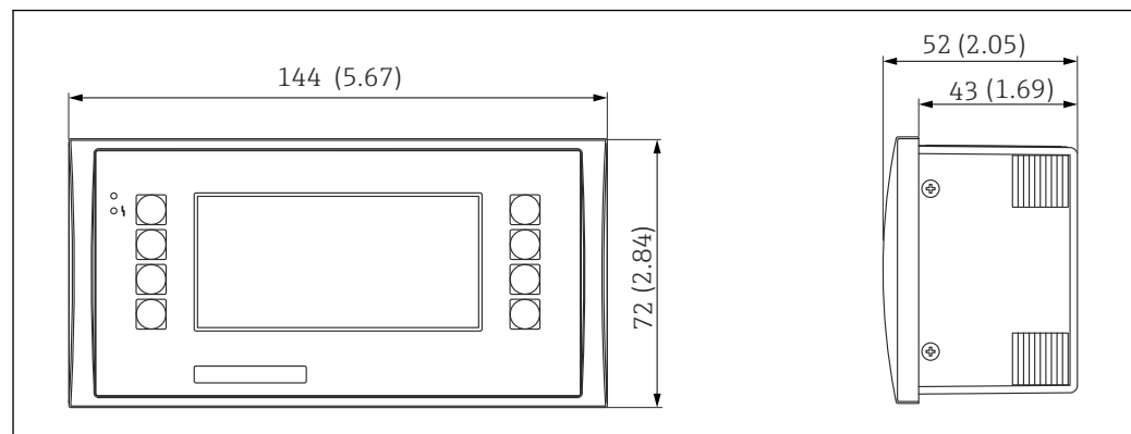
50 Bedien- und Anzeigeeinheit für Schalttafeleinbau. Maßeinheit mm (in)
