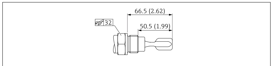
37 Gewinde ISO228 G 3/4. Maßeinheit mm (in)
