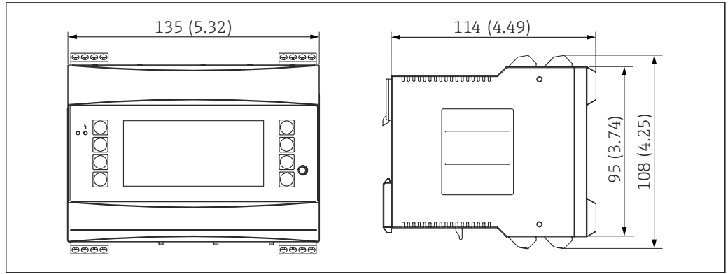
48 Gehäuse für Hutschiene nach IEC 60715. Maßeinheit mm (in)
