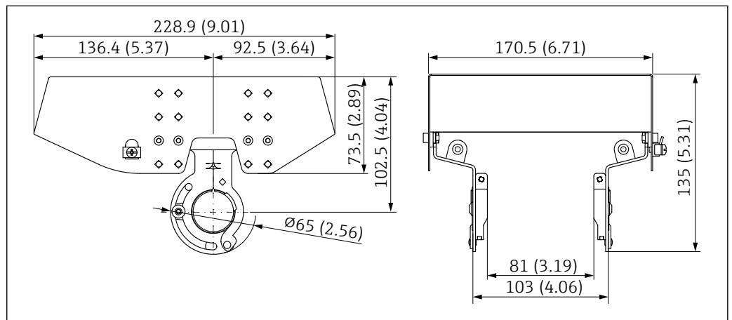
52 Wetterschutzhaube für Zweikammer Gehäuse Aluminium. Maßeinheit mm (in)
