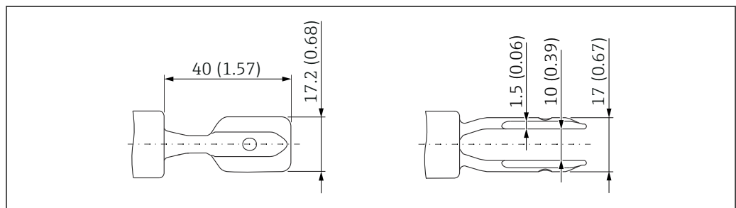
35 Schwinggabel. Maßeinheit mm (in)
