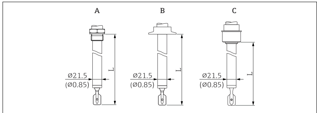
34 Sondenbauarten: Rohrverlängerung, Kurzrohrversion (Sensorlänge L). Maßeinheit mm (in)
