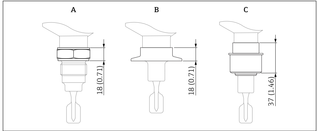
36 Maximale Angabe der Höhe der Prozessanschlüsse. Maßeinheit mm (in)
