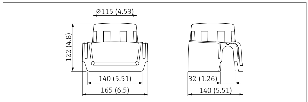
53 Wetterschutzhaube für Einkammergehäuse Aluminium. Maßeinheit mm (in)
