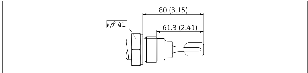
38 Gewinde ISO228 G 1. Maßeinheit mm (in)
