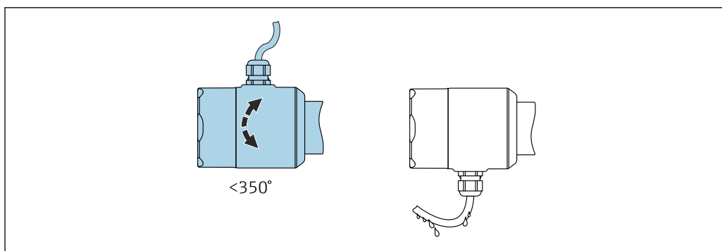
25 Gehäuse ohne Feststellschraube mit Abtropfschlaufe
