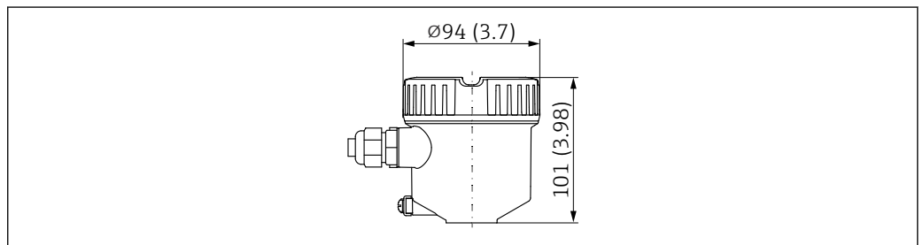
28 Abmessungen Einkammer Gehäuse Kunststoff; Deckel ohne Sichtscheibe. Maßeinheit mm (in)
