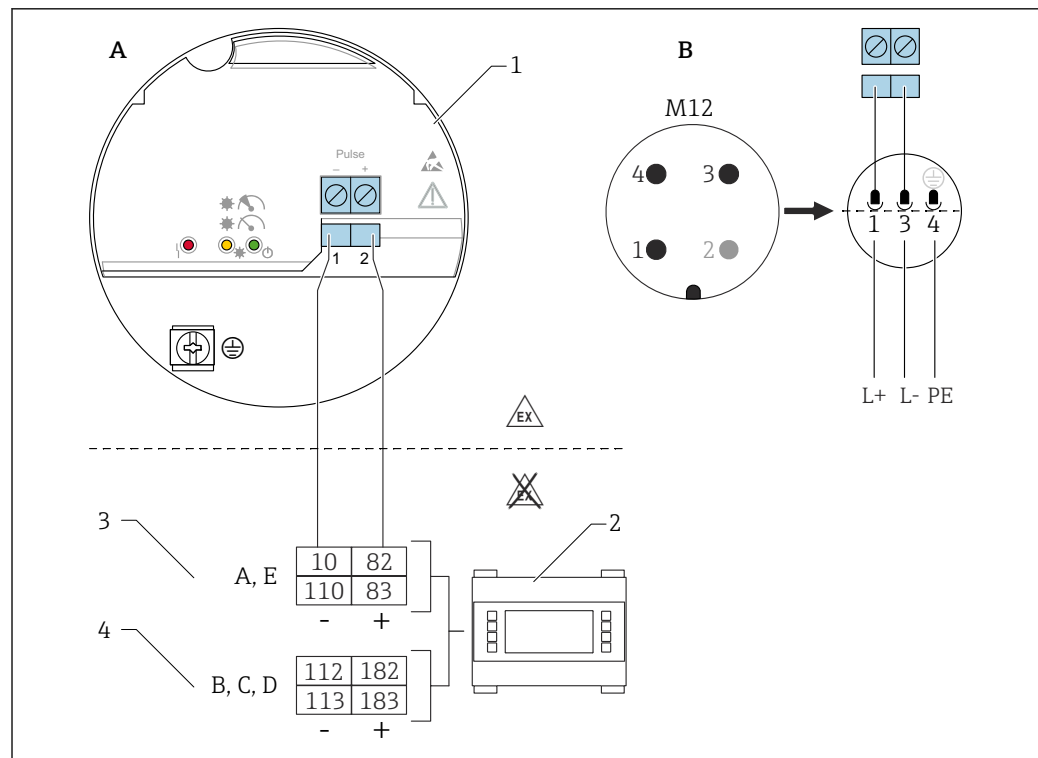
14 Anschlussschema: Anschluss Elektronikeinsatz FEL60D an den Dichterechner FML621
