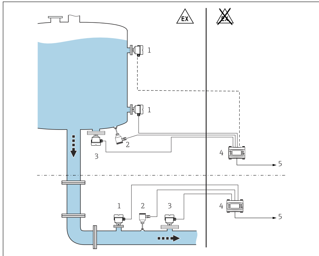
15 Dichtemessung mit Dichterechner FML621
