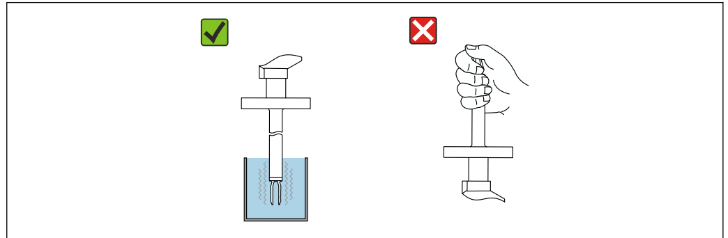
18 Funktionstest der Schwinggabel
