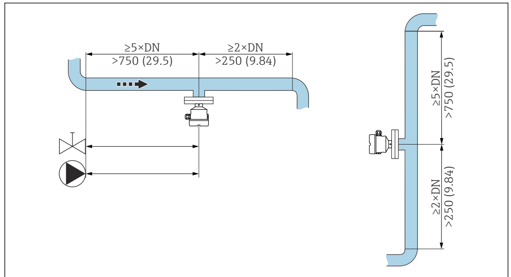
6 Installation Einlaufstrecke. Maßeinheit mm (in)
