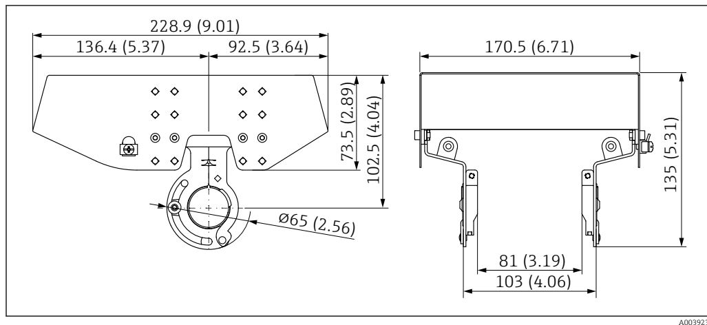
19 Wetterschutzhaube für Zweikammer Gehäuse Aluminium. Maßeinheit mm (in)
