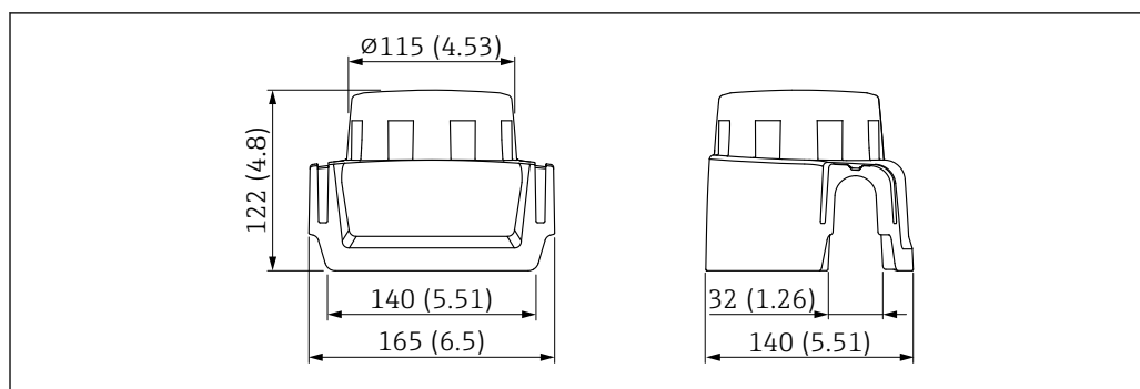
20 Wetterschutzhaube für Einkammer Gehäuse Aluminium oder 316L. Maßeinheit mm (in)
