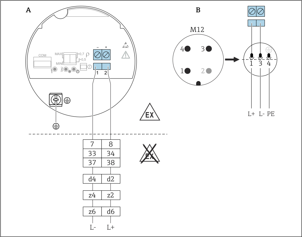
图 25 电子插件 FEL67: PFM 输出
