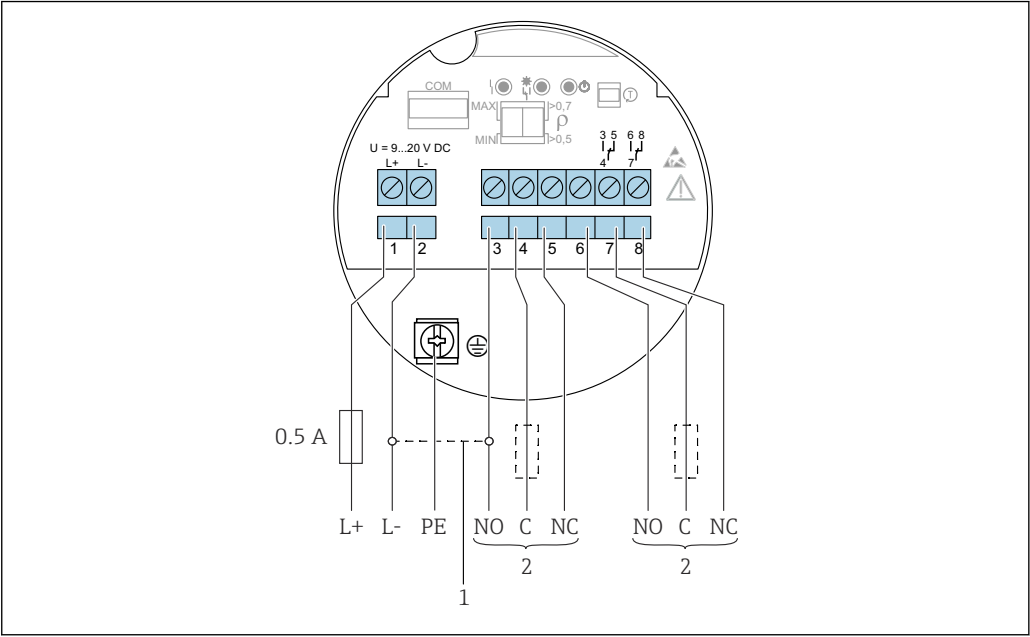
23 电子插件 FEL64 DC: 直流连接型, 带继电器输出
