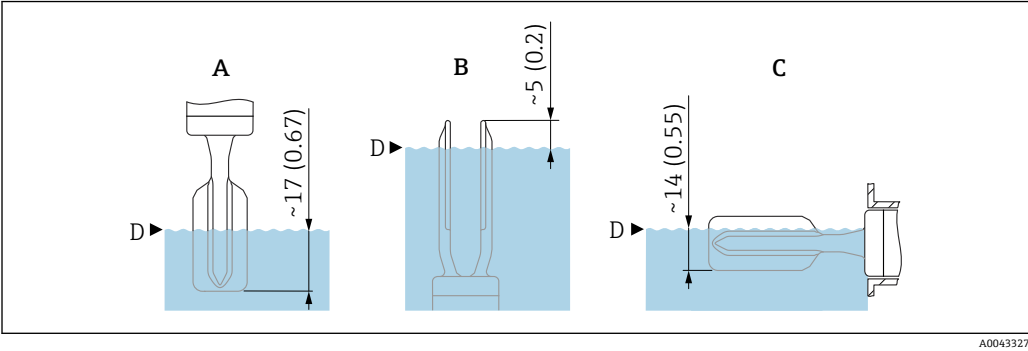
图 6 搪瓷涂层叉体的常见开关点。测量单位 mm (in)
