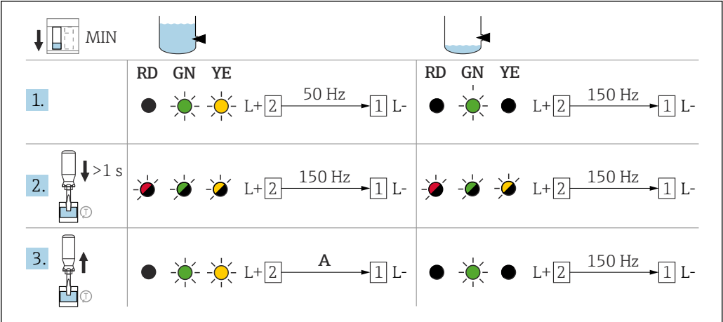
40 FEL67 在低限 (MIN) 检测模式下的继电器响应和故障报警信号
