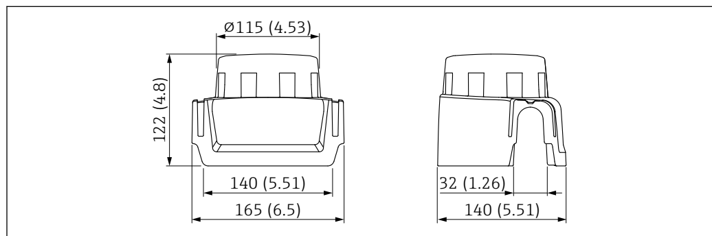
■ 46 保护盖，适用单腔体铝外壳或 316L 外壳。测量单位 mm (in)
