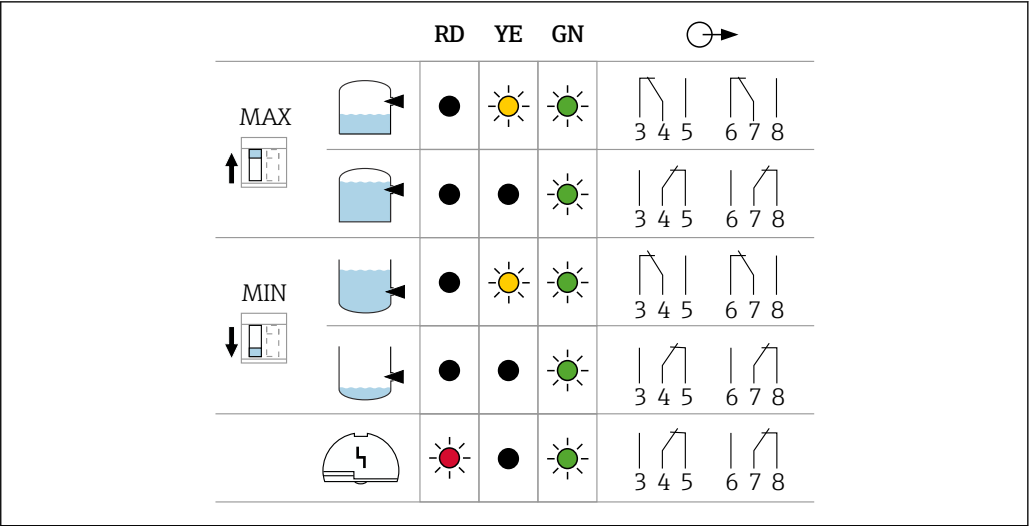
22 电子插件 FEL64 的继电器响应和故障信号
