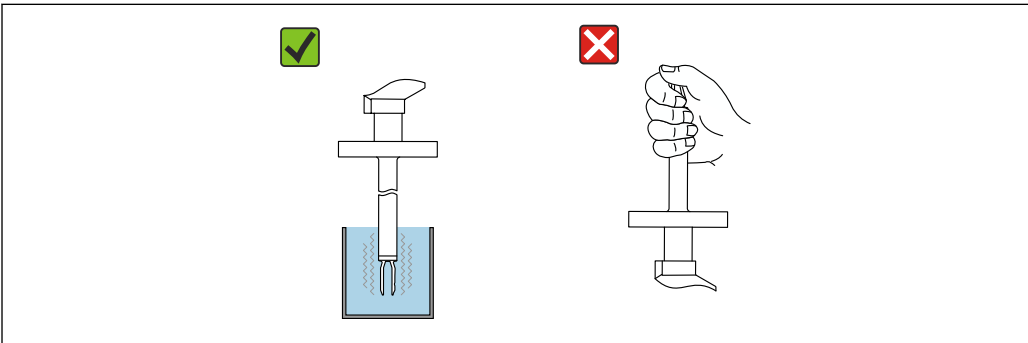
34 音叉的功能测试
