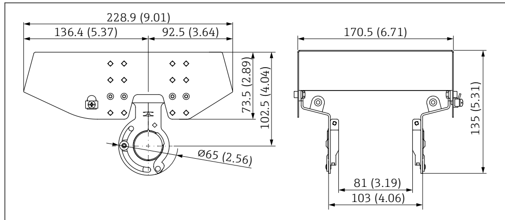
■ 45 双腔体铝外壳的防护罩。测量单位 mm (in)
