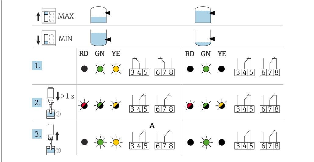
图 38 FEL64、FEL64DC 的继电器响应和故障报警信号
