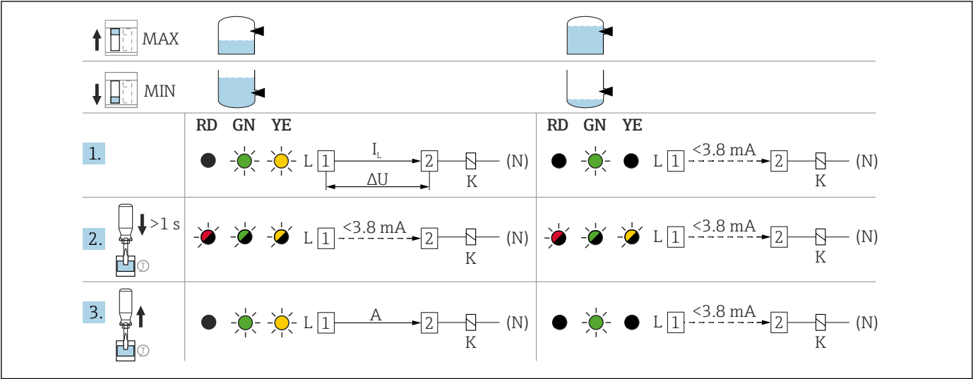
36 FEL61 的继电器响应和故障报警信号
