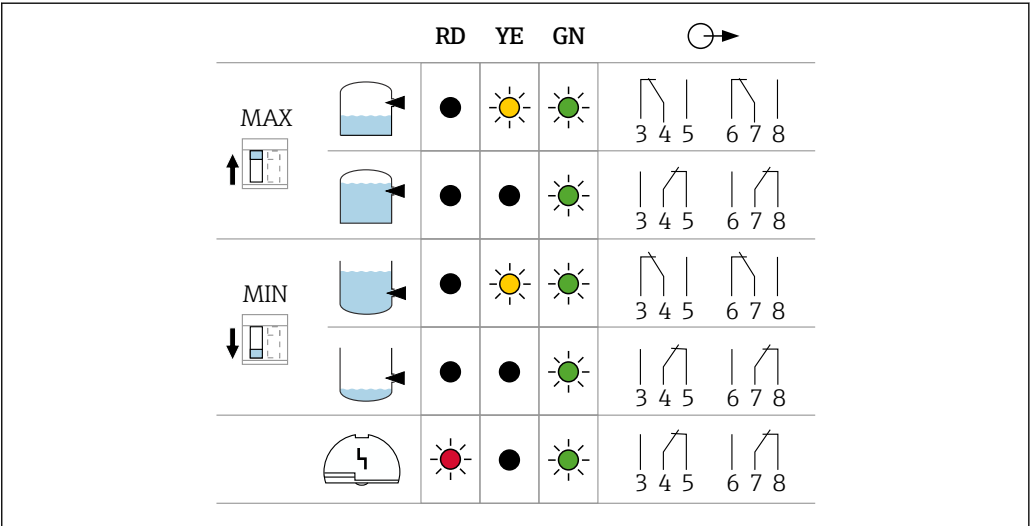
24 电子插件 FEL64 DC 的继电器响应和故障信号
