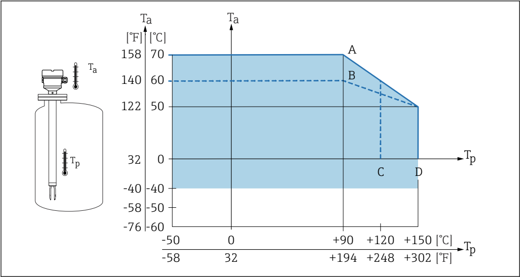
图 49 外壳允许环境温度 T_a 与罐体内部过程温度 T_p 的关系:
