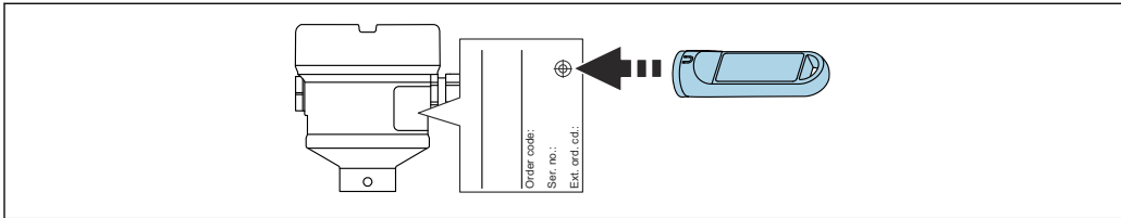
图 42 使用测试磁铁进行功能测试
