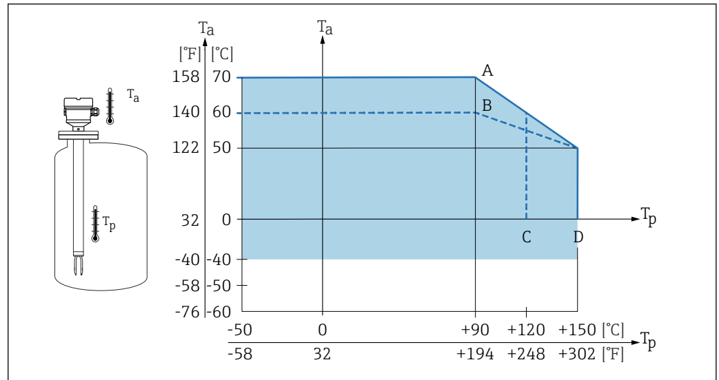
49 Temperatura ambiente ammissibile T_a nella custodia in funzione della temperatura di processo T_p nel recipiente:
