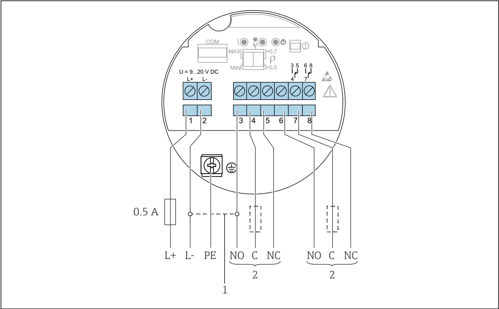
23 Collegamento c.c. con uscita a relè, inserto elettronico FEL64 DC
