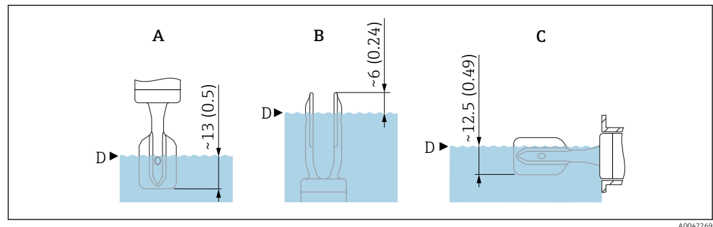
5 Punti di commutazione tipici, diapason rivestito in plastica (ECTFE, PFA). Unità di misura mm (in)
