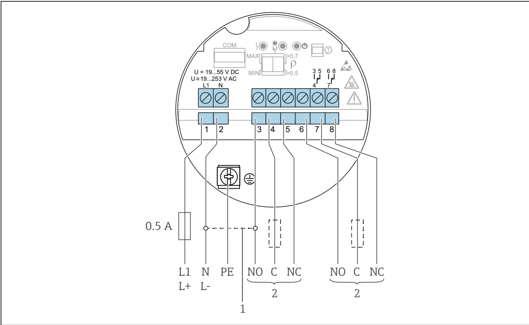
21 Connessione di corrente universale con uscita a relè, inserto elettronico FEL64
