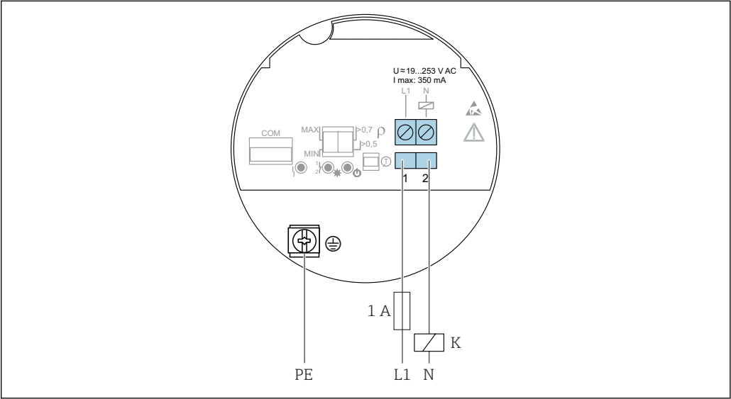
16 Bifilare c.a., inserto elettronico FEL61
