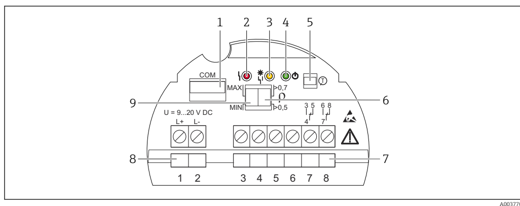
Fig. 32 Esempio di inserto elettronico FEL64DC
