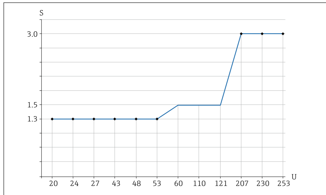
18 Potenza di mantenimento/potenza nominale minima consigliata in base al carico
