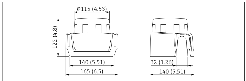
46 Coperchio di protezione per custodia a vano unico, alluminio o 316L. Unità di misura mm (in)
