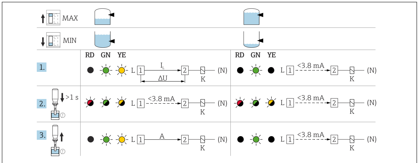
36 FEL61 - Comportamento di commutazione e segnalazione
