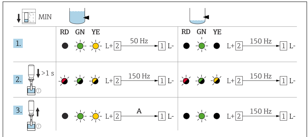
40 Comportamento di commutazione di MIN e segnalazione con FEL67
