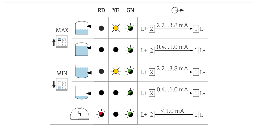
28 Azione dell'uscita di commutazione e segnalazione, inserto elettronico FEL68
