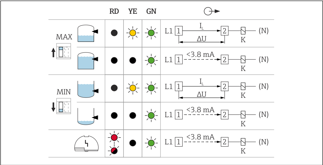
17 Azione dell'uscita di commutazione e segnalazione, inserto elettronico FEL61
