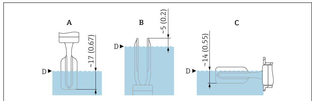
6 Punti di commutazione tipici, diapason smaltato. Unità di misura mm (in)
