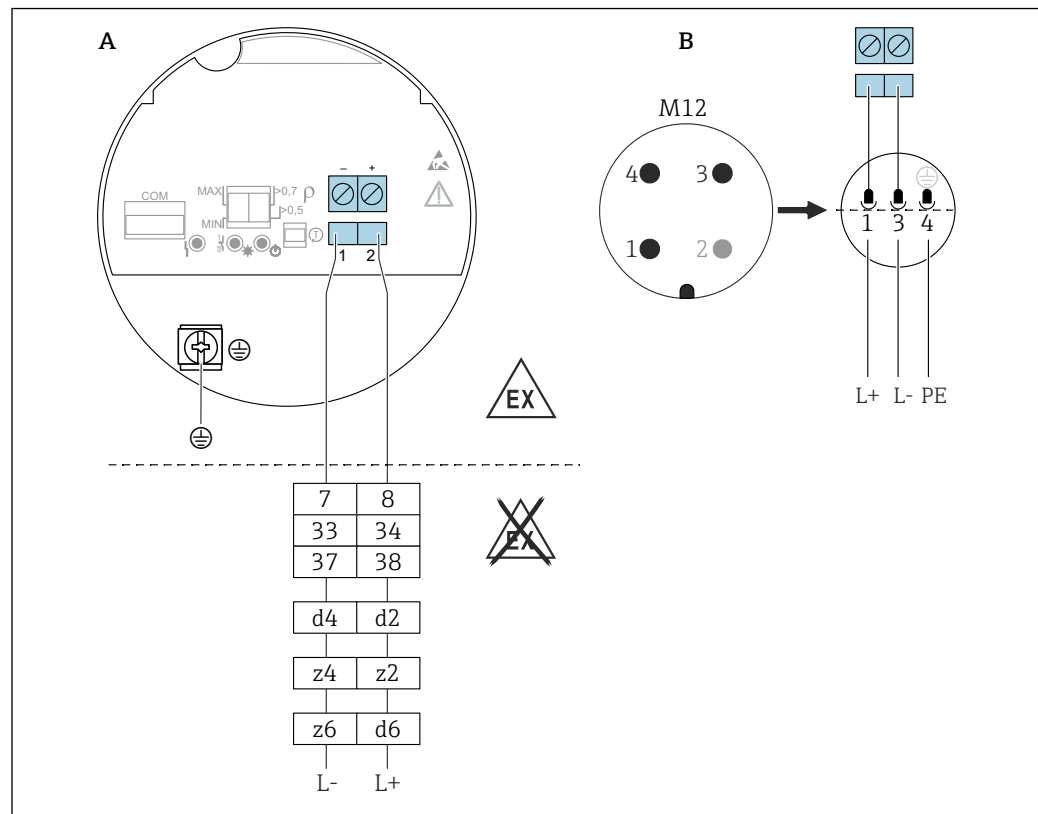
25 Uscita PFM, inserto elettronico FEL67
