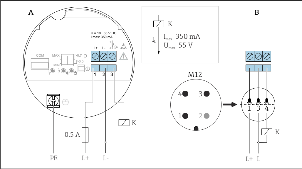
19 PNP c.c. trifilare, inserto elettronico FEL62 A Collegamento dei fili ai morsetti B Collegamento dei fili con connettore M12 nella custodia, secondo la norma EN61131-2
