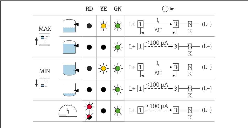
20 Azione dell'uscita di commutazione e segnalazione, inserto elettronico FEL62 MAX DIP switch per impostazione della modalità di sicurezza MAX MIN DIP switch per impostazione della modalità di sicurezza MIN RD LED rosso per avvertenza o allarme YE LED giallo, stato di commutazione GN LED verde per indicazione dello stato operativo, dispositivo in funzione I_L Carico di corrente di commutazione
