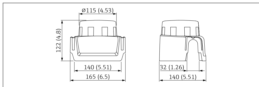
22 Coperchio di protezione per custodia a vano unico, alluminio o 316L. Unità di misura mm (in)
