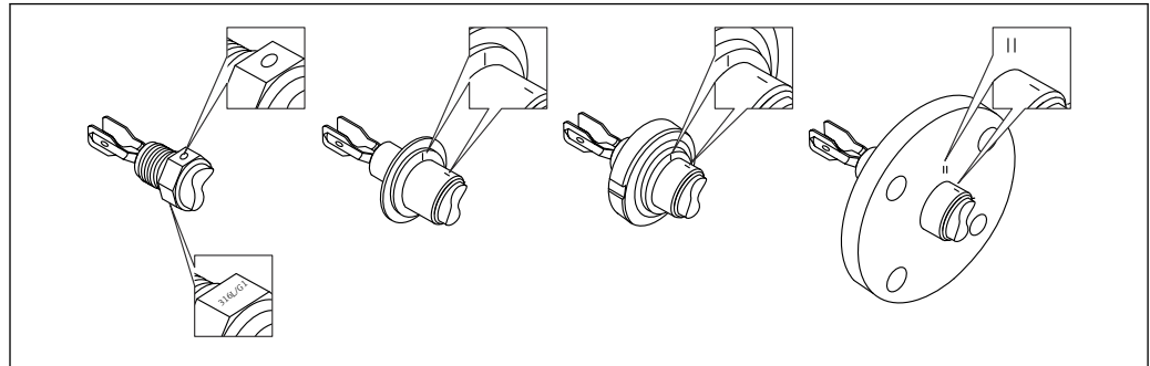
12 Posizione del diapason quando installato orizzontalmente nel silo utilizzando il contrassegno
