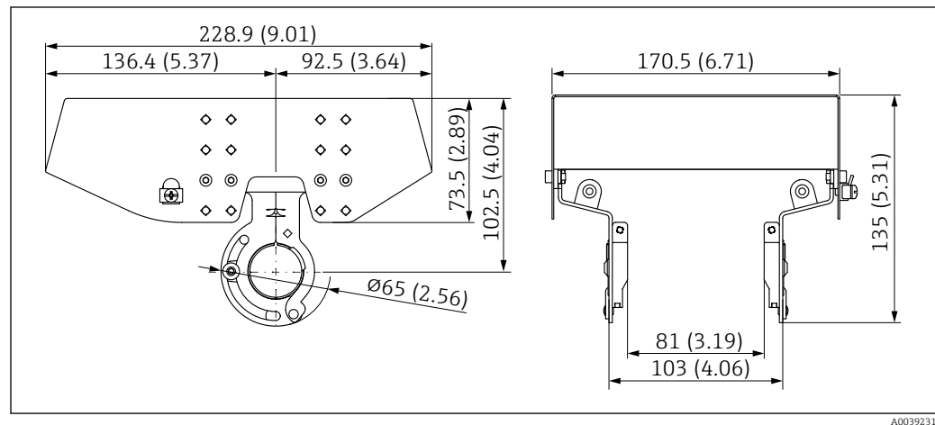
21 Coperchio di protezione per custodia a doppio vano in alluminio. Unità di misura mm (in)
