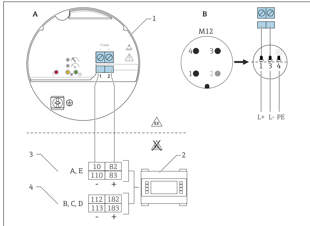
17 Schema di connessione: connessione dell'inserto elettronico FEL60D all'elaboratore di densità FML621
