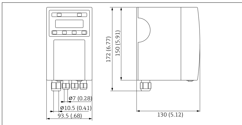
9 Dimensioni della pompa. Unità di misura mm (in)
