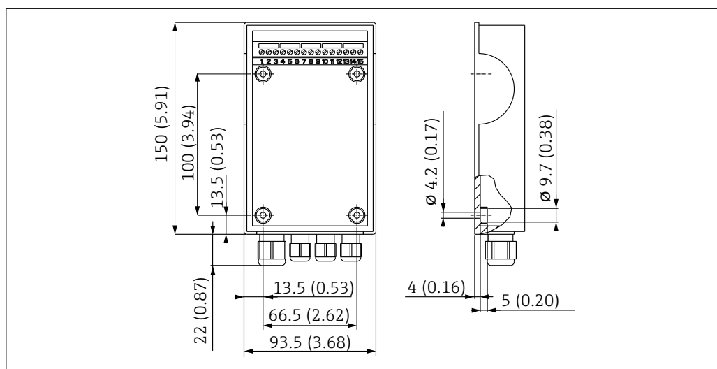
10 Dimensioni per foratura piastra per supporto a parete
