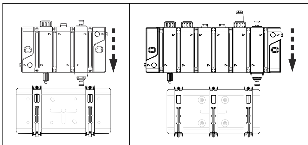
4 2 fermagli di fissaggio per 1 ... 5 moduli
