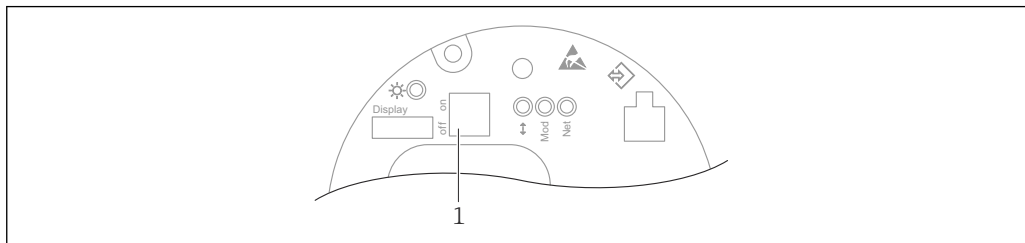
1 Mikroprzełącznik DIP do blokowania i odblokowania dostępu do ustawień przyrządu
