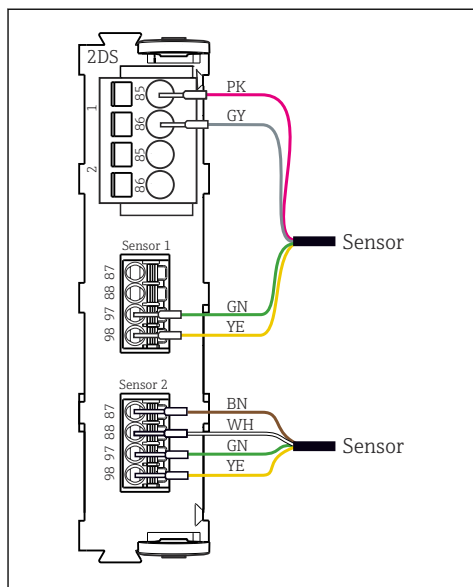
32 Sensorer med og uden ekstra forsyningsspænding ved sensormodul 2DS
