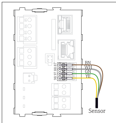
30 Memosens-sensorer uden ekstra forsyningsspænding
