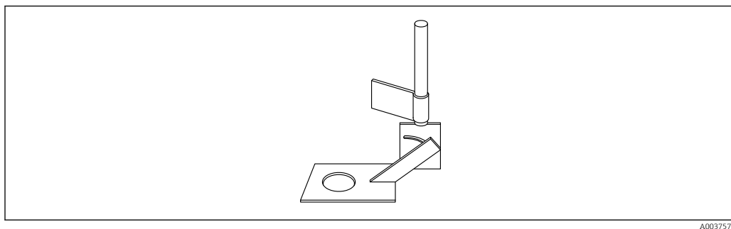
21 Suporte universal 1.4301 com mecanismo de inclinação e cabeça de retenção, corte do sensor \varnothing 108 mm (4.25 in)
