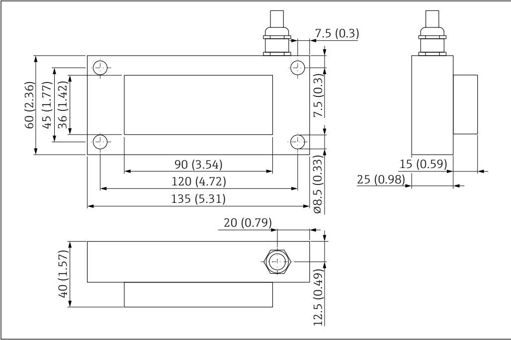
6 Dimensões. Unidade de medida mm (in)
