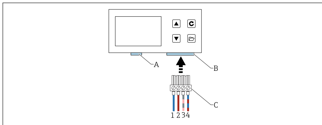
15 Conexão com um display remoto
