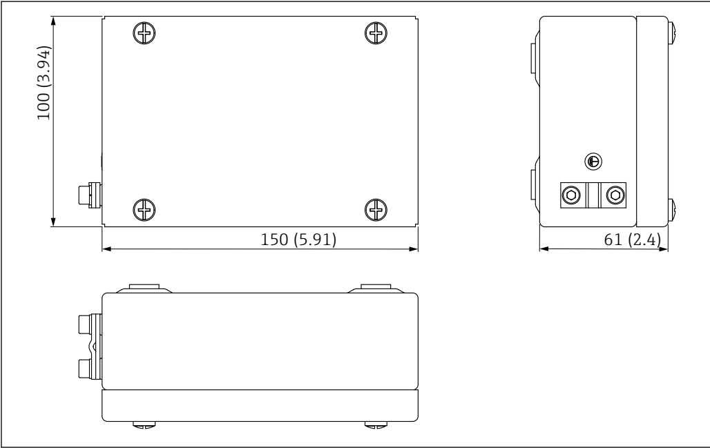
7 Dimensões do invólucro dos componentes eletrônicos ATEX. Unidade de medida mm (in)
