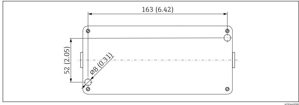
11 Gabarito de instalação para o invólucro com o módulo de eletrônica remoto. Unidade de medida mm (in)
