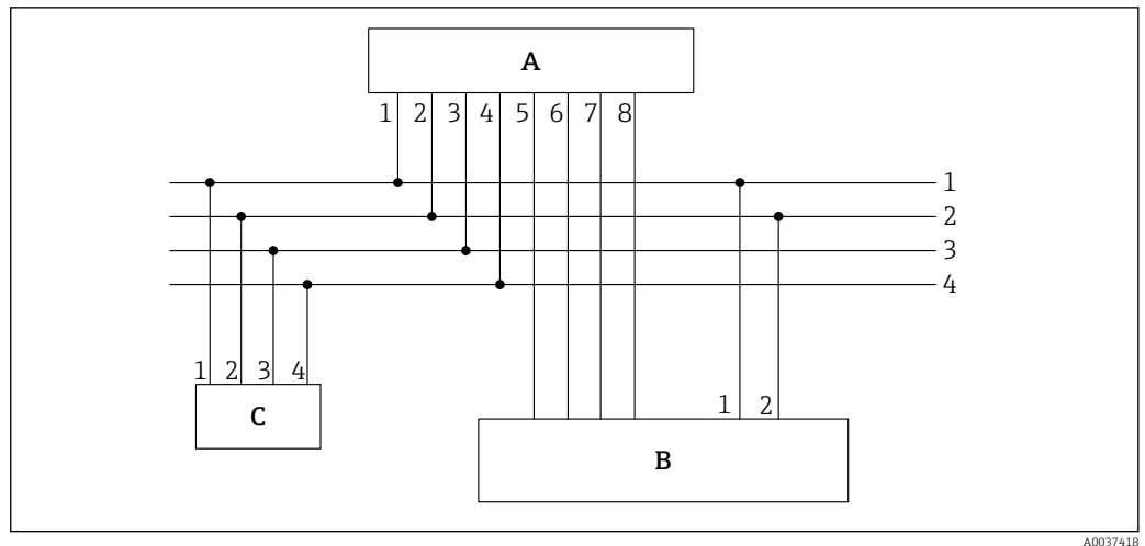
16 Exemplo de conexão, cabo com soquete de 10 pinos (no lado do equipamento) e arruelas na extremidade do cabo
