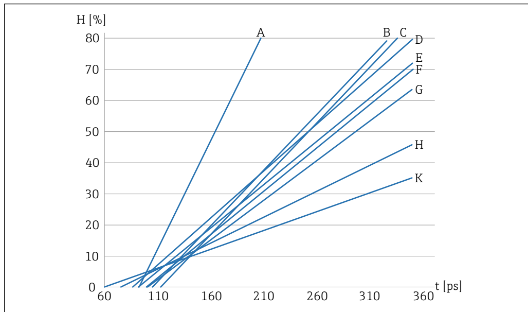
18 Conjunto de curvas de calibração B (Cal.A, Cal.B, Cal.C, Cal.D, Cal.E, Cal.F, Cal.G, Cal.H, Cal.K)
