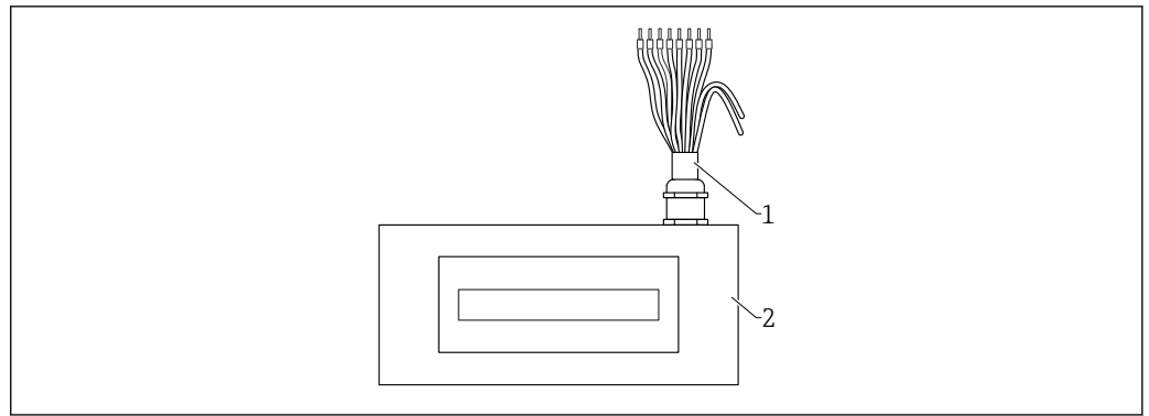
13 Sensor retangular (versão padrão) com atribuição de cabo de 10 pinos
