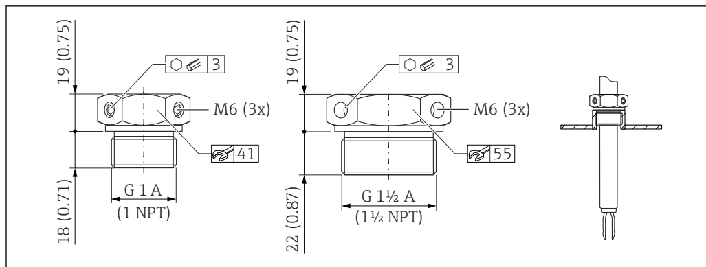
54 Manchons coulissants pour un fonctionnement sans pression p_e = 0 \text{ bar} (0 psi). Unité de mesure mm (in)
