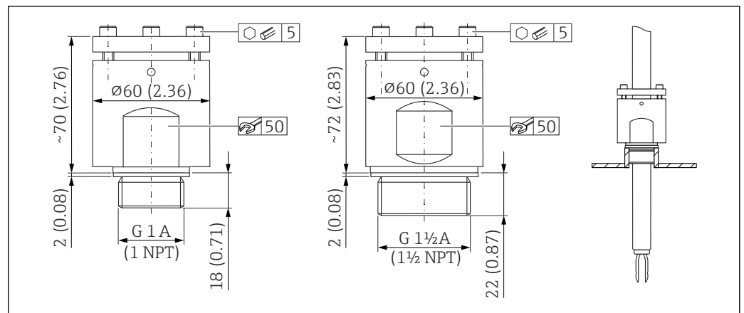
55 Manchons coulissants haute pression. Unité de mesure mm (in)
