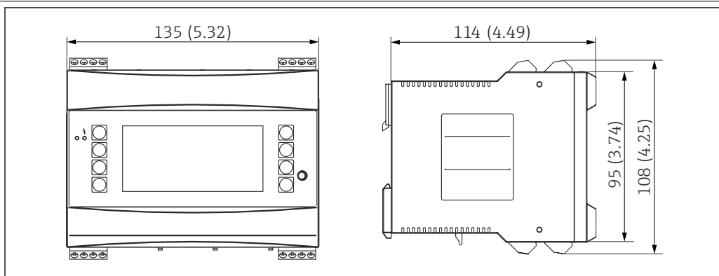
48 Boîtier pour rail DIN selon IEC 60715. Unité de mesure mm (in)
