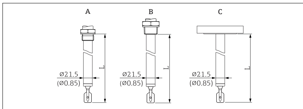
34 Constructions de sonde : tube prolongateur, version tube court (longueur L du capteur). Unité de mesure mm (in)
