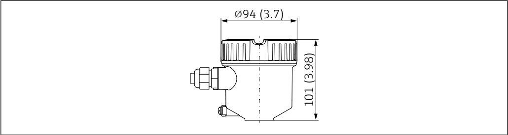
27 Dimensions du boîtier à simple compartiment, plastique ; couvercle sans fenêtre. Unité de mesure mm (in)
