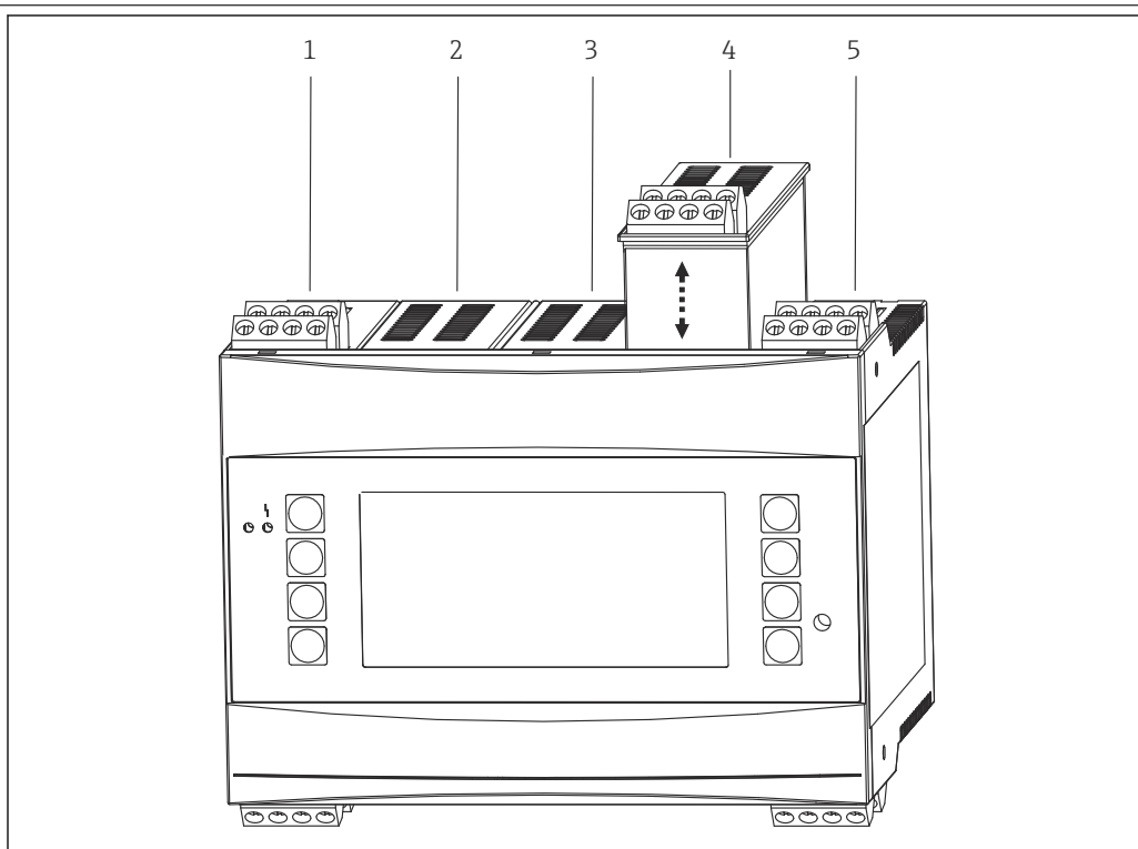
49 Appareil avec cartes d'extension supplémentaires
