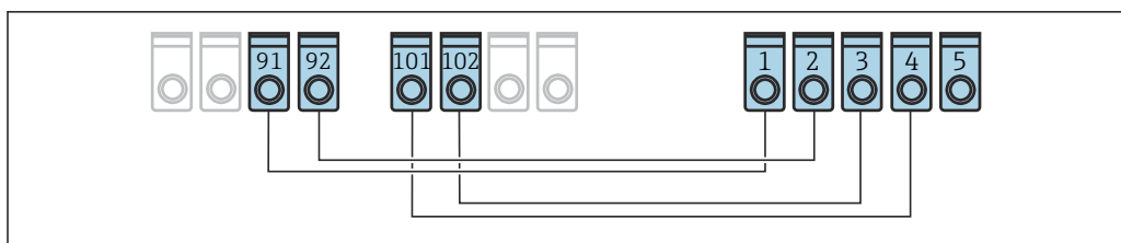
20 Connexions de fil entre l'afficheur séparé et l'unité de base.
