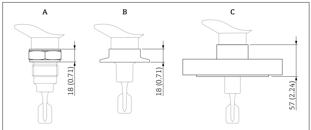
36 Spécification de hauteur maximale pour les raccords process. Unité de mesure mm (in)
