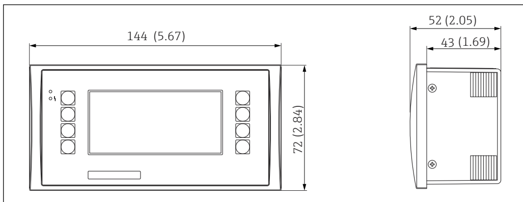
50 Unité d'affichage et de configuration pour montage en façade d'armoire. Unité de mesure mm (in)
