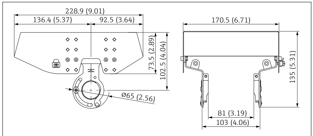
52 Capot de protection pour boîtier à double compartiment en aluminium. Unité de mesure mm (in)
