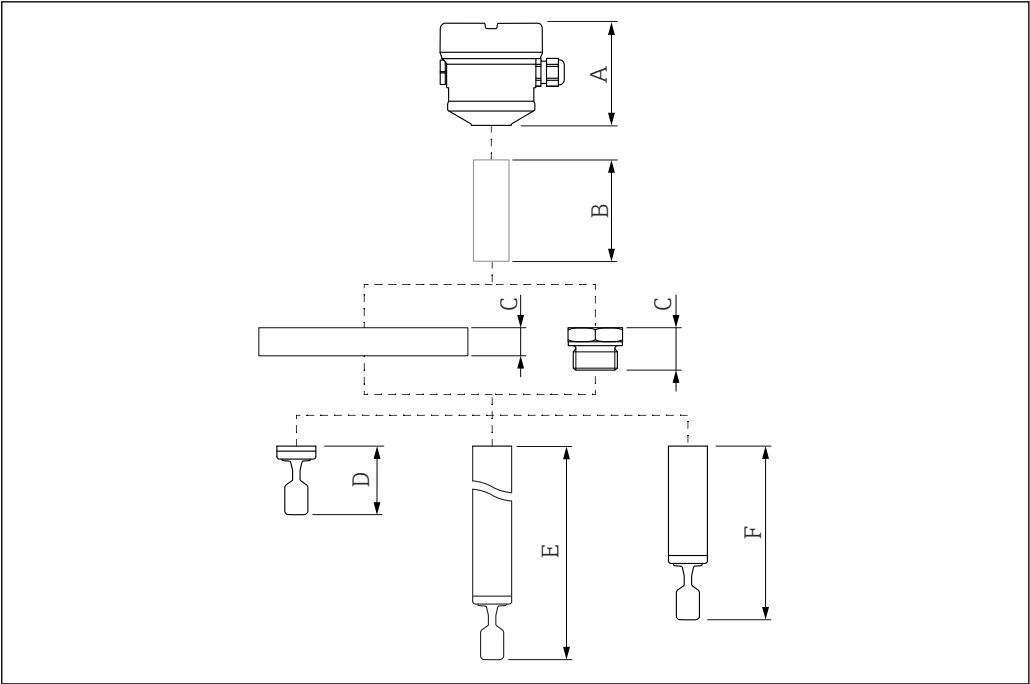
26 Composants permettant de déterminer la hauteur de l'appareil
