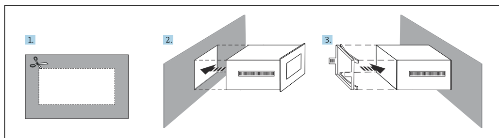
19 Montage de l'afficheur
