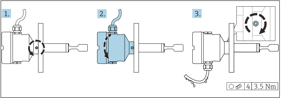
11 Harici kilit vidası ve damlama döngüsüne sahip muhafaza
