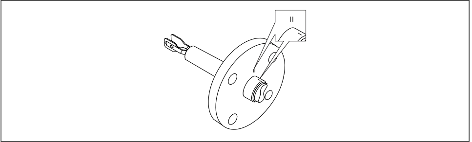
9 İşaretleme kullanılarak kanala yatay olarak monte edildiğinde ayar çatalının konumu
