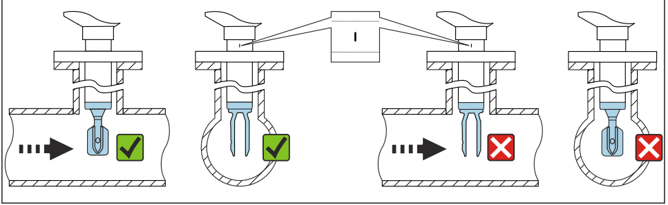
10 Boruya kurulum (çatal pozisyonunu ve işaretini dikkate alın)
