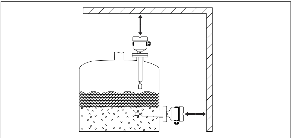
7 Luați în considerare distanța din afara rezervorului
