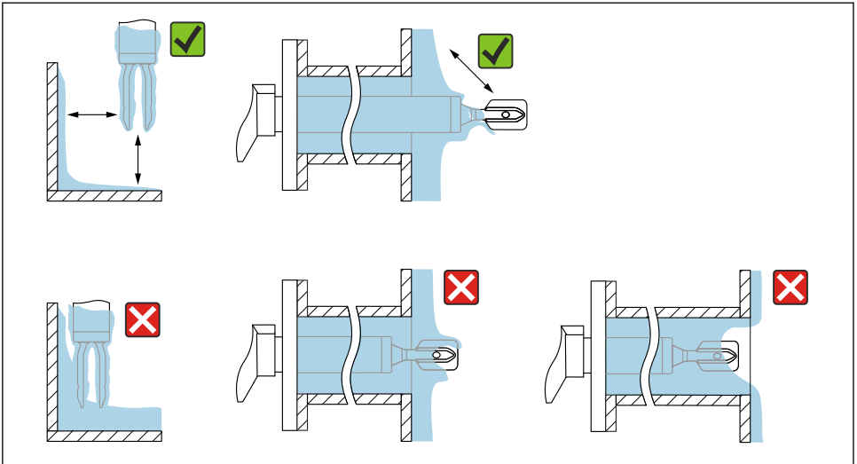
6 Exemple de instalare pentru un fluid de proces deosebit de vâcos
