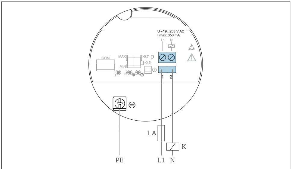
13 2 cabluri c.a., inserție electronică FEL61
