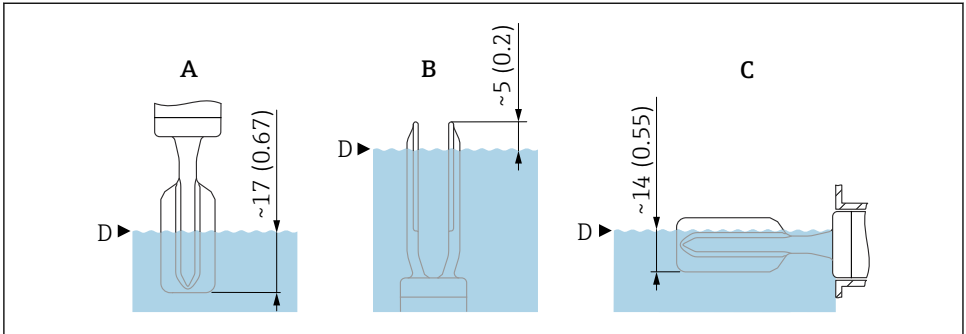
3 Points de détection typiques, fourche vibrante revêtue d'émail. Unité de mesure mm (in)
