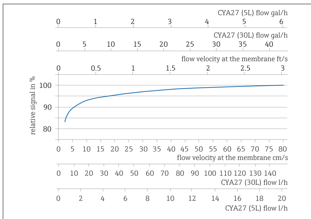
2 Sammenhæng mellem elektrodens hældning og flowhastigheden ved membranen/konstruktionens volumenflow
