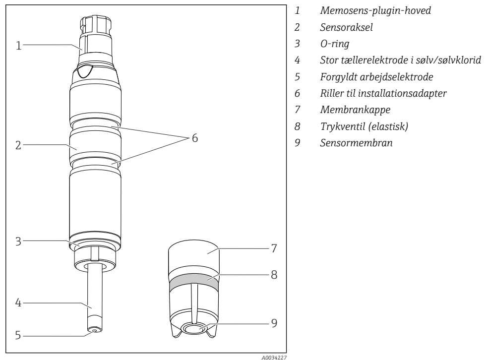
1 Sensorens opbygning
