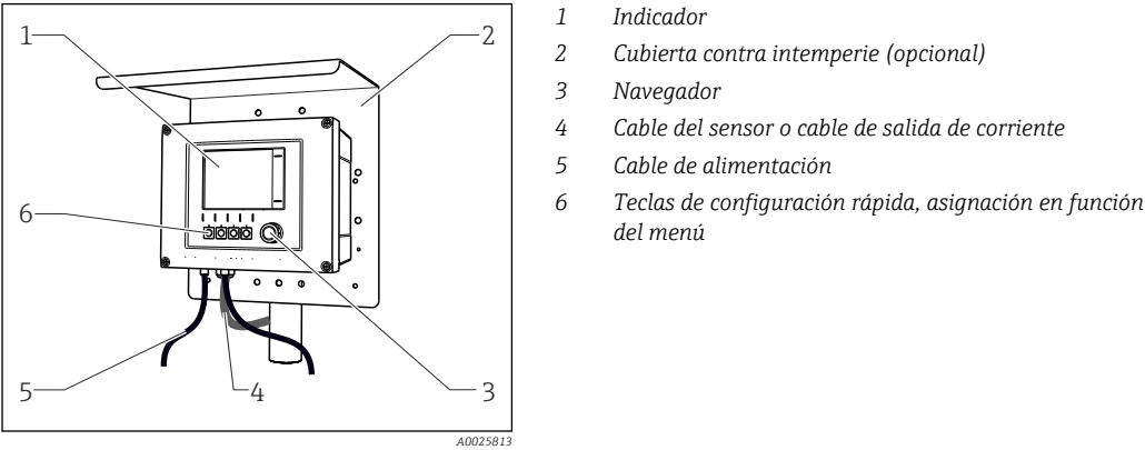
1 Montaje en barra de soporte
