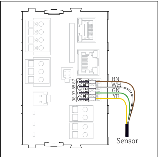
43 Memosens sensores sin fuente de alimentación adicional
