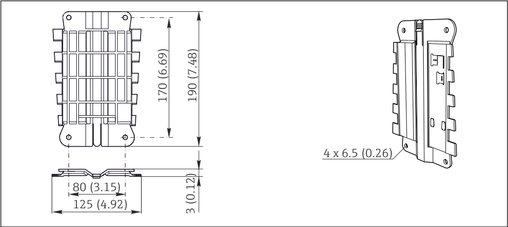
9 Placa de montaje. Unidad física: mm (in)
