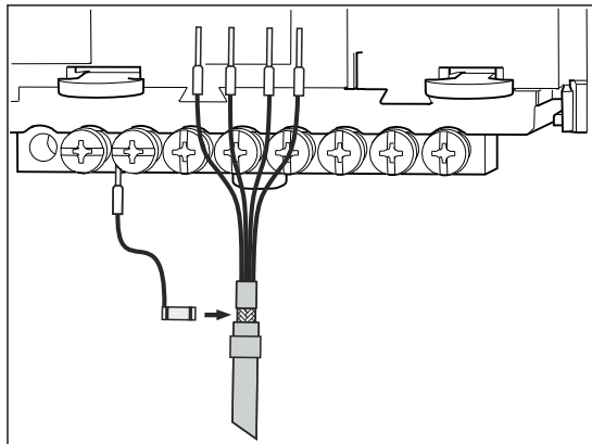
42 Conexión de tierra funcional
