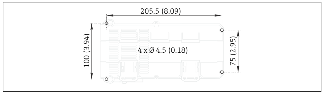
13 Esquema de taladros para montaje en pared en mm (pulgadas)
