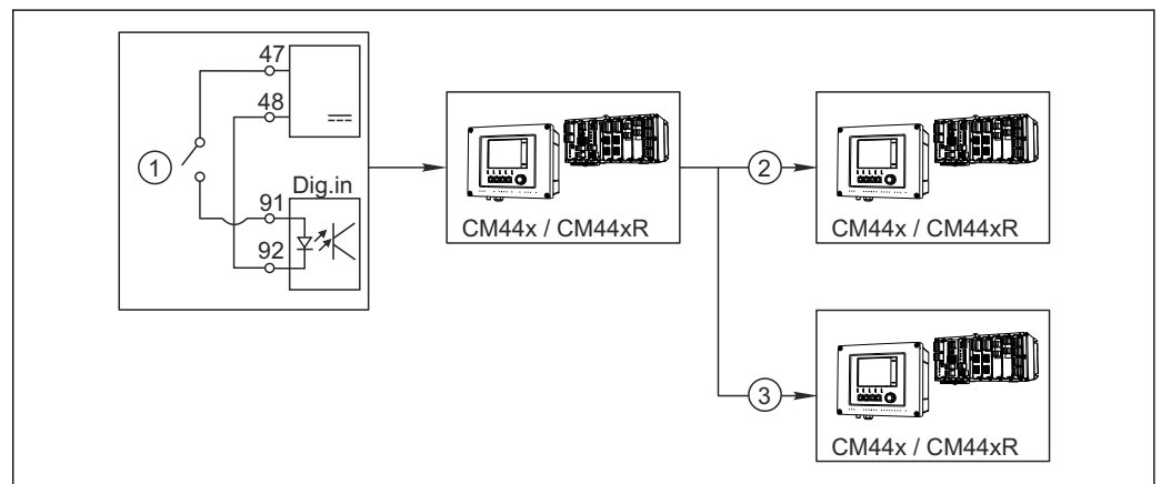
88 Ejemplo de un control de limpieza central
