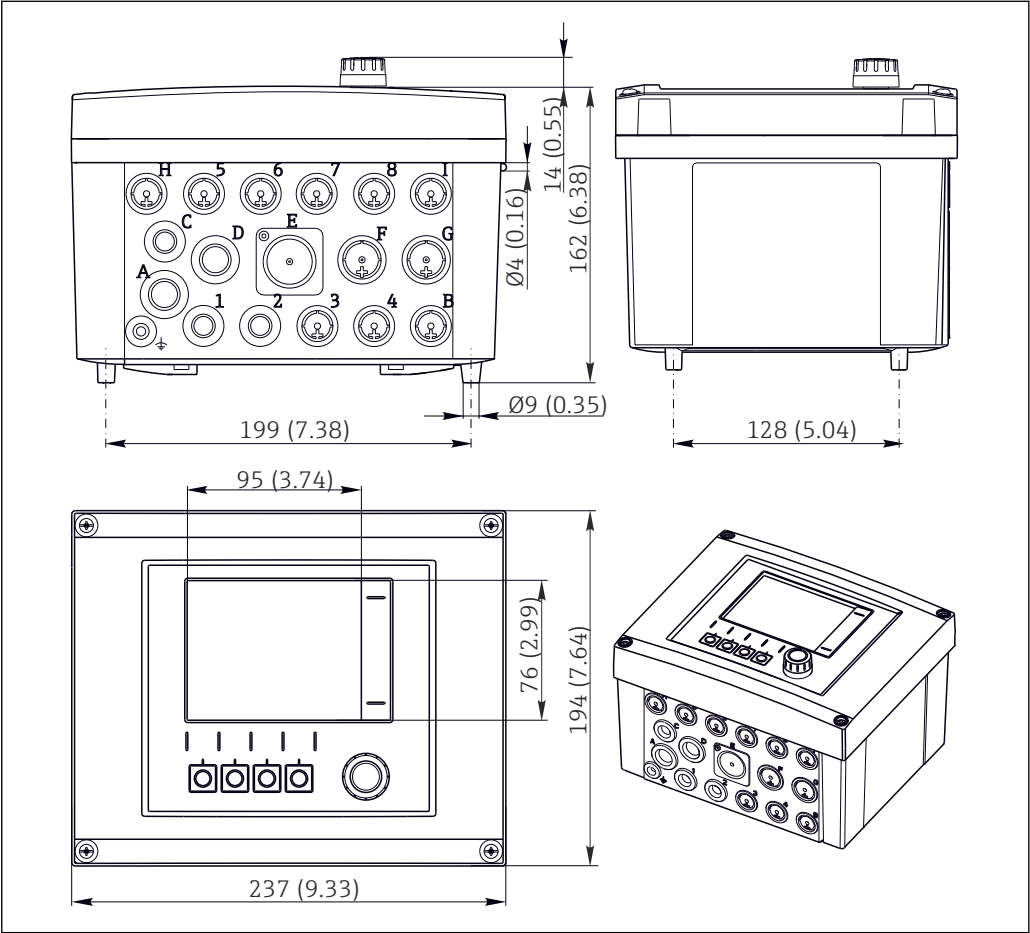
8 Medidas de la caja para montaje en campo en mm (in)
