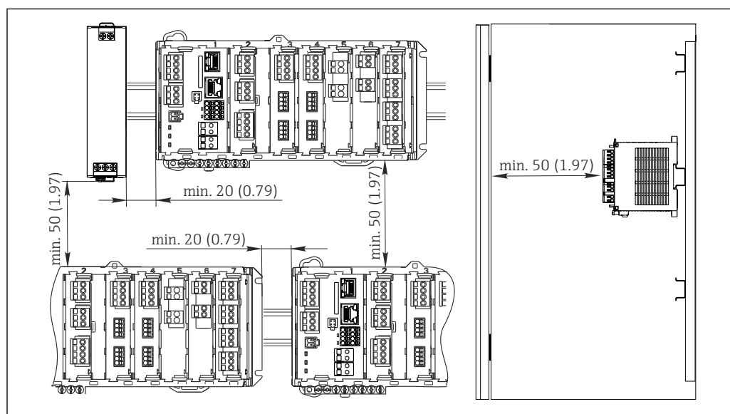
12 Espacio mínimo en mm (pulgadas)
