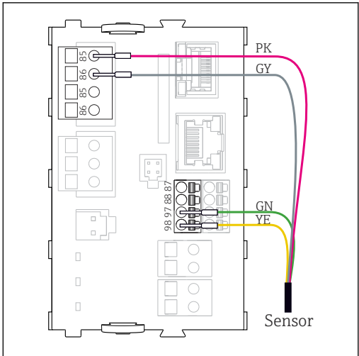
44 Memosens sensores con fuente de alimentación adicional
