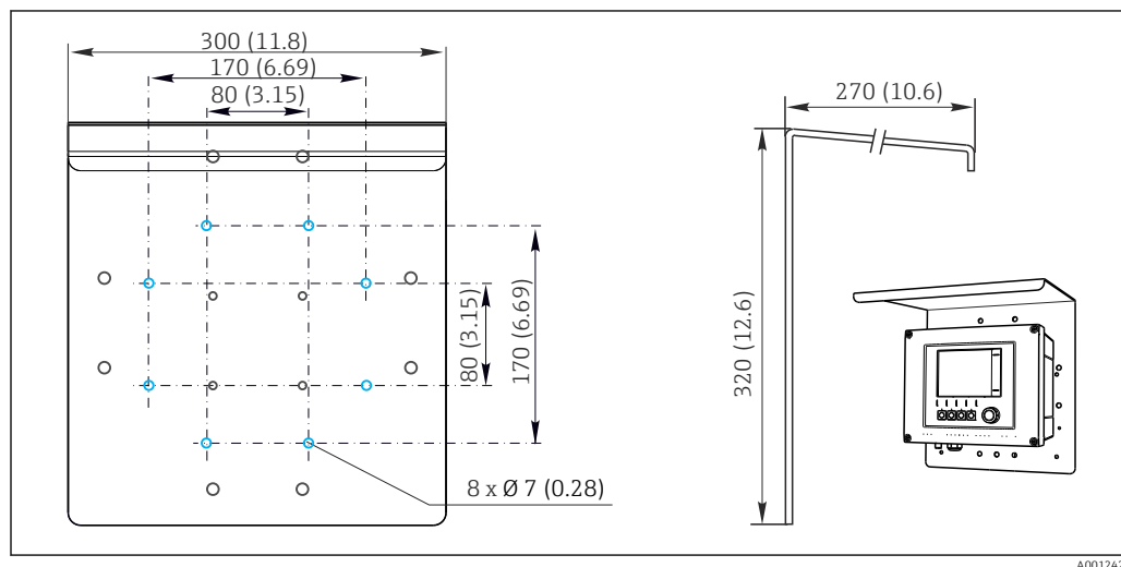
10 Dimensiones en mm (in)
