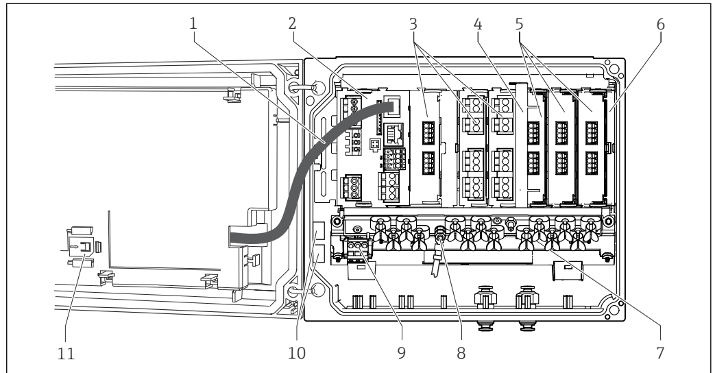
3 Ejemplo de un equipo de campo con módulo de comunicación del sensor de tipo 2DS Ex-i y cubierta del indicador abierta (sin cableado)
