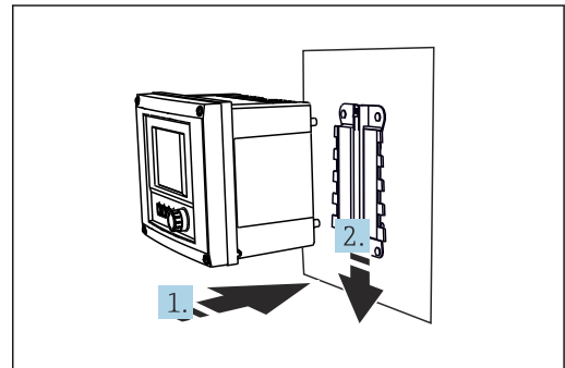
24 Sujete bien el equipo en el lugar deseado y fíjelo hasta oír el clic
