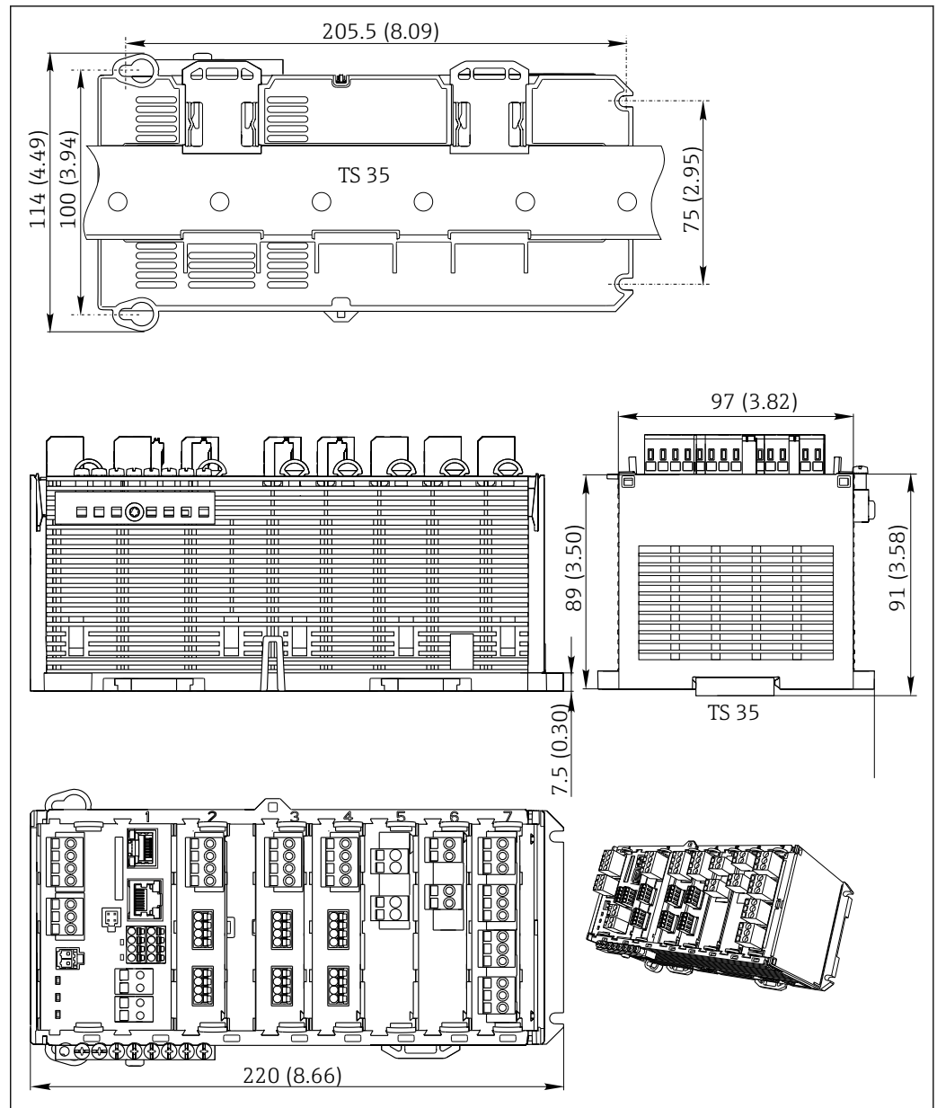
11 Dimensiones en mm (pulgadas)
