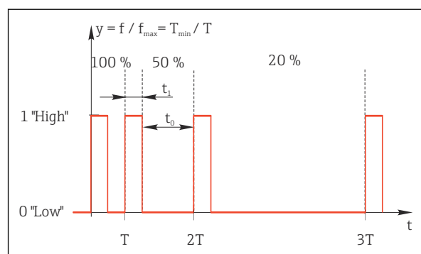
86 Aplicación típica: bomba dosificadora
