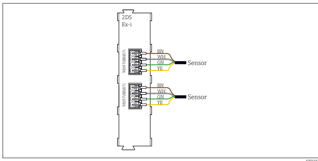
49 Sensores sin tensión de alimentación adicional en el módulo de comunicación del sensor de tipo 2DS Ex-i
