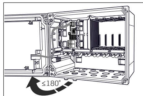
31 Abra la tapa que cubre la pantalla, ángulo máx. de apertura 180° (depende del lugar de montaje)
