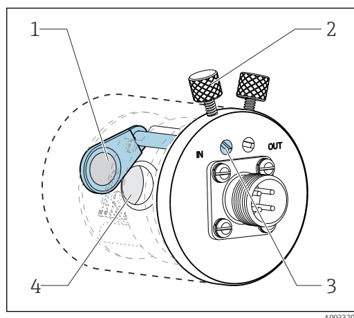
98 Filtro en posición "fuera"
