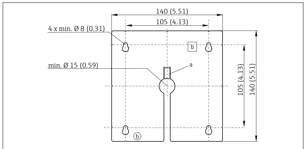
14 Placa de montaje para el indicador externo, dimensiones en mm (pulgadas)
