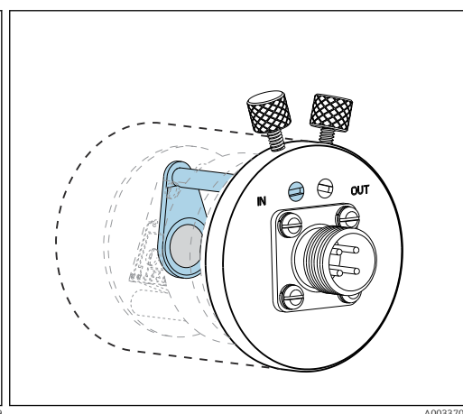
99 Filtro en posición "dentro"
