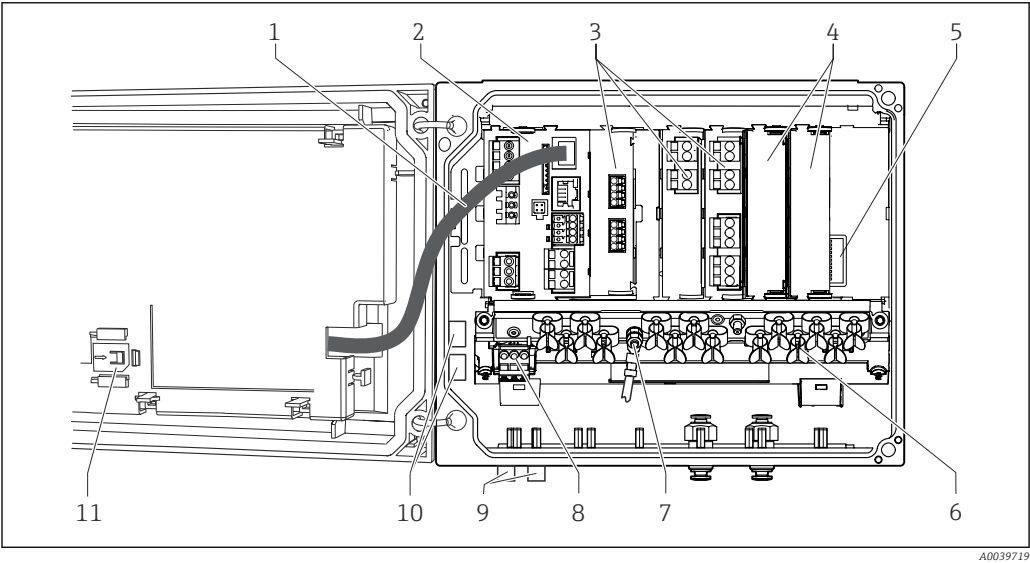
2 Ejemplo de un equipo de cuatro canales con tapa del indicador abierta (sin cableado)
