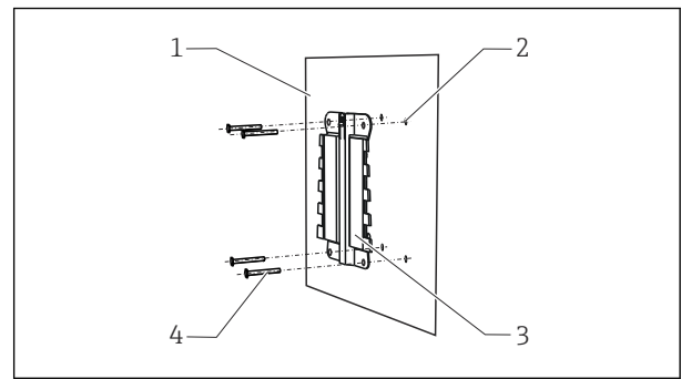
22 Montaje en pared
