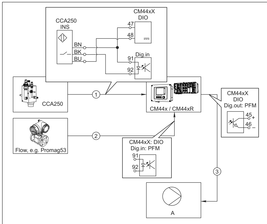
87 Ejemplo de control de cloro con control preventivo
