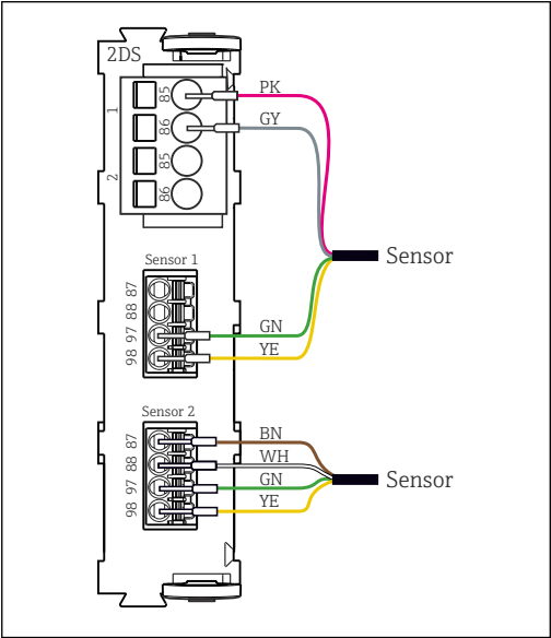
45 Sensores con y sin tensión de alimentación adicional en el módulo del sensor 2DS
