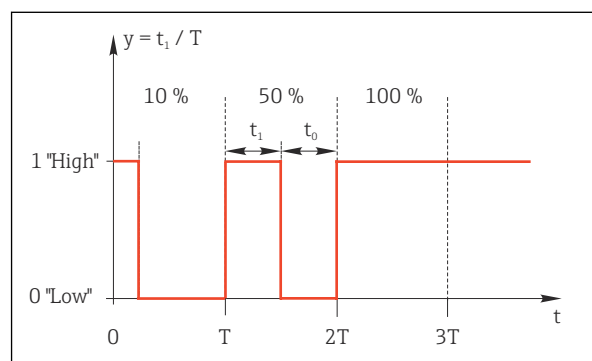
85 Aplicaciones típicas: válvula solenoide
