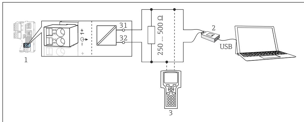
29 Mediante módem HART
