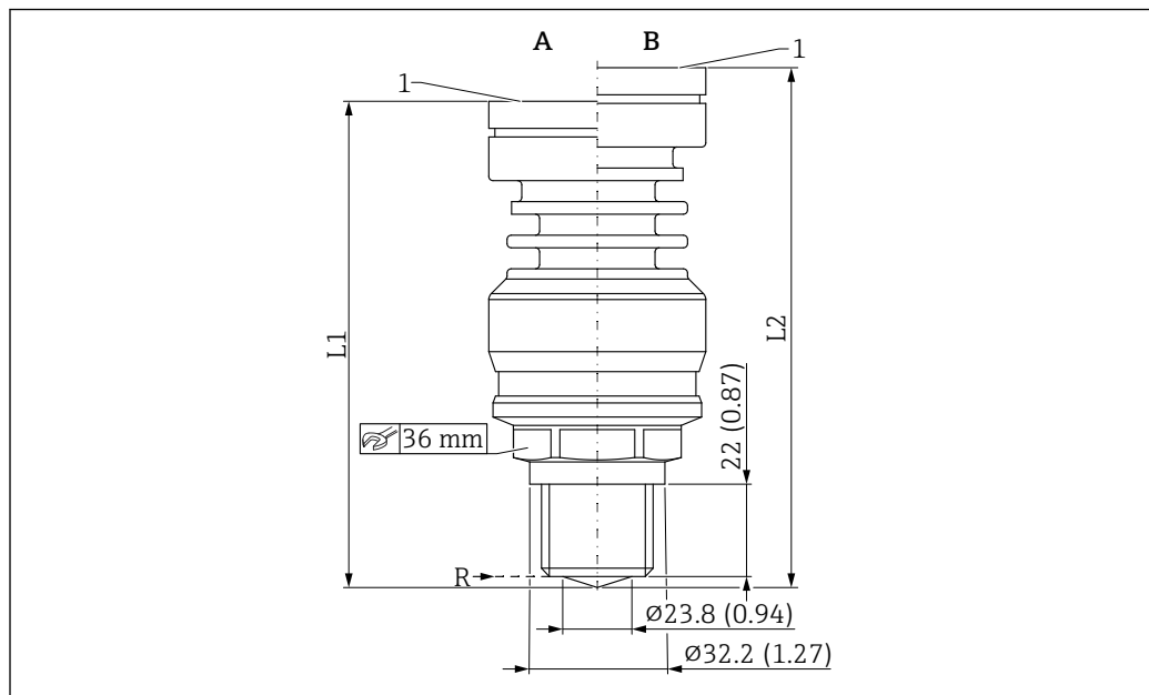
55 Dimensions ; antenne intégrée, PEEK, 20 mm (0,75 in) ; raccord process, filetage 3/4". Unité de mesure mm (in)
