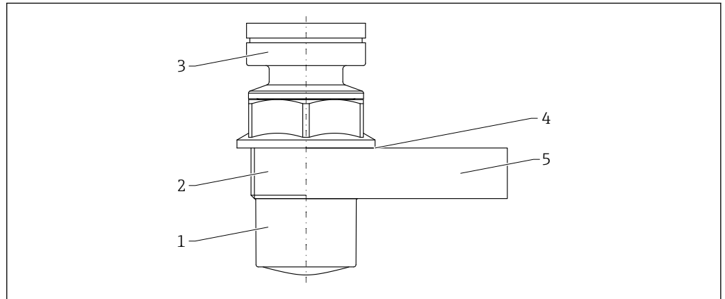
■ 57 Matériau ; antenne encapsulée, PVDF, 40 mm (1,5 in)
