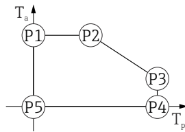
11 Boîtier plastique ; température de process 0 \dots +150 \text{ }^{\circ}\text{C} ( +32 \dots +302 \text{ }^{\circ}\text{F} ) avec agrément CSA C/US
