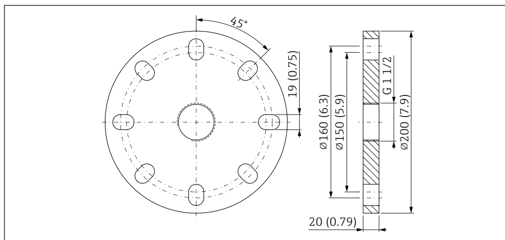
47 Dimensions de la bride UNI 3"/DN80/80A. Unité de mesure mm (in)
