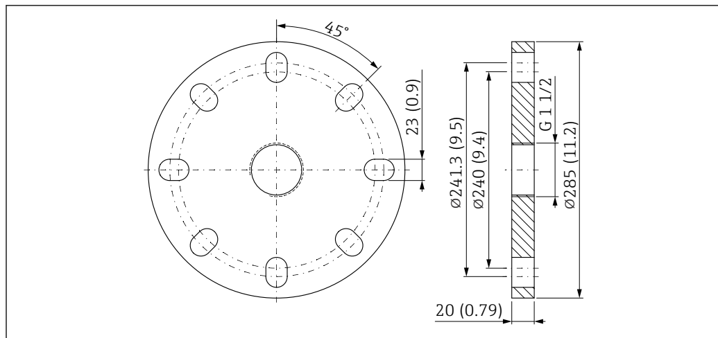
54 Dimensions de la bride UNI 6"/DN150/150A. Unité de mesure mm (in)
