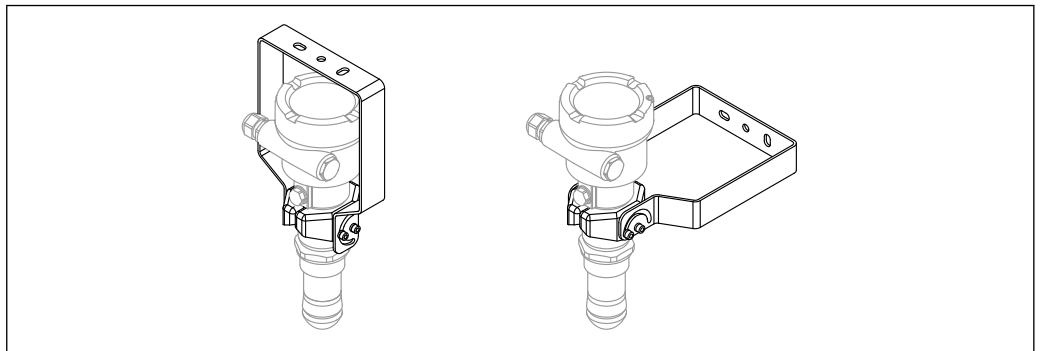
65 Montage sur toit ou paroi
