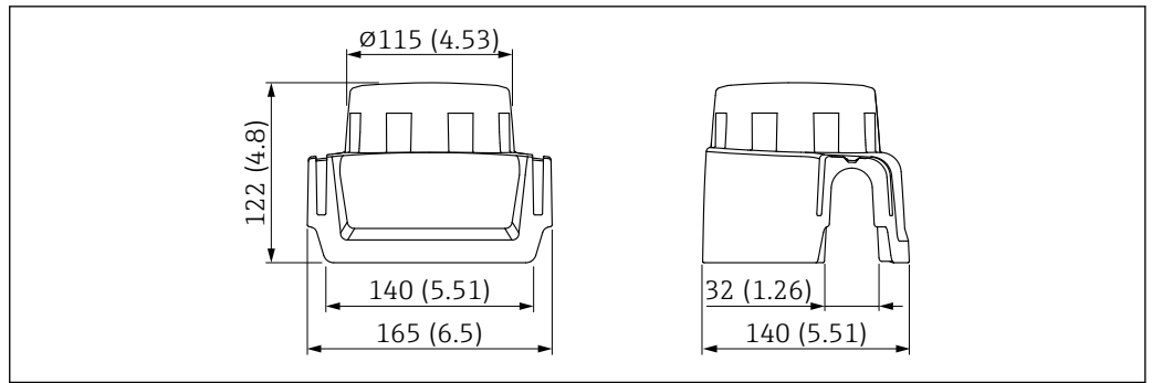
64 Dimensions. Unité de mesure mm (in)
