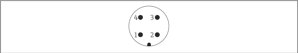
7 Vue du connecteur enfichable de l'appareil 1 Signal + 2 Non utilisée 3 Signal - 4 Masse
