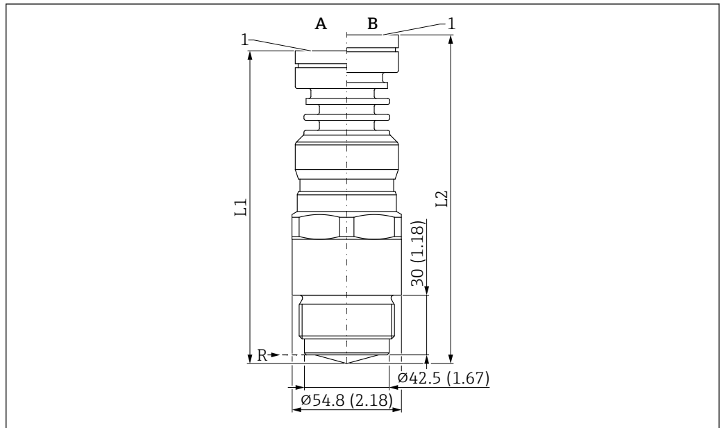
56 Dimensions ; antenne intégrée, PEEK, 40 mm (1,5 in) ; raccord process, filetage 1-1/2". Unité de mesure mm (in)
