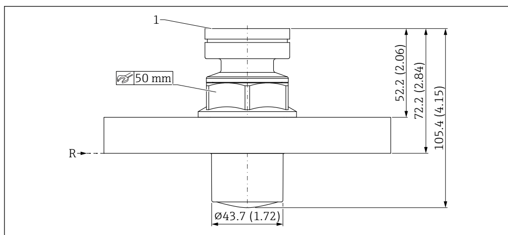
46 Dimensions de l'antenne encapsulée, PVDF, 40 mm (1,5 in), raccord process bride UNI. Unité de mesure mm (in)
