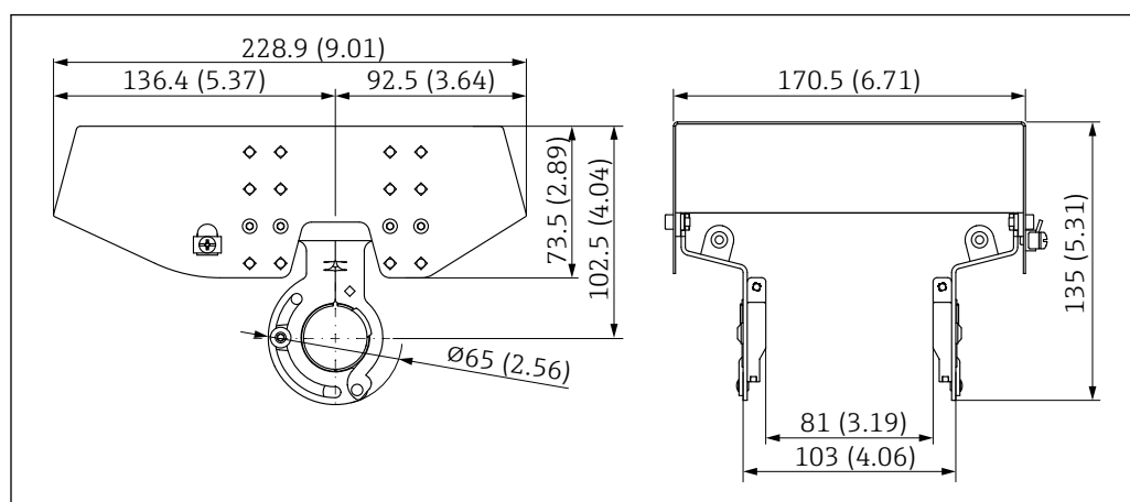
63 Dimensions. Unité de mesure mm (in)
