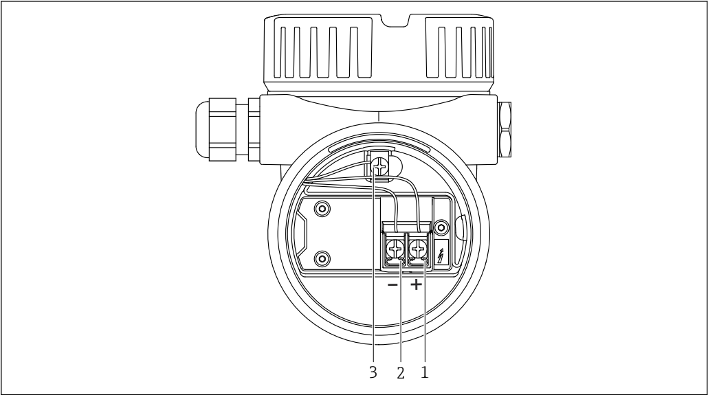
6 Bornes de raccordement et borne de terre dans le compartiment de raccordement 1 Borne plus 2 Borne moins 3 Borne de terre interne
