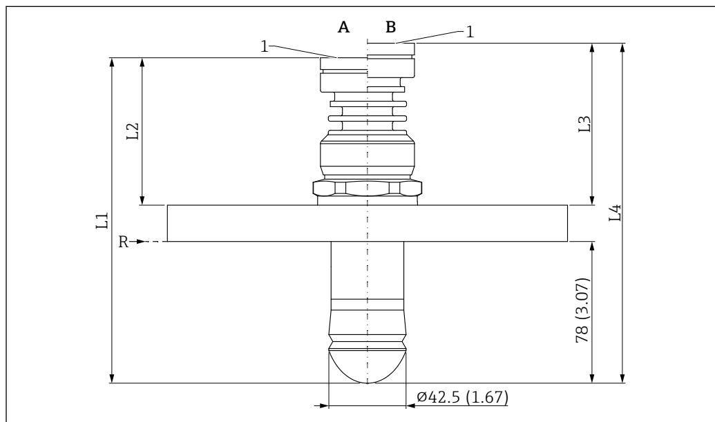
51 Dimensions de l'antenne drip-off 50 mm (2 in), bride UNI raccord process. Unité de mesure mm (in)
