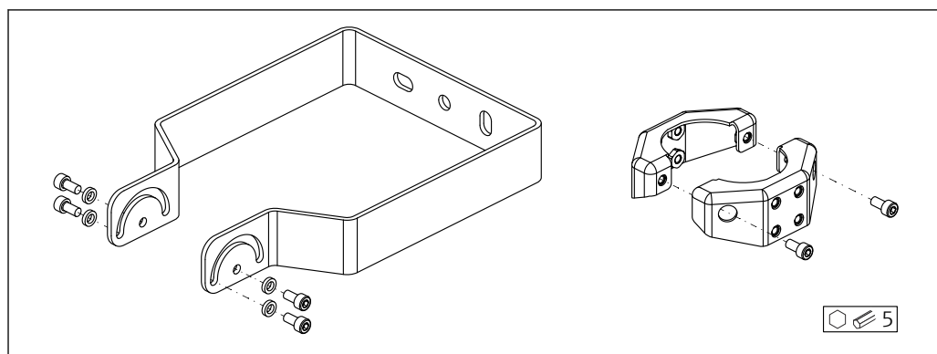
67 Contenu de la livraison de l'étrier de montage, réglable
