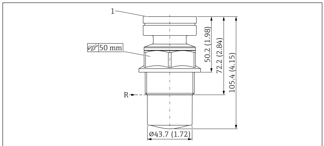
45 Dimensions de l'antenne encapsulée, PVDF, 40 mm (1,5 in). Unité de mesure mm (in)
