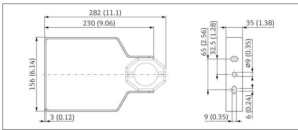
66 Dimensions de l'étrier de montage. Unité de mesure mm (in)
