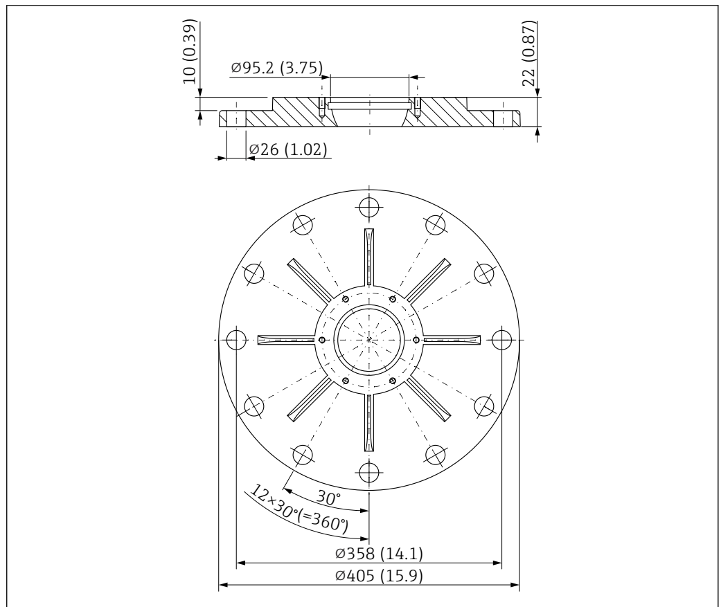
58 Dimensions de la bride UNI 10"/DN250/250A pour antennes avec dispositif d'orientation. Unité de mesure mm (in)
