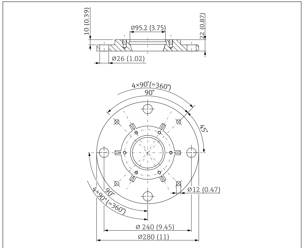
43 Dimensions de la bride UNI 6"/DN150/150A pour antennes avec dispositif d'orientation. Unité de mesure mm (in)
