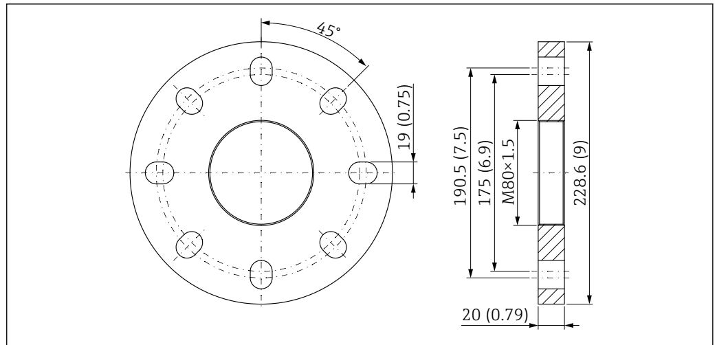
48 Bride UNI 4"/DN100/100A pour antenne drip-off, PTFE, 50 mm (2 in) avec raccord d'air de purge. Unité de mesure mm (in)
