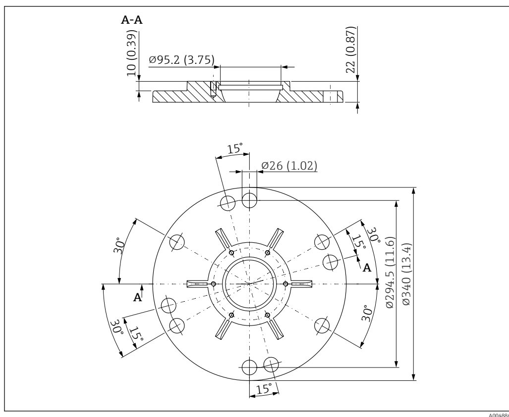
57 Dimensions de la bride UNI 8"/DN200/200A pour antennes avec dispositif d'orientation. Unité de mesure mm (in)
