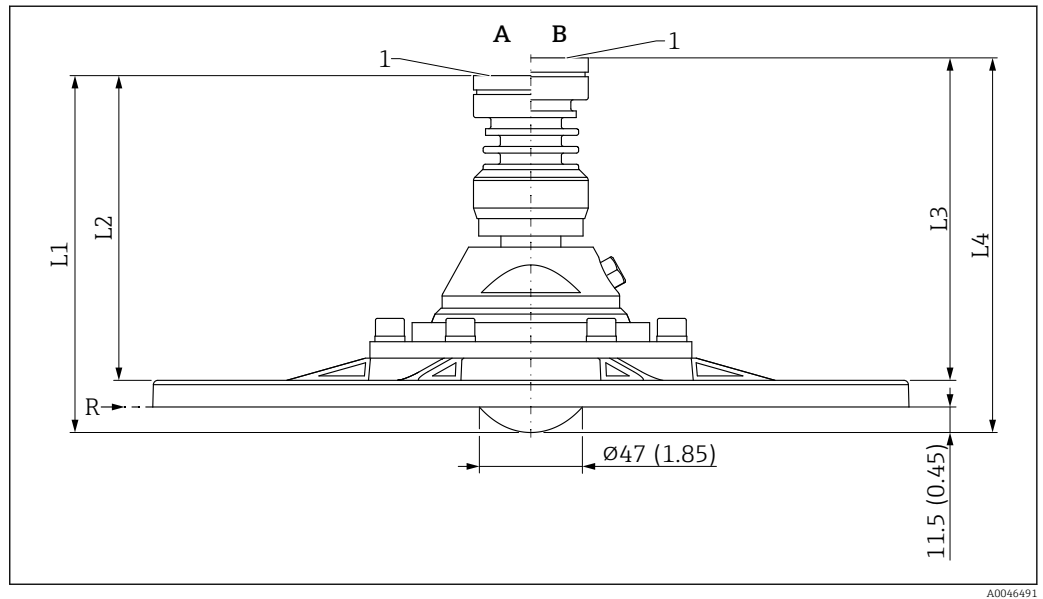
54 Dimensions de l'antenne affleurante, 80 mm (3 in), avec bride UNI, dispositif d'orientation et raccord d'air de purge. Unité de mesure mm (in)
