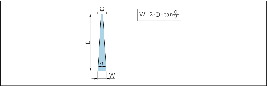
11 Relation entre l'angle d'émission \alpha , la distance D et la largeur de faisceau W
