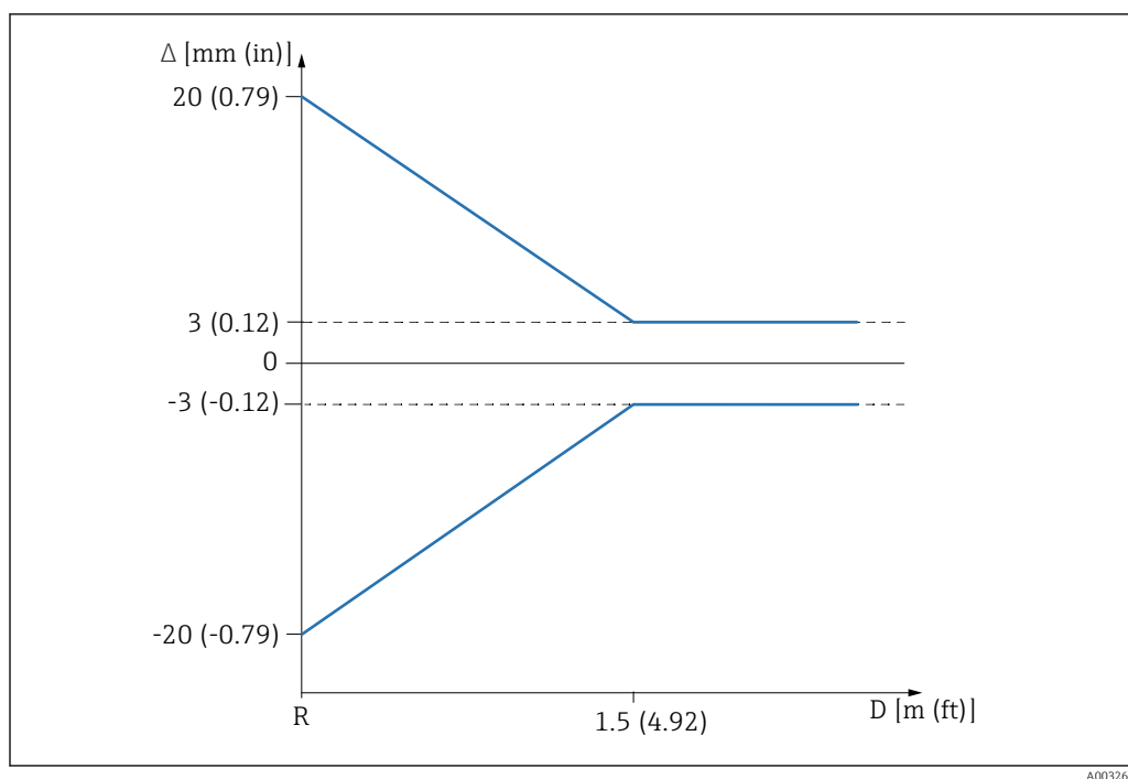
7 Écart de mesure maximal dans la portée proximale
