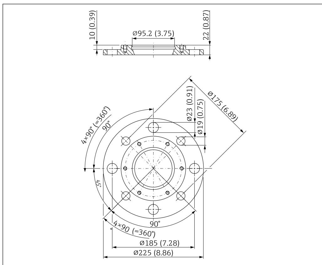
42 Dimensions de la bride UNI 4"/DN100/100A pour antennes avec dispositif d'orientation. Unité de mesure mm (in)
