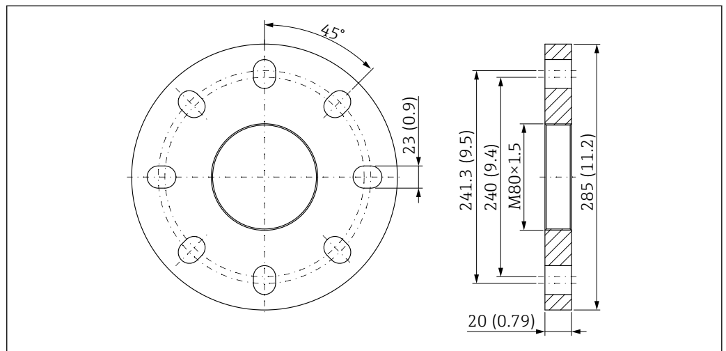
49 Bride UNI 6"/DN150/150A pour antenne drip-off, PTFE, 50 mm (2 in) avec raccord d'air de purge. Unité de mesure mm (in)
