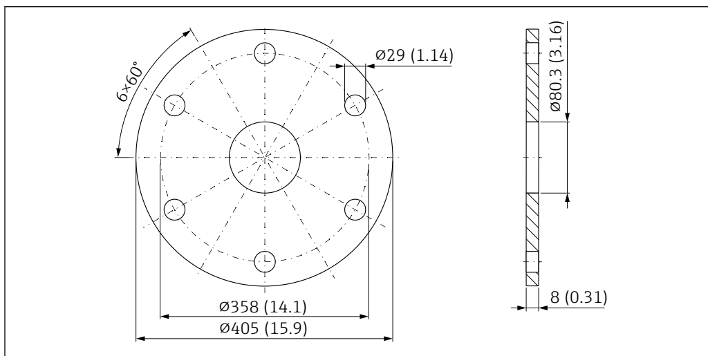
53 Dimensions de la bride UNI 10"/DN250/250A pour antenne DN80 avec raccord d'air de purge. Unité de mesure mm (in)
