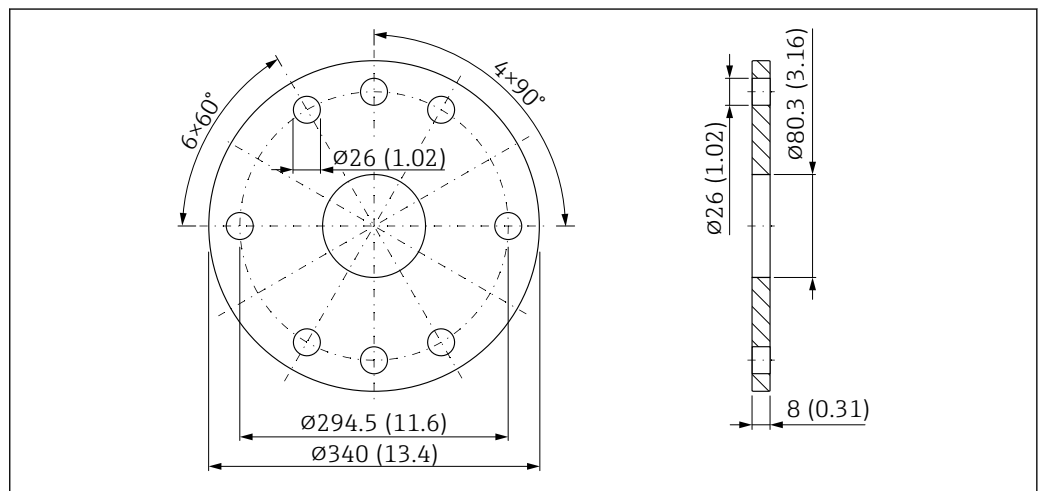
52 Dimensions de la bride UNI 8"/DN200/200A pour antenne DN80 avec raccord d'air de purge. Unité de mesure mm (in)
