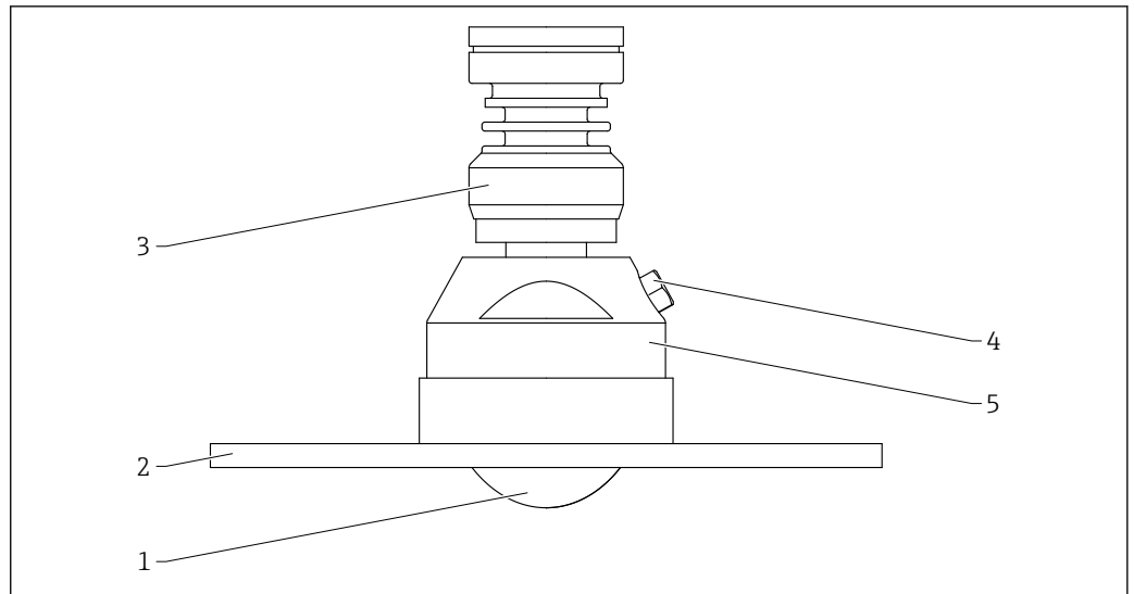
63 Matériau ; antenne affleurante, 80 mm (3 in), avec bride UNI et raccord d'air de purge. Unité de mesure mm (in)
