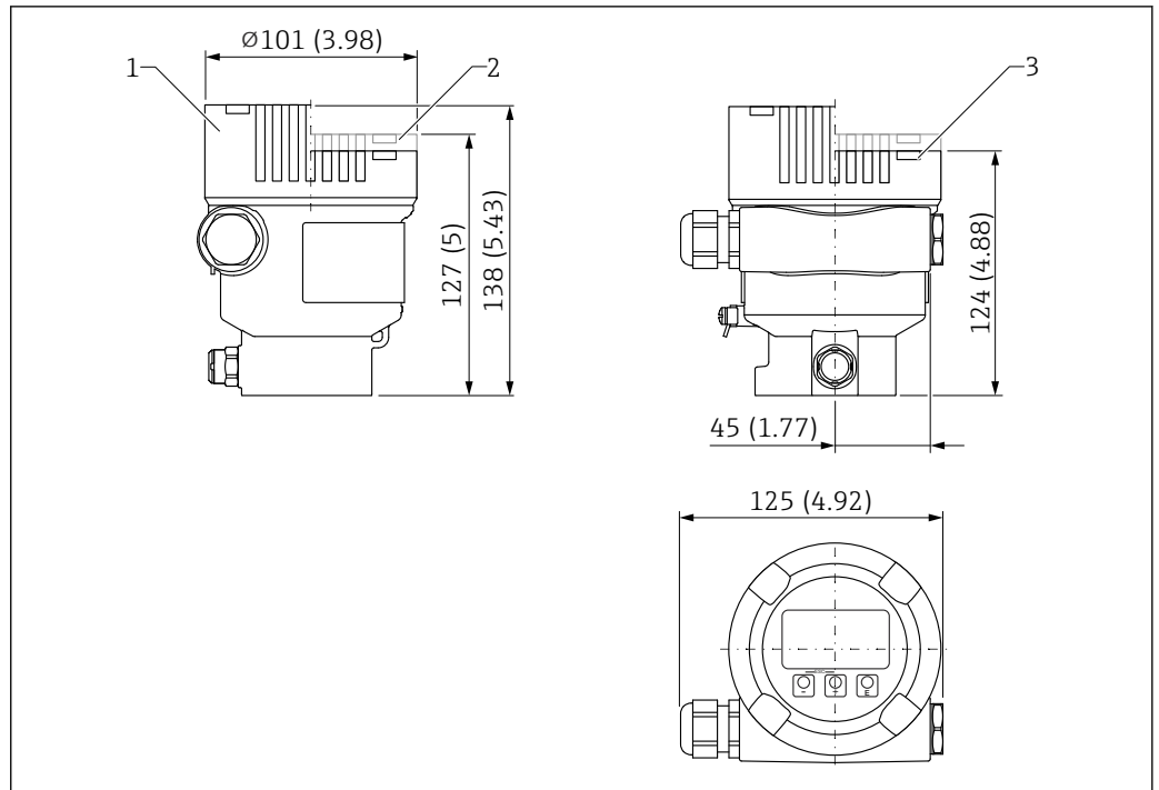
36 Dimensions du boîtier à simple compartiment en aluminium. Unité de mesure mm (in)
