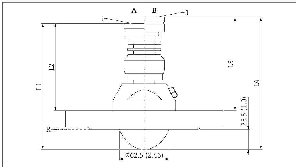
50 Dimensions de l'antenne affleurante, PTFE, 80 mm (3 in), avec bride standard et raccord d'air de purge . Unité de mesure mm (in)
