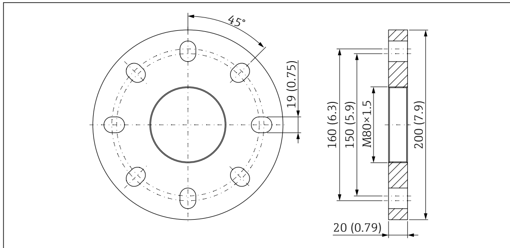
47 Bride UNI 3"/DN80/80A pour antenne drip-off, PTFE, 50 mm (2 in) avec raccord d'air de purge. Unité de mesure mm (in)
