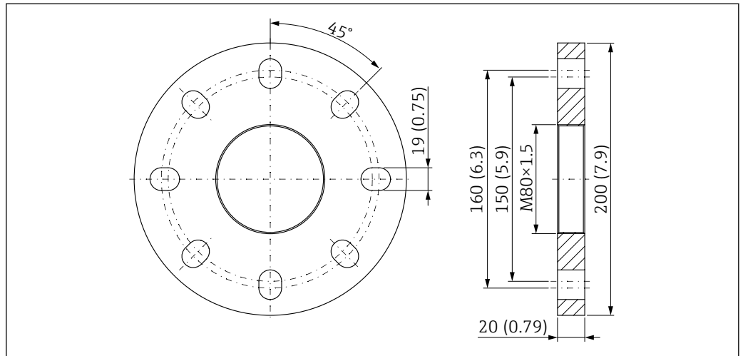
47 Brida UNI 3" / DN 80 / 80 A para antena de goteo, PTFE, 50 mm (2 in) con conexión de aire de purga. Unidad de medida mm (in)
