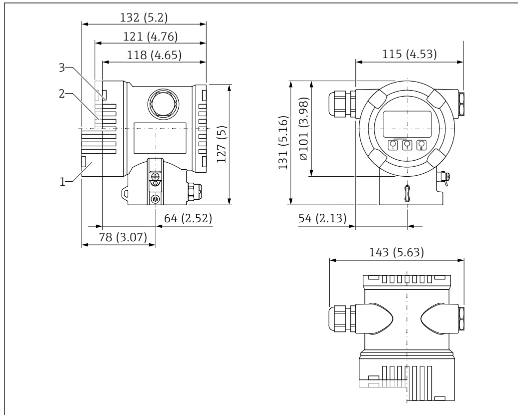
38 Medidas de la caja de compartimento doble. Unidad de medida mm (in)
