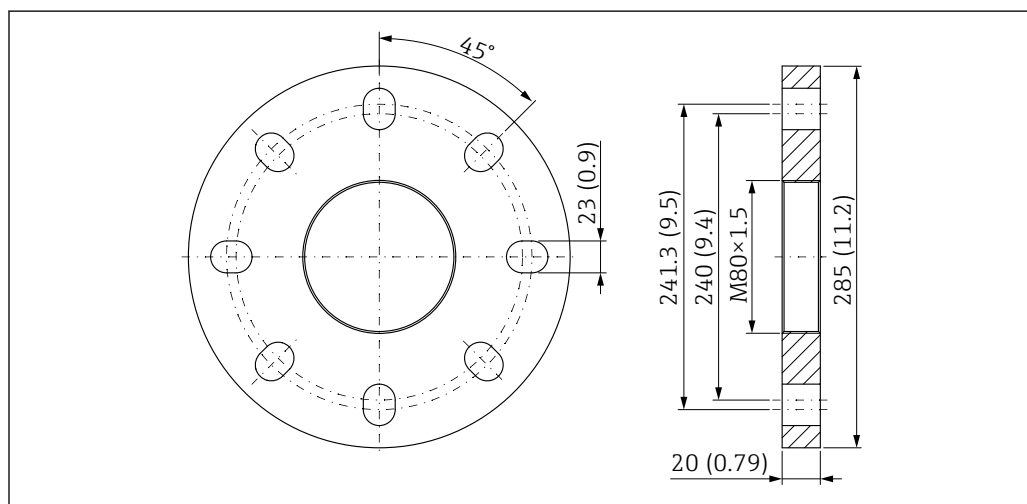
■ 49 UNI brida 6" / DN 150 / 150 A para antena de goteo, PTFE, 50 mm (2 in) con conexión de aire de purga. Unidad de medida mm (in)
