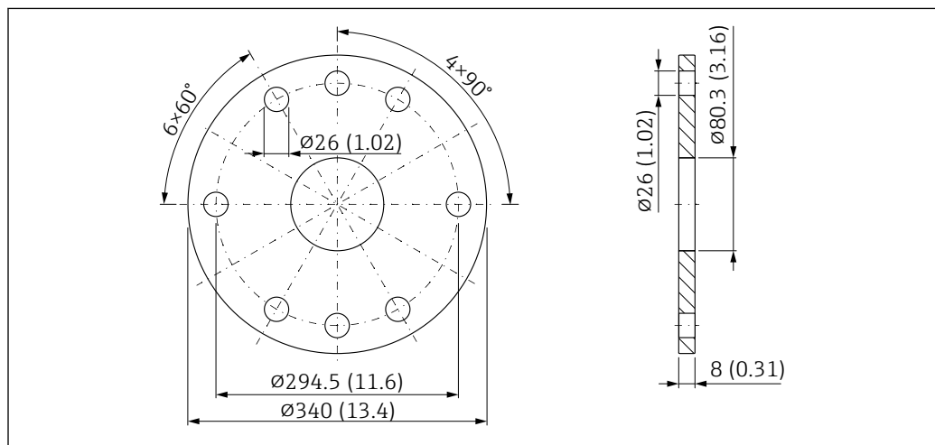
52 Medidas de la brida UNI 8" / DN 200 / 200 A para antenas DN 80 con conexión de aire de purga. Unidad de medida mm (in)
