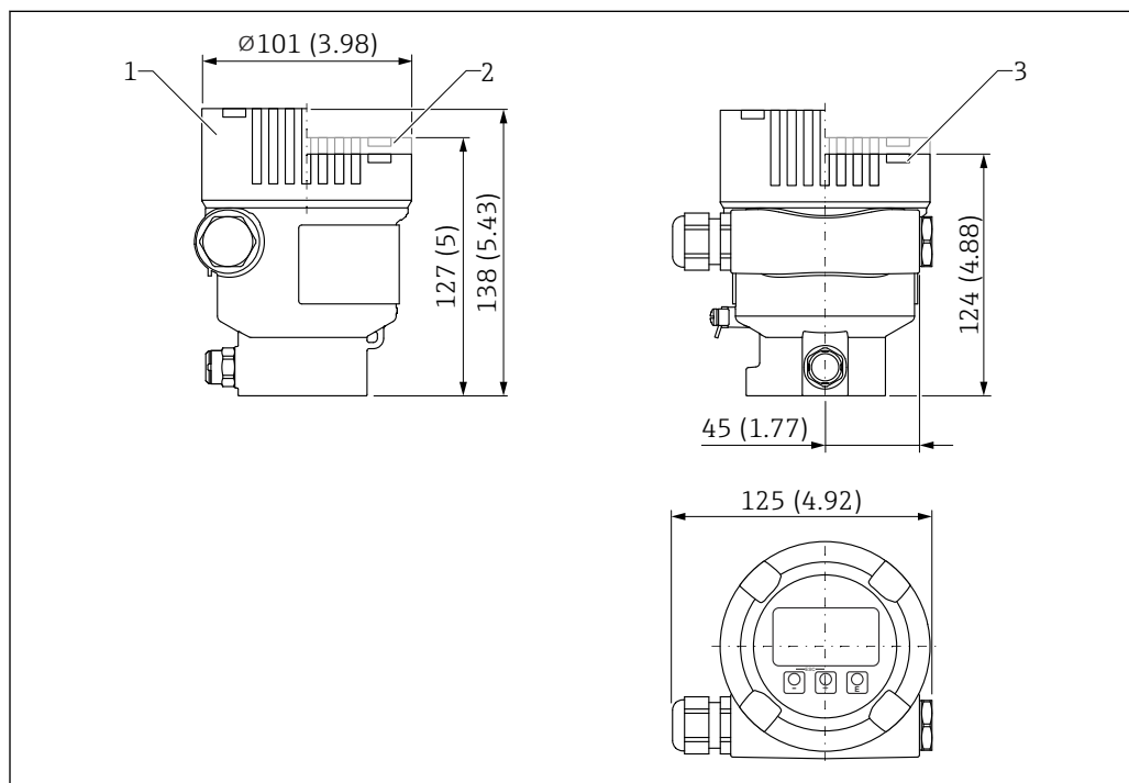
36 Medidas de la caja de aluminio de compartimento único. Unidad de medida mm (in)
