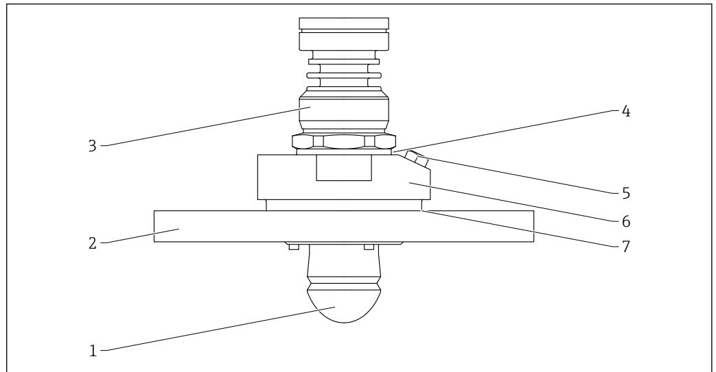
61 Material; antena de goteo, conexión de aire de purga . Unidad de medida mm (in)
