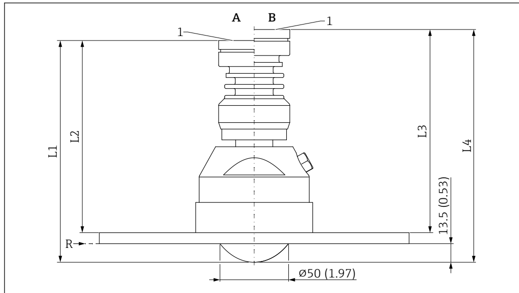
51 Medidas de la antena de montaje enrasado, PTFE, 80 mm (3 in), con brida UNI y conexión de aire de purga. Unidad de medida mm (in)
