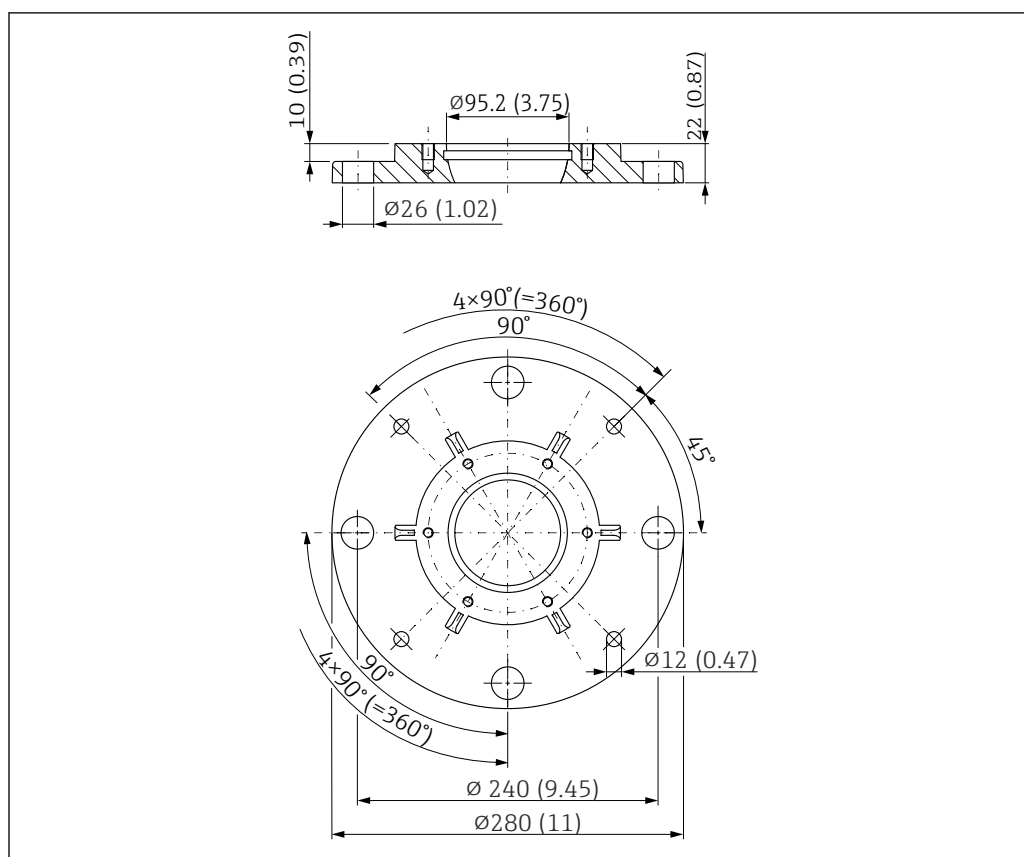
56 Medidas de la brida UNI 6" / DN 150 / 150 A para antenas con unidad de alineación. Unidad de medida mm (in)
