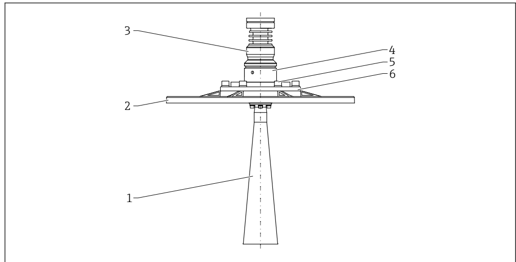
60 Material; antena de trompeta DN 65, con brida UNI y unidad de alineación. Unidad de medida mm (in)
