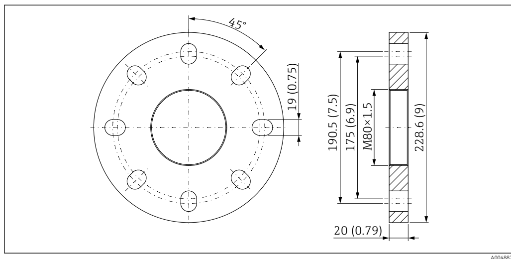
■ 48 Brida UNI 4" / DN 100 / 100 A para antena de goteo, PTFE, 50 mm (2 in) con conexión de aire de purga. Unidad de medida mm (in)
