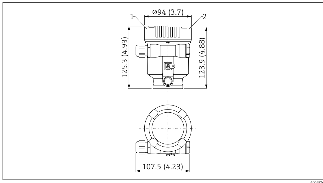
35 Medidas de la caja de compartimento único, plástico (PBT). Unidad de medida mm (in)
