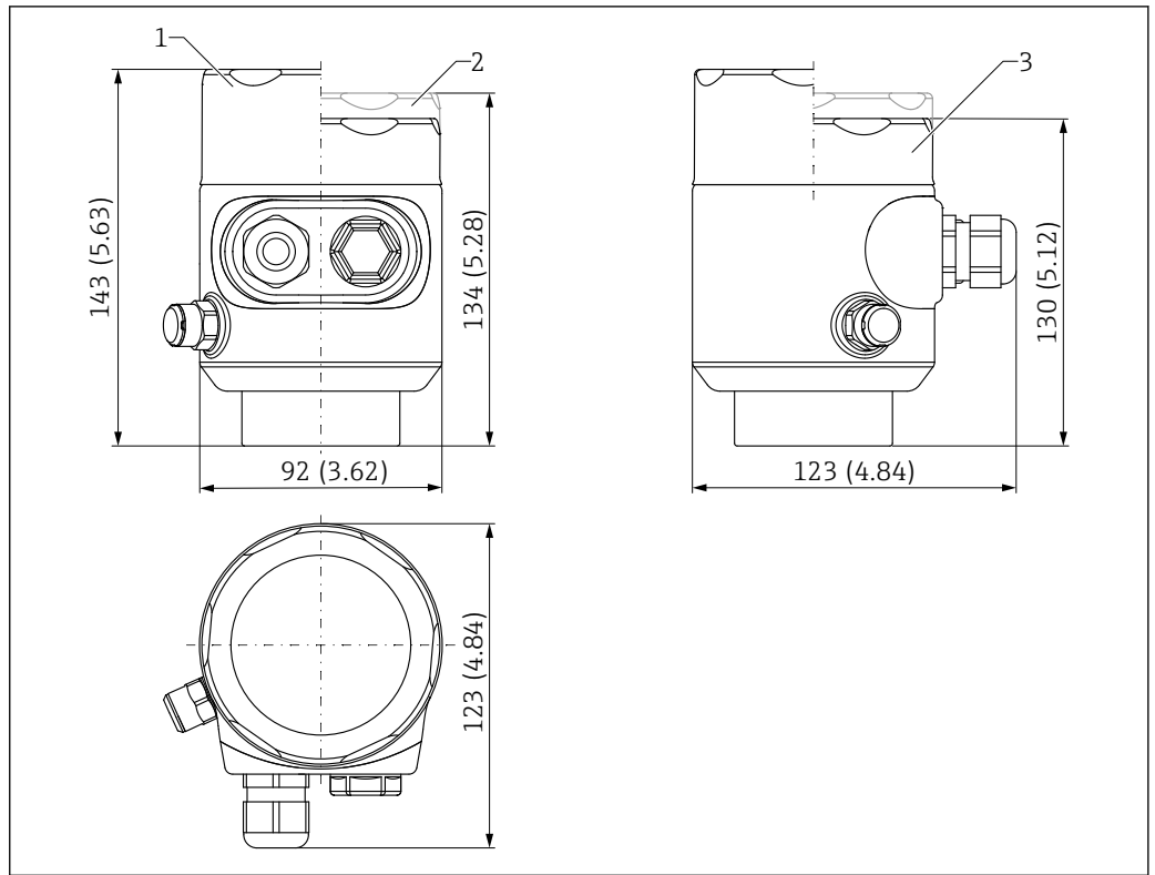
37 Medidas de la caja de compartimento único de 316L, higiene. Unidad de medida mm (in)
