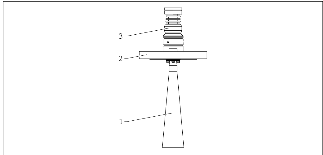
59 Material; antena de trompeta DN 65. Unidad de medida mm (in)
