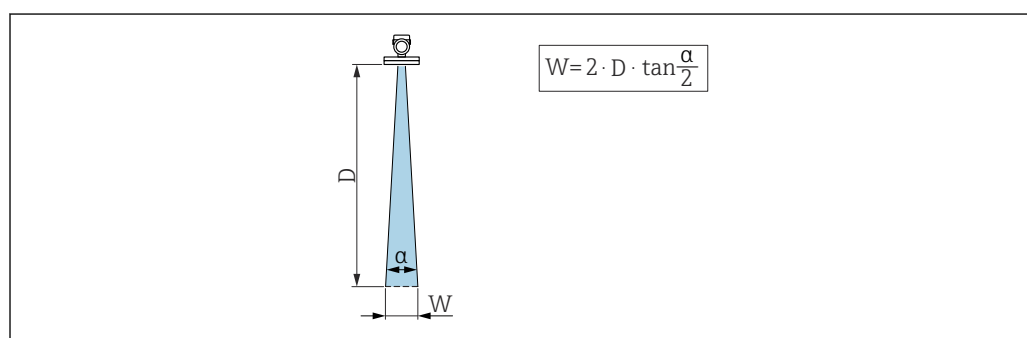
11 Relación entre el ángulo de abertura del haz \alpha , la distancia D y el diámetro del ancho del haz W
