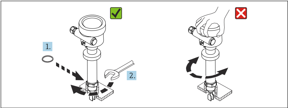
图 10 旋转拧入设备
