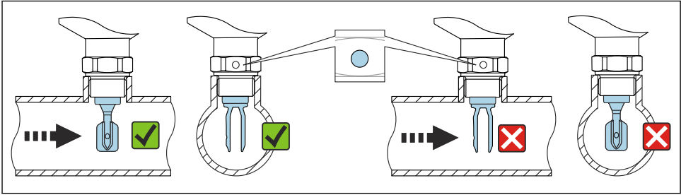
图 9 安装在管道中 (注意叉体安装位置和标记)
