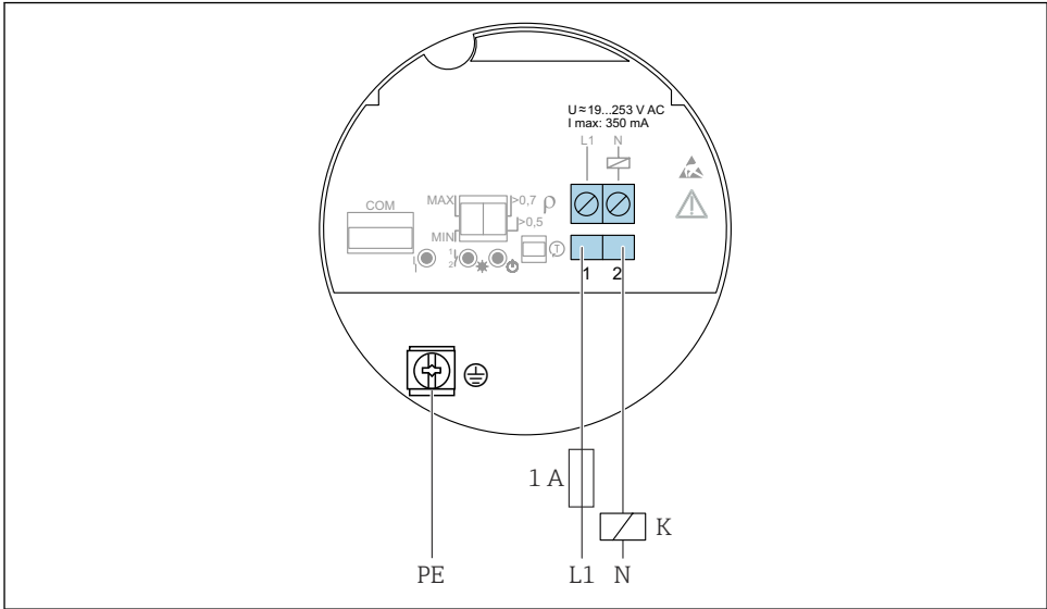
图 13 FEL61 电子插件：两线制连接，交流 AC 型
