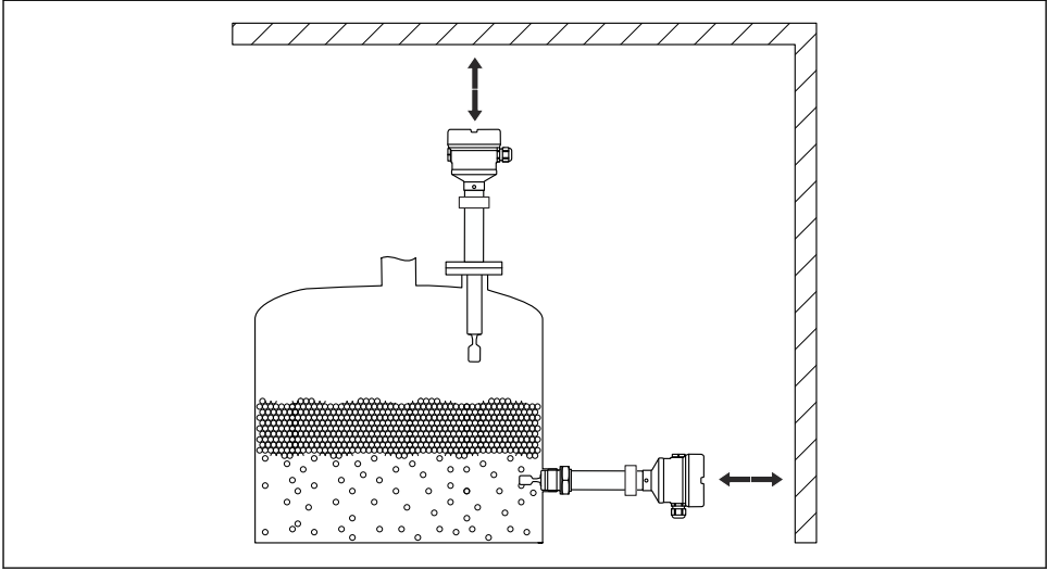
图 6 罐体外部预留安装间隙
