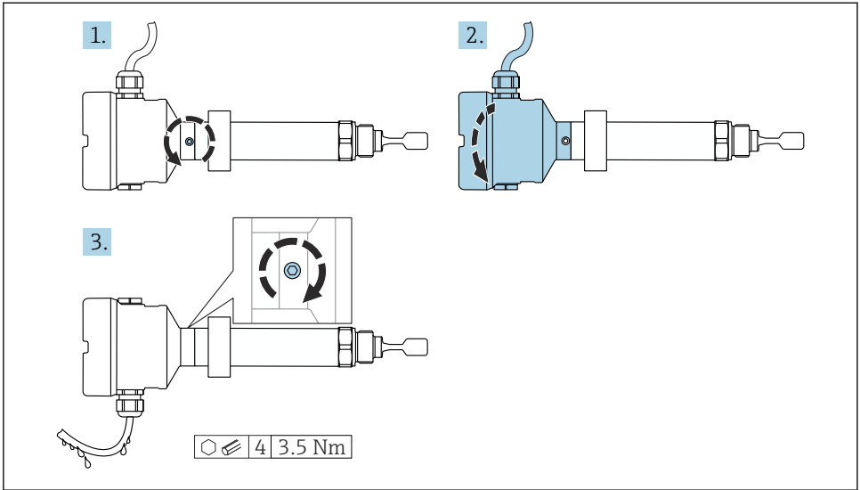
图 11 外壳带外部锁紧螺丝和排水回路
