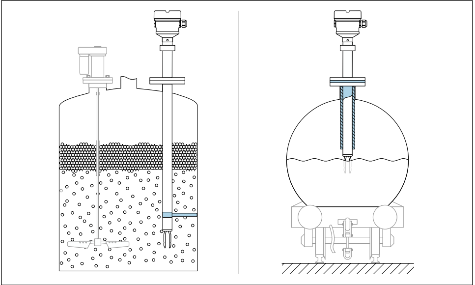
图 7 实例：存在动态负载时，应支撑设备
