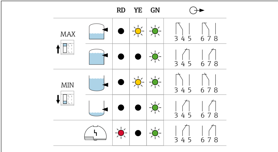
图 19 电子插件 FEL64 的继电器响应和故障信号
