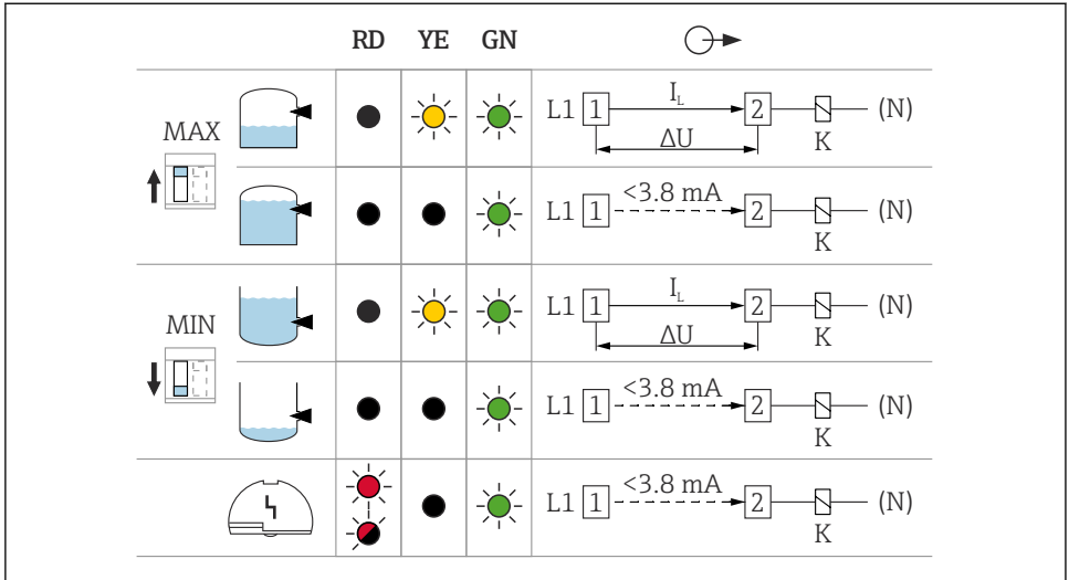
图 14 电子插件 FEL61 的继电器响应和故障信号
