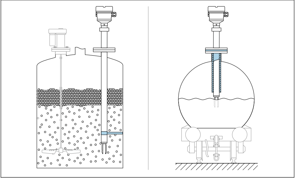
7 Dinamik yük durumunda destek örnekleri
