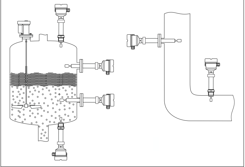
1 Bir kanal, tank veya boru için kurulum örnekleri
