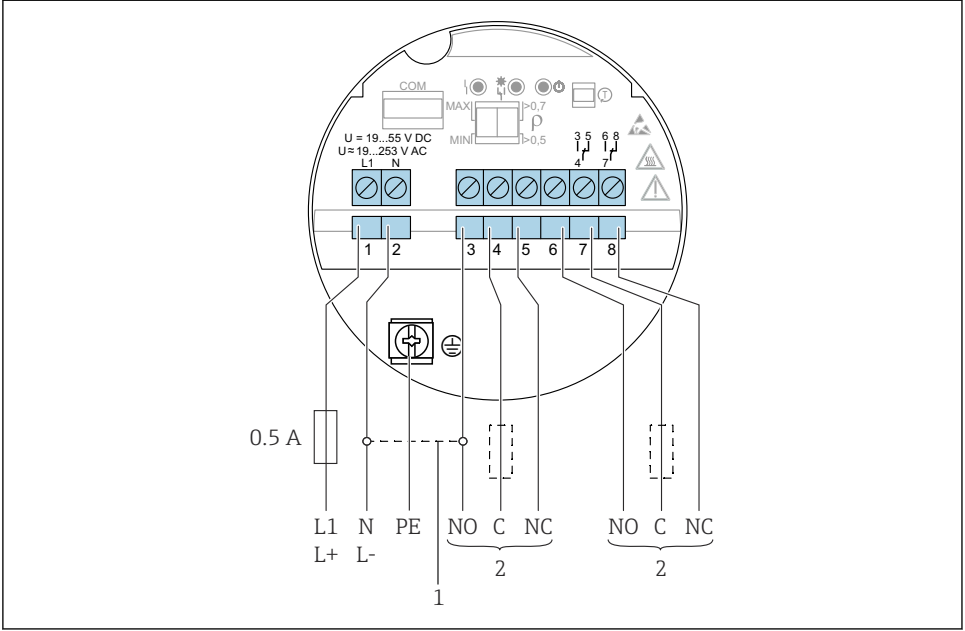
18 Röle çıkışlı universal akım bağlantısı, elektronik devre FEL64
