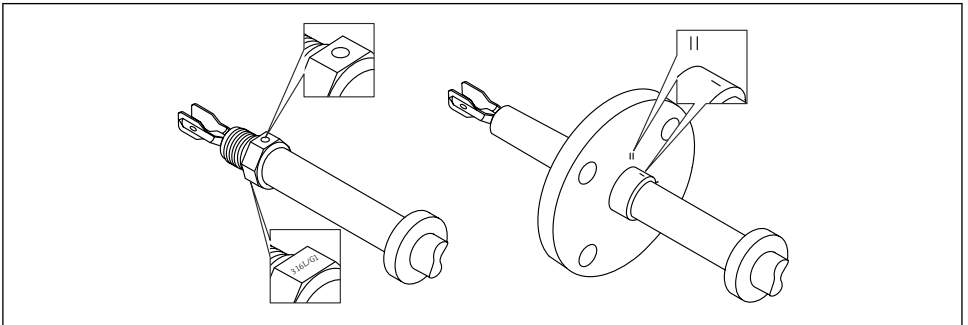
8 İşaretleme kullanılarak kanala yatay olarak monte edildiğinde ayar çatalının konumu
