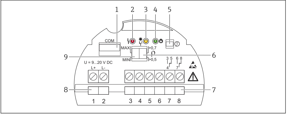
27 Örnek elektronik devre: FEL64DC
