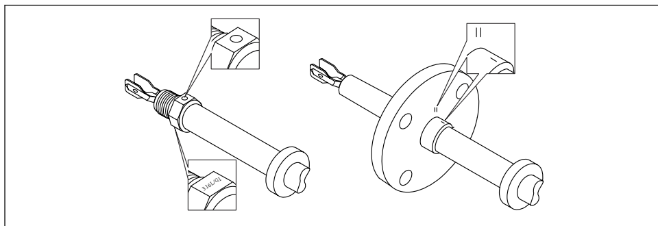
8 Positie van de trilvork bij horizontale installatie in de tank via de markering
