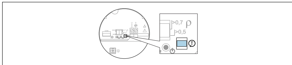
29 Positie van de toets voor de functietest voor elektronicamodules FEL61/62/64/64DC/67/68
